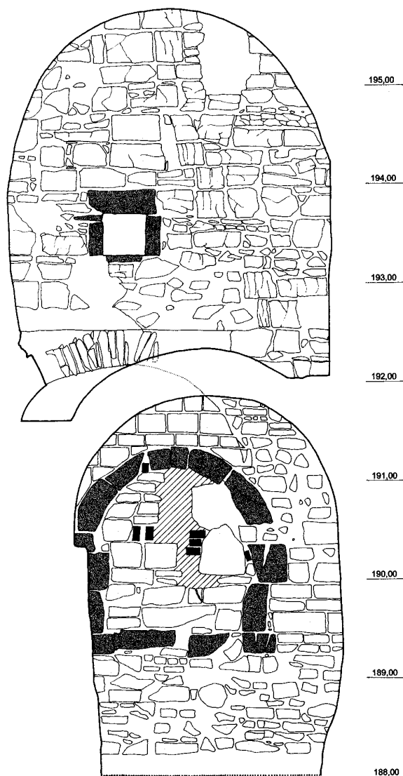
Obr. 5: Praha 1 - Staré Město, čp. 460/I. Pohled na jižní vnější stranu románského domu čp. 459/I s románským portálem, zbytkem klenby jeho zděné šíje a odkládací nikou v úrovni 2. podlaží. Nika a portál zvýrazněny. Pohled od jihu (kresba M. Semerád, L. Boháč a S. Matoušová).
