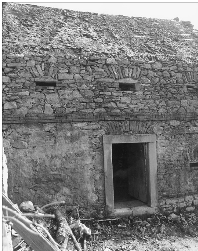
Obr. 3 : Pláň (okr. Plzeň - sever), sýpka usedlosti č. 5, pohled ze dvora. Současný stav s odhaleným hliněným lepenecem.
