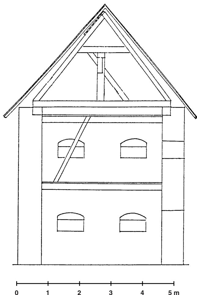
Obr. 4: Lestkov (okr. Tachov), sýpka usedlosti č. 84, příčný řez.
