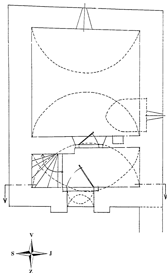
Obr. 9: Horní Jadruž (okr. Tachov), sýpka usedlosti č. 13, půdorys přízemí a příčný řez.
