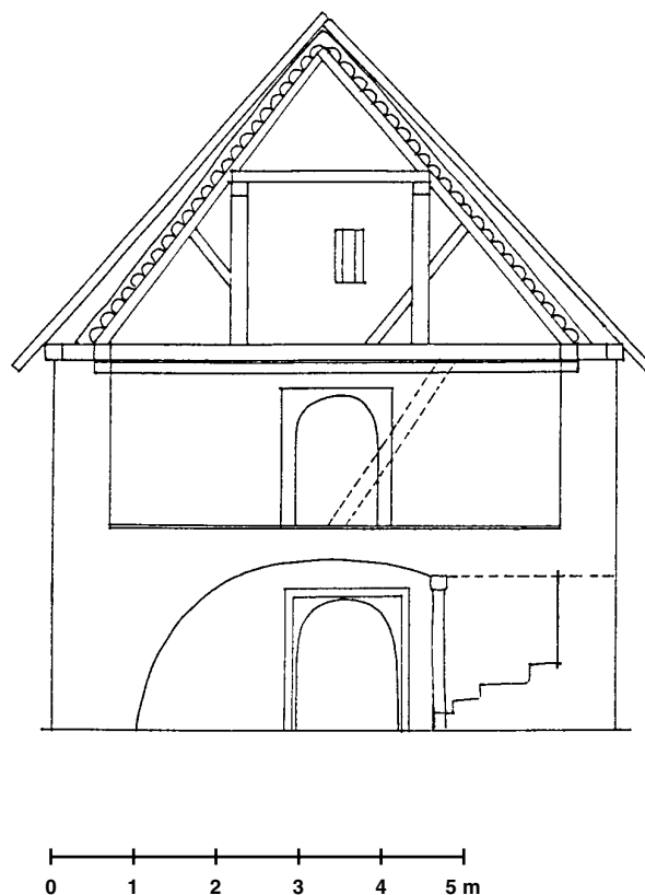
Obr. 9: Horní Jadruž (okr. Tachov), sýpka usedlosti č. 13, půdorys přízemí a příčný řez.
