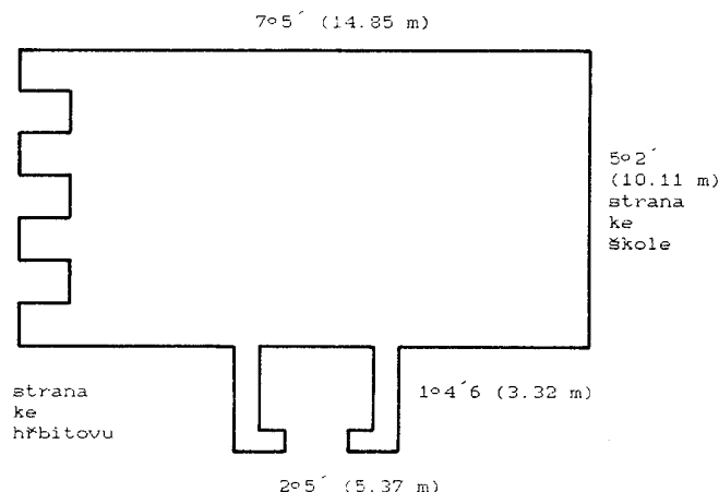
Obr. 14: Rožmberk nad Vltavou, dům čp. 6. Schematický plánec bývalé kaple podle nákresu v dokladech o koupi objektu Matyášem Mittaschem roku 1791; knižní zápis doplněný vlastnoručním Mittaschovým plánkem byl proveden roku 1794 (kresba L. Lancinger, 1997).
