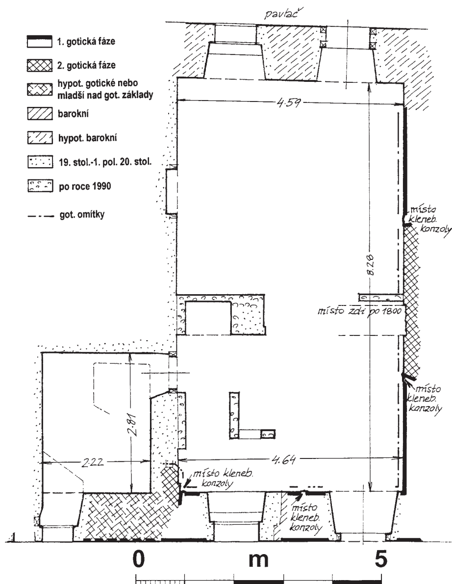
Obr. 6: Rožmbek nad Vltavou, dům čp. 6. Schematický půdorys přízemí domu s vyhodnocením stáří jednotlivých konstrukcí (zaměření a kresba J. Sommer, 1997).
