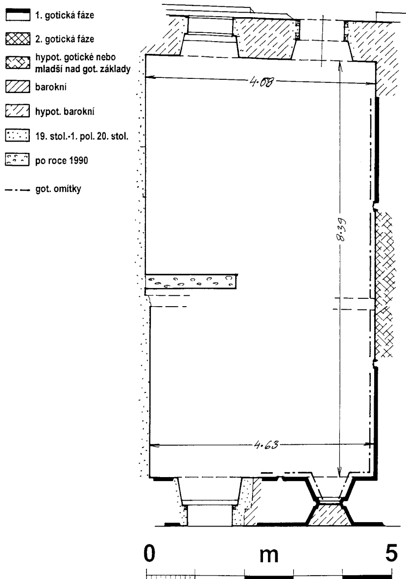
Obr. 7: Rožmberk nad Vltavou, dům čp. 6. Schematický půdorys prvního patra domu s vyhodnocením stáří jednotlivých konstrukcí (zaměření a kresba J. Sommer, 1997).
