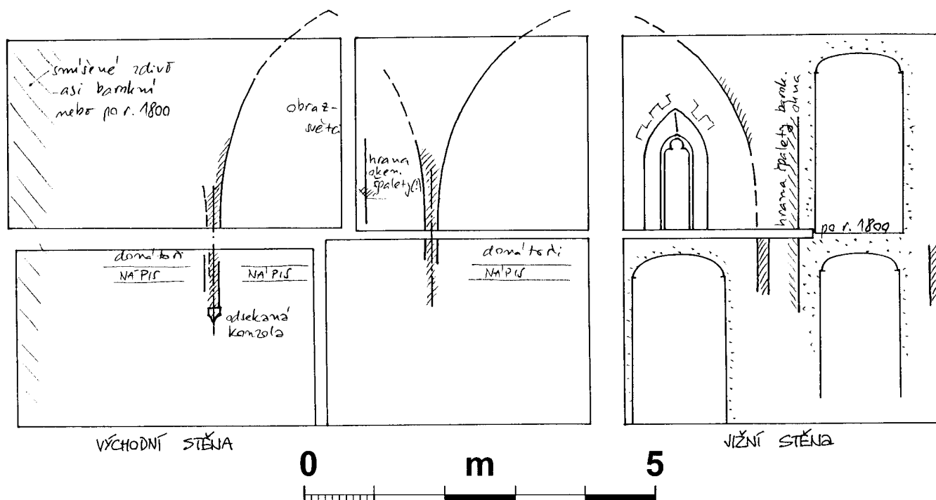
Obr. 8: Rožmberk nad Vltavou, dům čp. 6. Schematický náčrtek vnitřního líce jihovýchodní (vlevo) a jihozápadní (vpravo) stěny domu s vyznačením nalezených pozůstatků gotické kaple. Plná čára - zjištěné hrany čelních oblouků gotické klenby, přerušovaná čára - doplněné tvary čelních oblouků, šrafura - zjištěné stopy odsekaných kamenických článků (zaměření a kresba J. Sommer, 1997).
