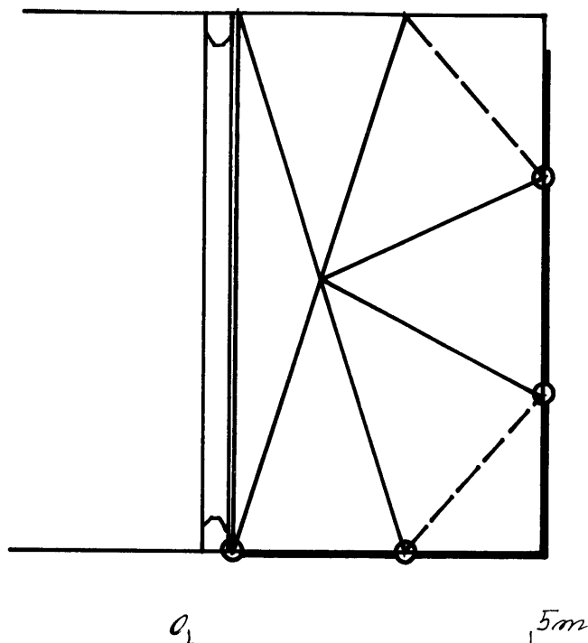
Obr. 15: Rožmberk nad Vltavou, dům čp. 6. Půdorysný náčrt rekonstrukce klenebního obrazce kaple. Kroužky označují polohy doložených klenebních výběhů. Plnými čarami jsou označeny linie žebër, jejichž existenci můžeme považovat za jistou. Čárkovanými čarami jsou vyznačena pravděpodobná žebra, oddělující koutová pole. Je možné, že v klenbě byla ještě další žebra, která mohla vytvářet hvězdovitý obrazec (kresba J. Sommer, 2000).
