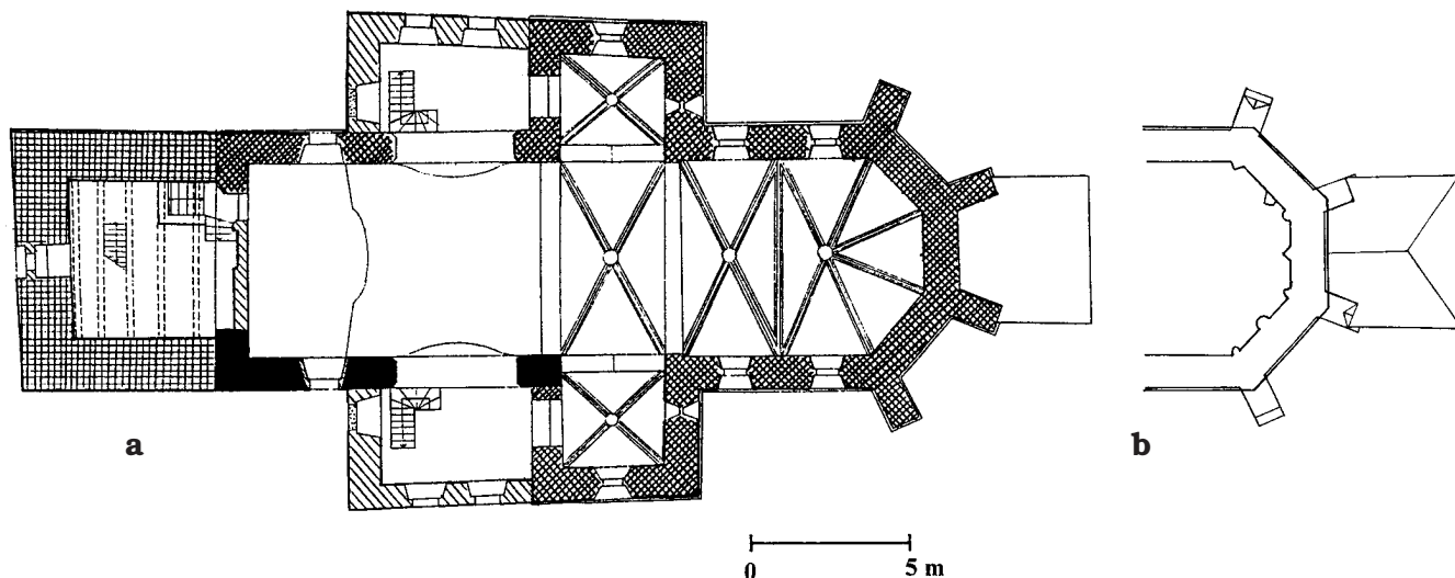
Obr. 3: Kostelec nad Vltavou, kostel Narození P. Marie, a - půdorys v úrovni 1. patra věže, b - půdorys závěru v úrovni římsy.
