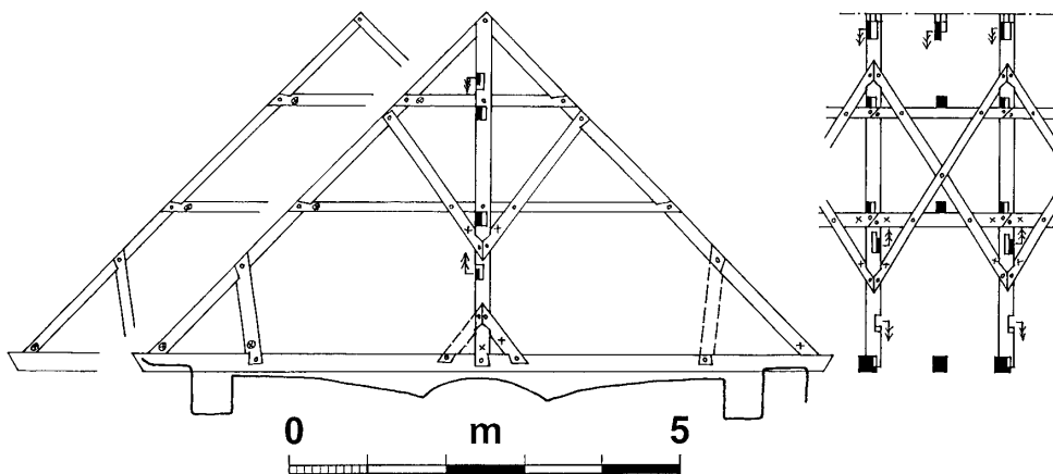
Obr. 21: Čížová, kostel sv. Jakuba Většího. Schematický náčrtek plné vazby krovu presbyteria, vpravo náčrtek podélné vazby v ose krovu, vlevo schéma mezilehlé vazby.
