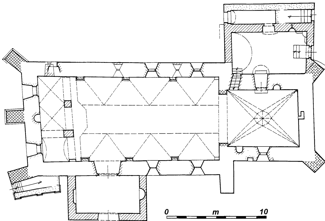
Obr. 2: Čížová, kostel sv. Jakuba Většího. Půdorys kostela s vyznačením stavebního vývoje. Bílé plochy - pozdně románské či raně gotické zdivo z doby kolem poloviny 13. století. Přerušovaná křížkovaná šrafování - opěrné pilíře presbyteria, snad ze 14. nebo z 15. století, možná na starších základech. Křížkovaná šrafování - gotické zdivo ze 14. a z 15. století. Šikmá šrafování zleva dolů - pozdně renesanční nebo raně barokní zdivo ze 16. a 17. století. Šikmá šrafování zleva vzhůru - barokní zdivo z 18. století. Tečkování - 19. století.
