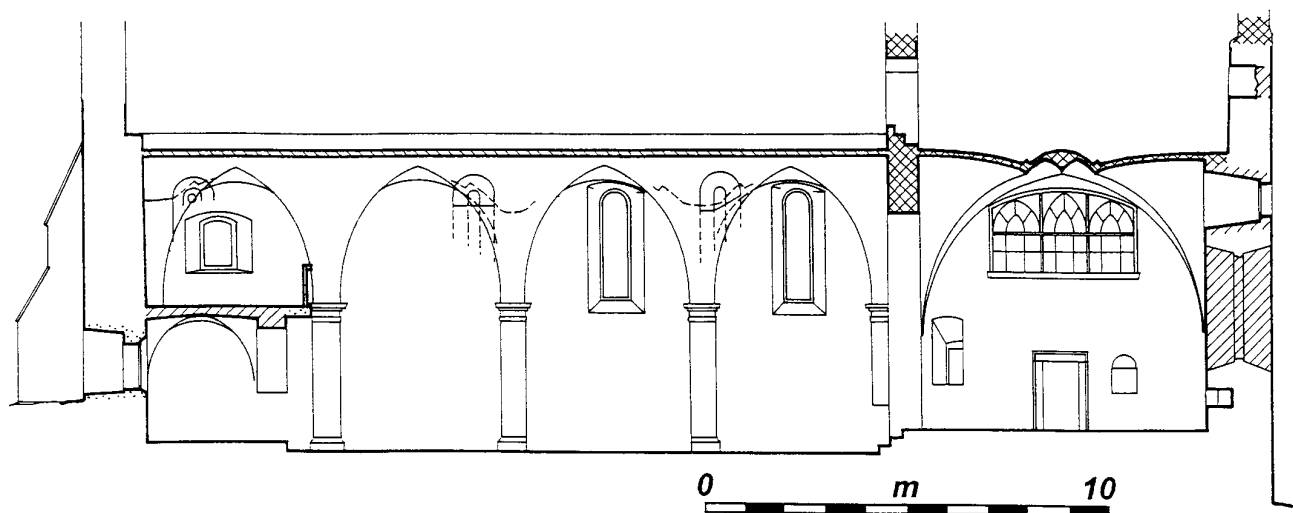
Obr. 3: Čížová, kostel sv. Jakuba Většího. Podélný řez stavbou s pohledem na severní stranu; s vyznačením stavebního vývoje. Bílé plochy - pozdně románské či raně gotické zdivo z doby kolem poloviny 13. století. Křížkovaná šrafování - gotické zdivo ze 14. a z 15. století. Šikmá šrafování zleva dolů - pozdně renesanční nebo raně barokní zdivo ze 16. a 17. století. Šikmá šrafování zleva vzhůru - barokní zdivo z 18. století. Tečkování - 19. století.
