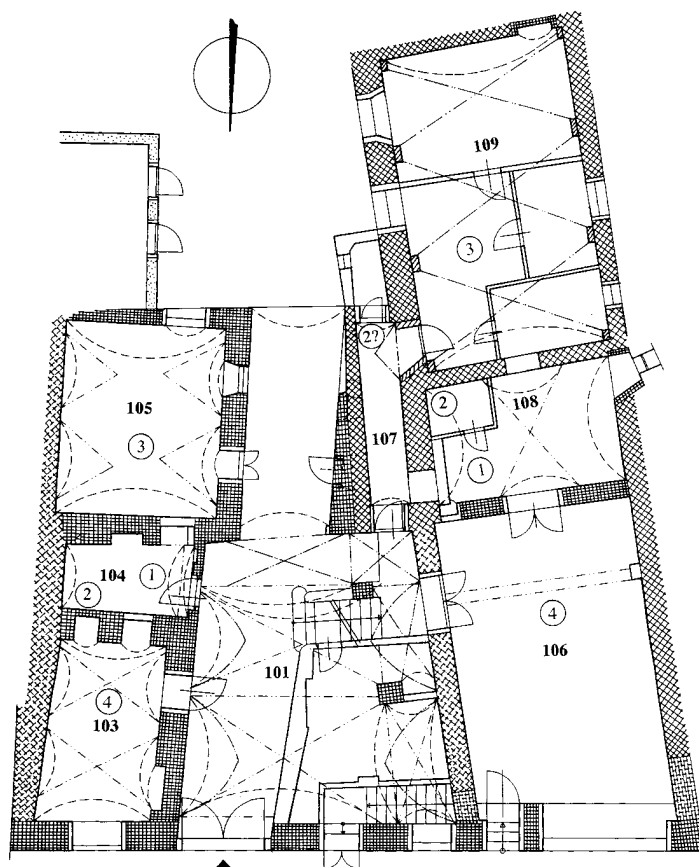
Obr. 6: Znojmo, Zelenářská č. 5, půdorys přízemí, křížkovane šikmo zdivo gotické, přerušované křížkovane šikmo zdivo hypoteticky gotické, křížkovane kolmo zdivo 1. renesanční fáze, přerušované křížkovane kolmo zdivo hypoteticky z 1. renesanční fáze, šrafované šikmo zdivo 2. renesanční fáze, tečkované zdivo pozdně barokní, neznačeno zdivo 19. a 20. století, 1 - síň, 2 - černá kuchyně, 3 - hlavní světnice, 4 - světnička.
