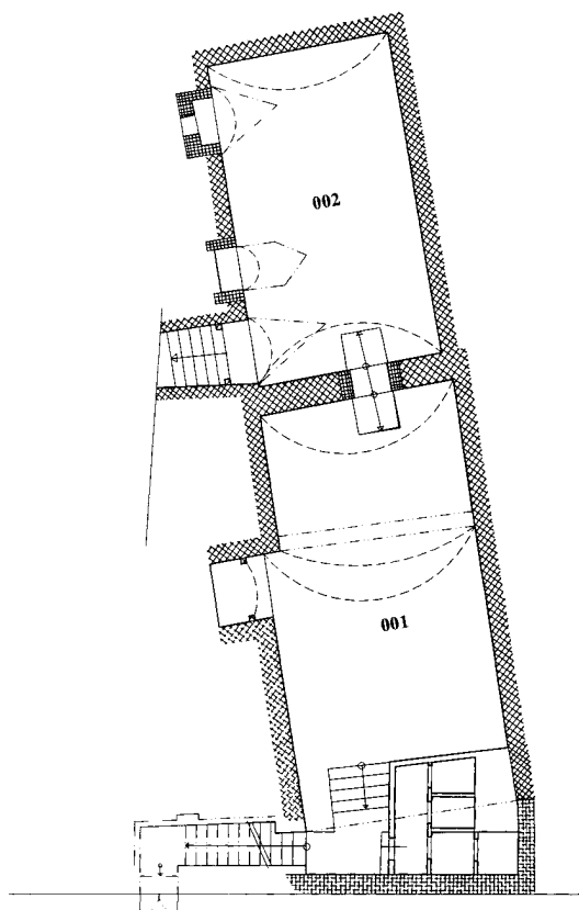
Obr. 4: Znojmo, Zelenářská č. 5, půdorys sklepů, křížkovane šikmo zdivo gotické, přerušované křížkovane šikmo zdivo hypoteticky gotické, křížkovane kolmo zdivo 1. renesanční fáze, přerušované křížkovane kolmo zdivo hypoteticky z 1. renesanční fáze, neznačeno zdivo 19. a 20. století (všechny kresby D. Černoušková).
