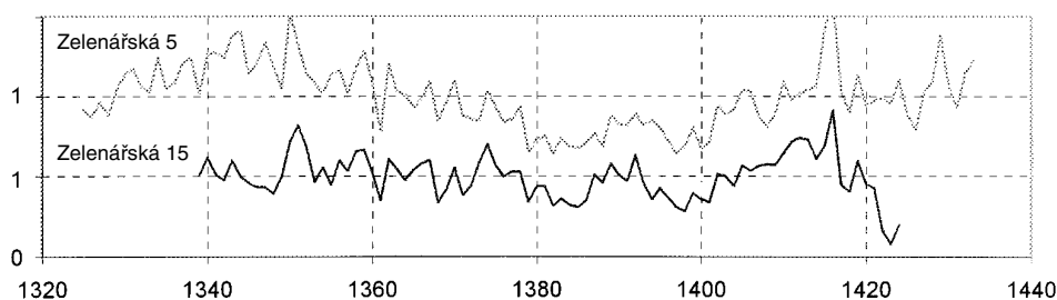
Obr. 10: Srovnání letokruhové řady trámu ze sklepa domu Zelenářská č. 5 se sumární řadou stropních trámů v 1. patře domu Zelenářská č. 15. Nápadná je shoda obou řad nejen v krátkodobém kolísání, ale i ve střednědobých a dlouhodobých trendech (kresba J. Kyncl).
