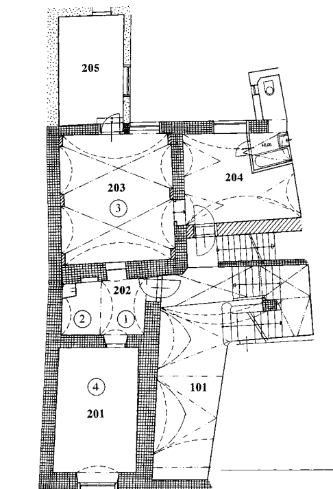
Obr. 5: Znojmo, Zelenářská č. 5, půdorys mezipatra, křížkovane kolmo zdivo 1. renesanční fáze, šrafované šikmo zdivo 2. renesanční fáze, tečkované zdivo hypoteticky pozdně barokní, neznačeno zdivo 19. a 20. století, 1 - síň, 2 - černá kuchyně, 3 - hlavní světnice, 4 - světnička.
