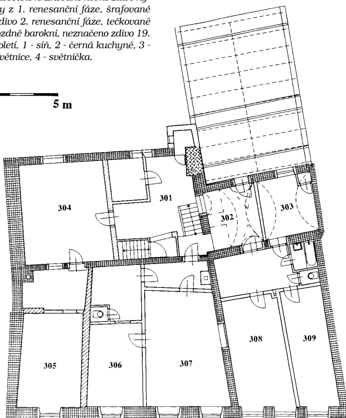
Obr. 7: Znojmo, Zelenářská č. 5, půdorys patra, přerušované křížkovane šikmo zdivo hypoteticky gotické, křížkovane kolmo zdivo 1. renesanční fáze, tečkované zdivo hypoteticky pozdně barokní, neznačeno zdivo 19. a 20. století
