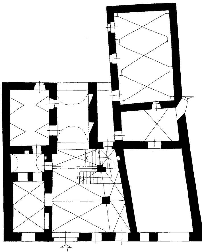
Obr. 8: Znojmo, Zelenářská č. 5, půdorys přízemí podle V. Dražana (Archiv SPÚ Brno).
