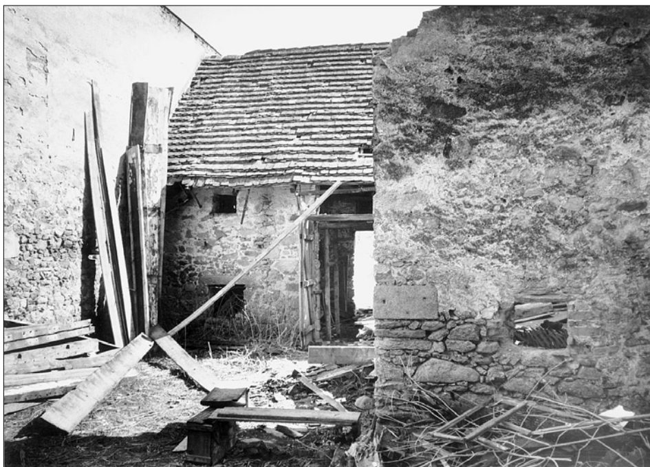
Obr. 8: Vyšší Brod, čp. 30, pohled do dvora od přední budovy, čelo dvorního křídla s druhotně zazděným tesaným kvádrem, v pozadí průjezdná stodola z r. 1881 (stav r. 1997).
