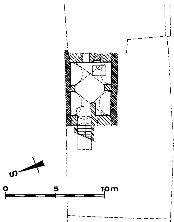
Obr. 5: Vyšší Brod, půdorys sklepa domu čp. 30.
