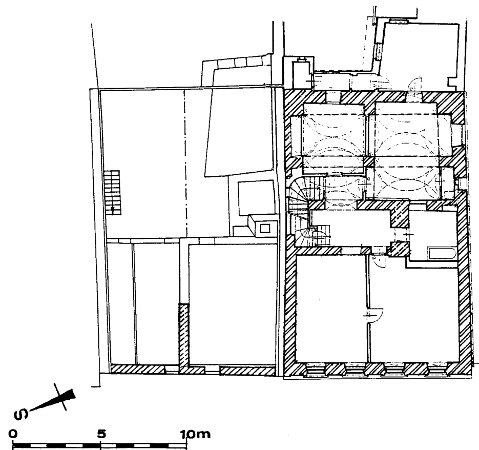
Obr. 4: Vyšší Brod, půdorys 1. patra domů čp. 30 a 31.
