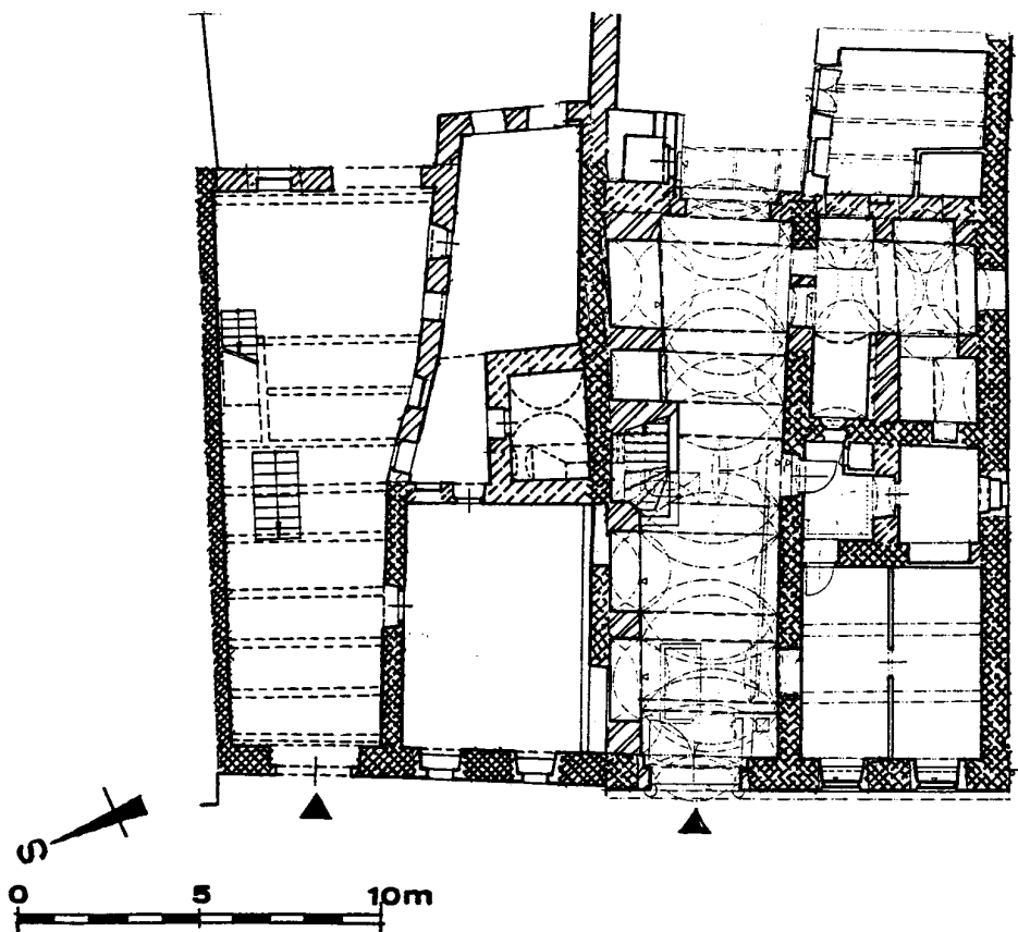
Obr. 3: Vyšší Brod, půdorys přízemí domů čp. 30 a 31 ve stavebně historické analýze. Společná legenda k analytickým plánům: mřížky značí zdivo pozdě gotické, šikmá šrafování - barokní, šikmé dvojčáry - klasicistní, mladší konstrukce ponechány bílé. Přerušované pojednání označuje zařízení hypotetické (kresba autor, 2000).
