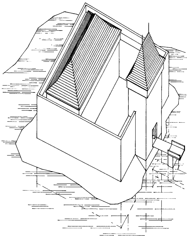
Obr. 26: Kuřivody, zámek. Hmotová rekonstrukce objektu tvrze pro 14. století.
