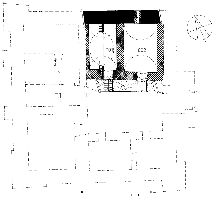
Obr. 4: Kuřivody, zámek. Půdorys suterénu s vyhodnocením stavebního vývoje. Černě - starší gotická etapa asi ze 14. století; zrněně - hypoteticky starší gotická etapa asi ze 14. století; šikmo křížkovaně - mladší gotická etapa asi ze druhé poloviny 15. století a počátku 16. století; kolmo křížkovaně - pozdně renesanční z první čtvrtiny 17. století (přestavba Bohuslava Berky z Dubé); šrafovaně - barokní a mladší úpravy; tečkovaně - úpravy ve druhé polovině 19. a první polovině 20. století, novodobě neznačeno. Na podkladě plánů L. Laigera z roku 1941 zaměřil Jan Pešta a Tomáš Russe, stav v listopadu 2000. Kresba a vyhodnocení Jan Pešta. Legenda platí i pro následující plány.
