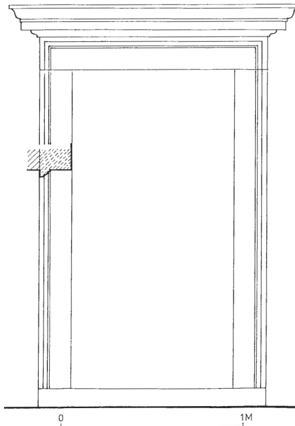
Obr. 22: Kuřivody, zámek. Renesancní portálek ve druhém patře z chodby do jižního křídla (zaměření a kresba J. Pešta).
