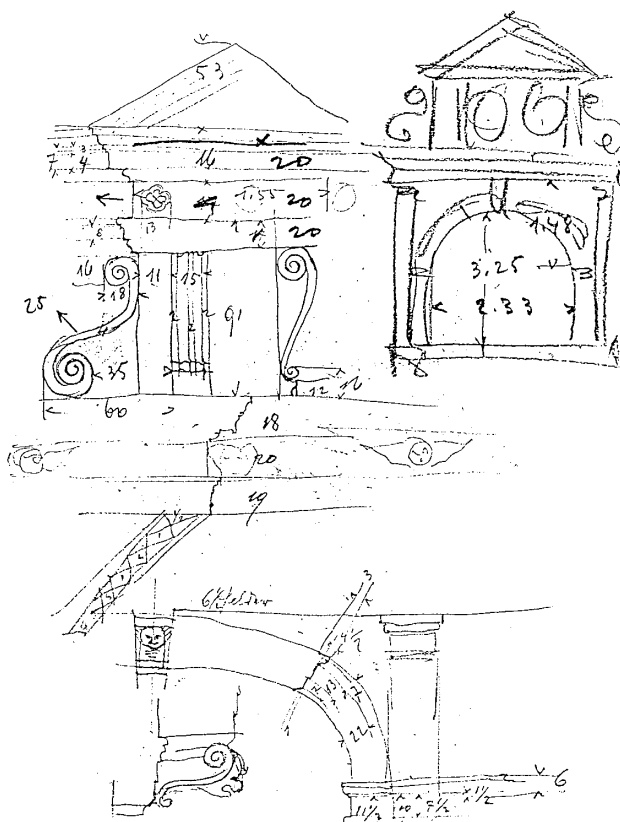
Obr. 9: Skici architektonických detailů hlavního portálu a dnes již neexistujícího nástavce nad portálem, asi z roku 1924. SOA Praha, Správa valdštejnských statků, sign. 36090).
