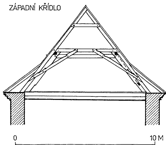
Obr. 23: Kuřivody, zámek. Charakteristické řezy krovem (zaměření M. Fuchs - jižní křídlo a J. Pešta - západní křídlo; kresba J. Pešta).
