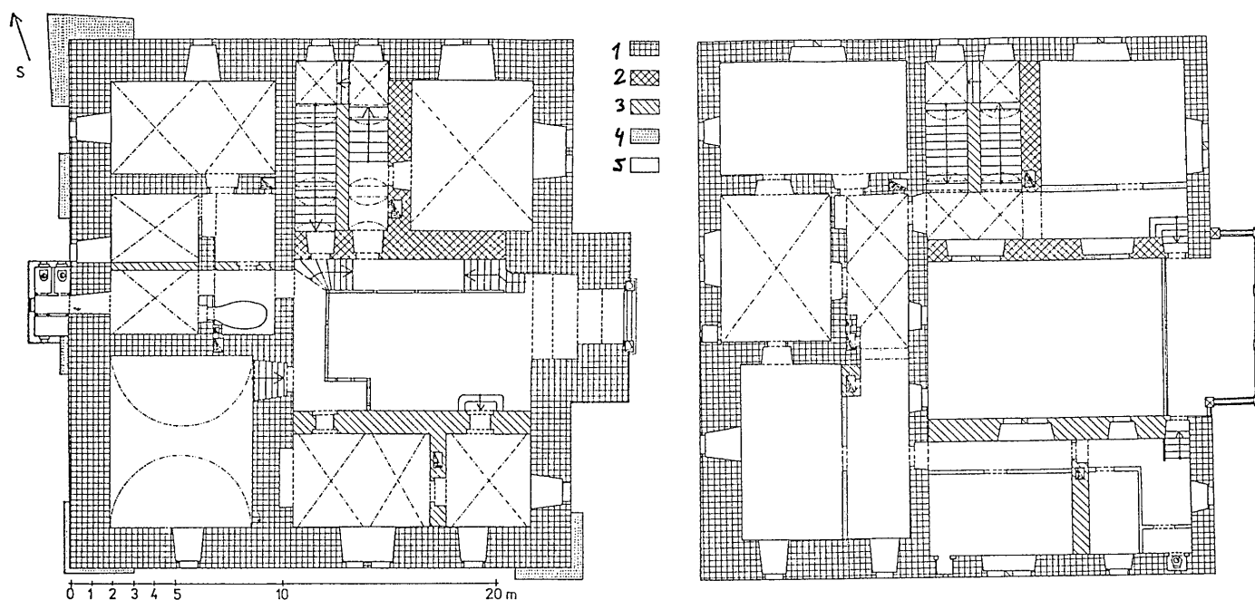
Obr. 12: Kuřivody, zámek. Plán přízemí, prvního a druhého patra zámku na podkladě zaměření L. Laigera z roku 1941 se schematickým vyhodnocením předpokládaného stavebního vývoje, podle J. Úlovce.
