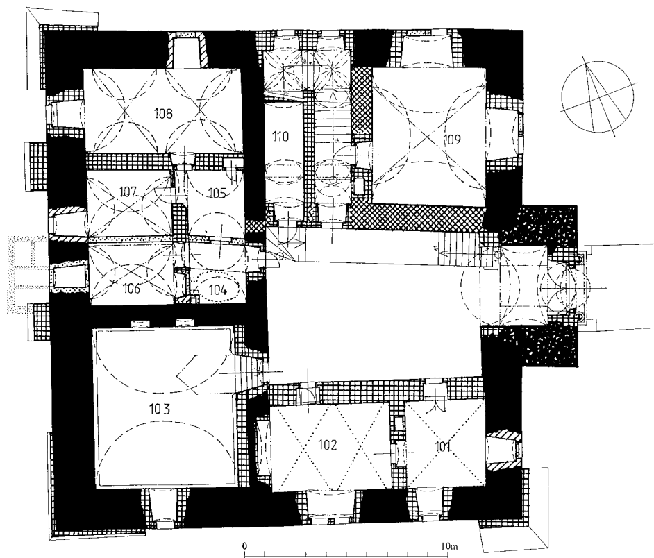
Obr. 5: Kuřivody, zámek. Kuřivody. Půdorys přízemí s vyhodnocením stavebního vývoje.
