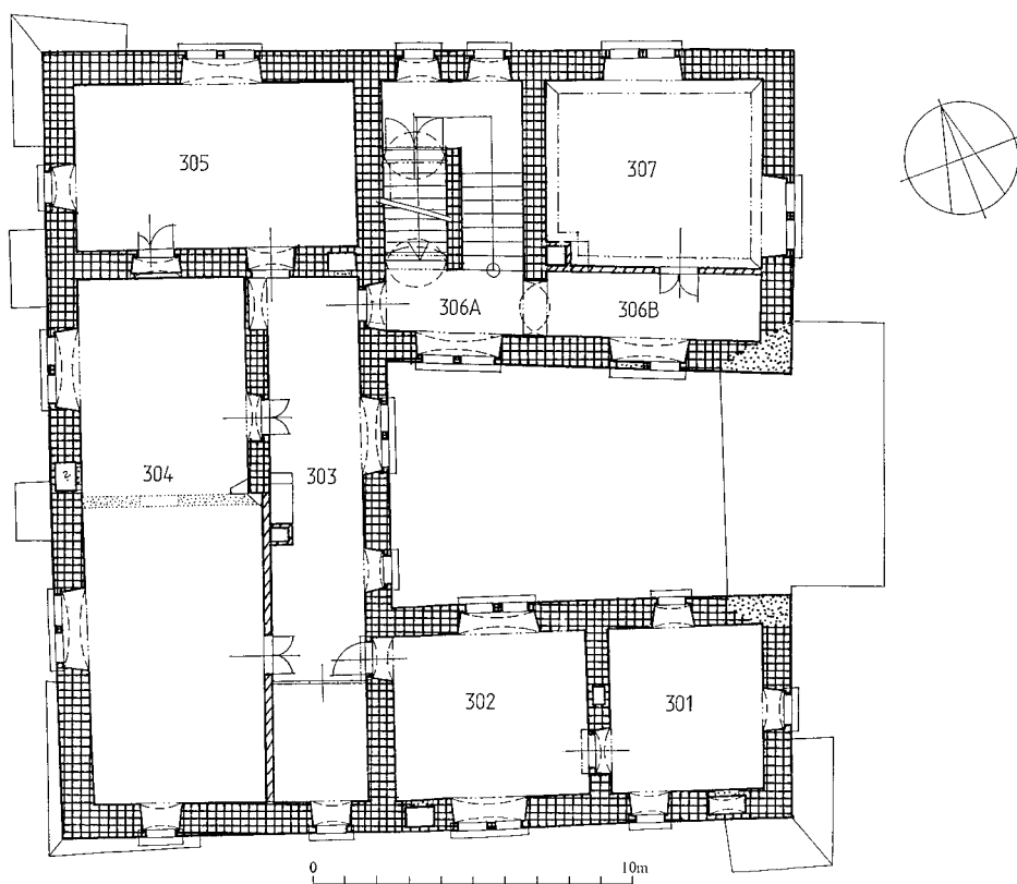
Obr. 7: Kuřivody, zámek. Půdorys druhého patra s vyhodnocením stavebního vývoje.
