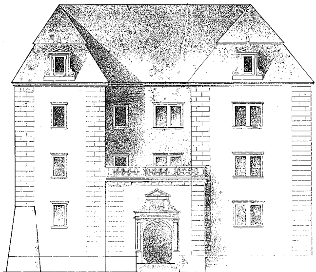
Obr. 10: Kuřivody, zámek. Projekt na přestavbu jižního (ve skutečnosti východního!) průčelí zámku, nedatováno, asi kolem roku 1883 (SOA Praha, Správa valdštejnských statků, sign. 36091).
