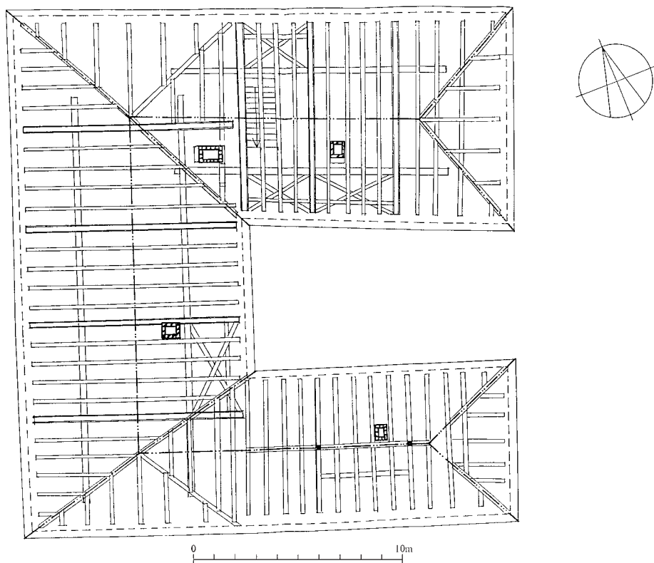
Obr. 8: Kuřivody, zámek. Orientační půdorys krovu.
