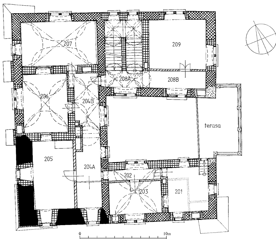
Obr. 6: Kuřivody, zámek. Půdorys prvního patra s vyhodnocením stavebního vývoje.
