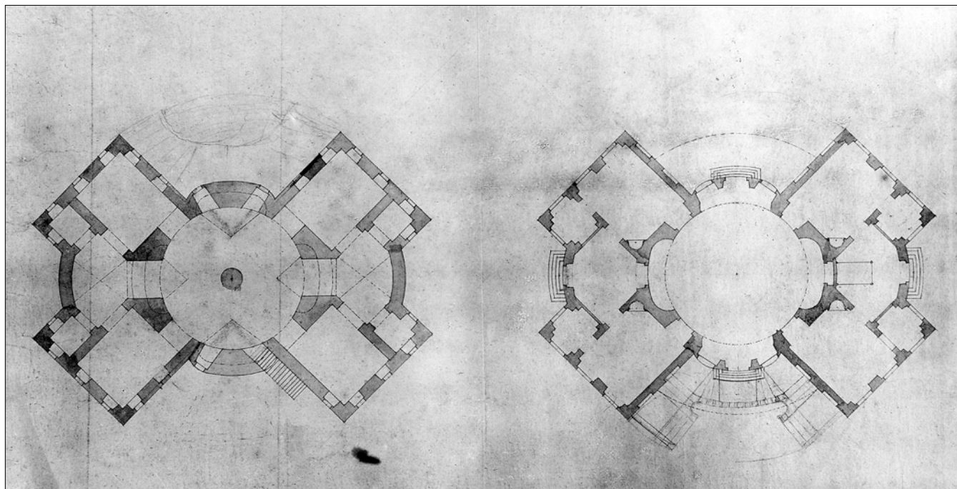
Obr. 4: Plán ke stavbě veltruského zámku z jindřichohradeckého archivu (půdorysy).
