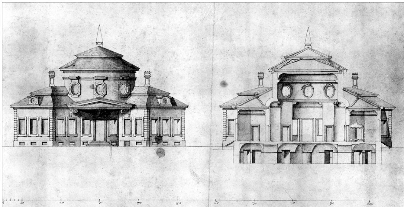
Obr. 5: Plán ke stavbě veltruského zámku z jindřichohradeckého archivu (nárys a řez).
