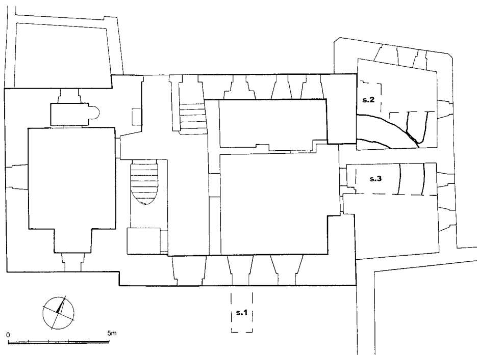
Obr. 6: Vraclav, čp. 115. Rozmístění archeologických sond 1, 2, 3 s vyznačením odkrytého zdiva. Podle plánu ing. K. Doubnera, detail bývalého chléva upřesněn.
