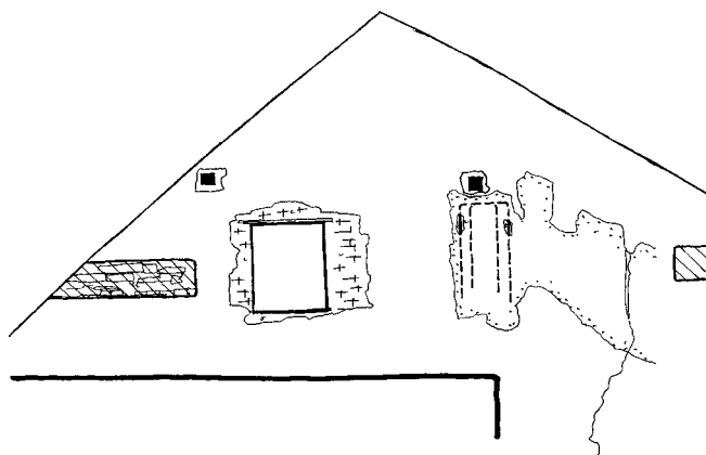
Obr. 17: Vraclav, dům čp. 115. Perspektivní náčrt východního líce východního štítu bývalé lodi kostela sv. Václava. Uprostřed vlevo dodatečně zřízený průchod, vpravo poloha zazděného původního okénka. Šrafirou jsou vyznačeny relikty odsekané profilované římsy, která na východní stěnu lodi zřejmě přecházela z podélných zdí lodi. Zdivo štítu je z lomového kamene; cihlová vyzdívka kolem průchodu je vyznačena křížky (kresba J. Sommer, 2001).
