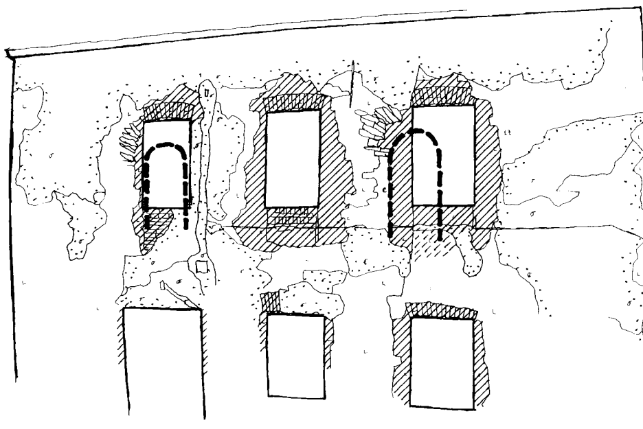
Obr. 13: Vraclav, dům čp. 115. Perspektivní náčrt jižní stěny bývalé lodi kostela sv. Václava. Tečkováním jsou lemovány plochy líce zdiva, kryté dochovanými omítkami; bílé je ponecháno lomové zdivo a cihlové zdivo z první výstavby kostela; šikmá šrafová značí části zdiva, pocházející z úprav z doby kolem poloviny 19. století, provedené převážně z cihlového zdiva (kresba J. Sommer, 2001).
