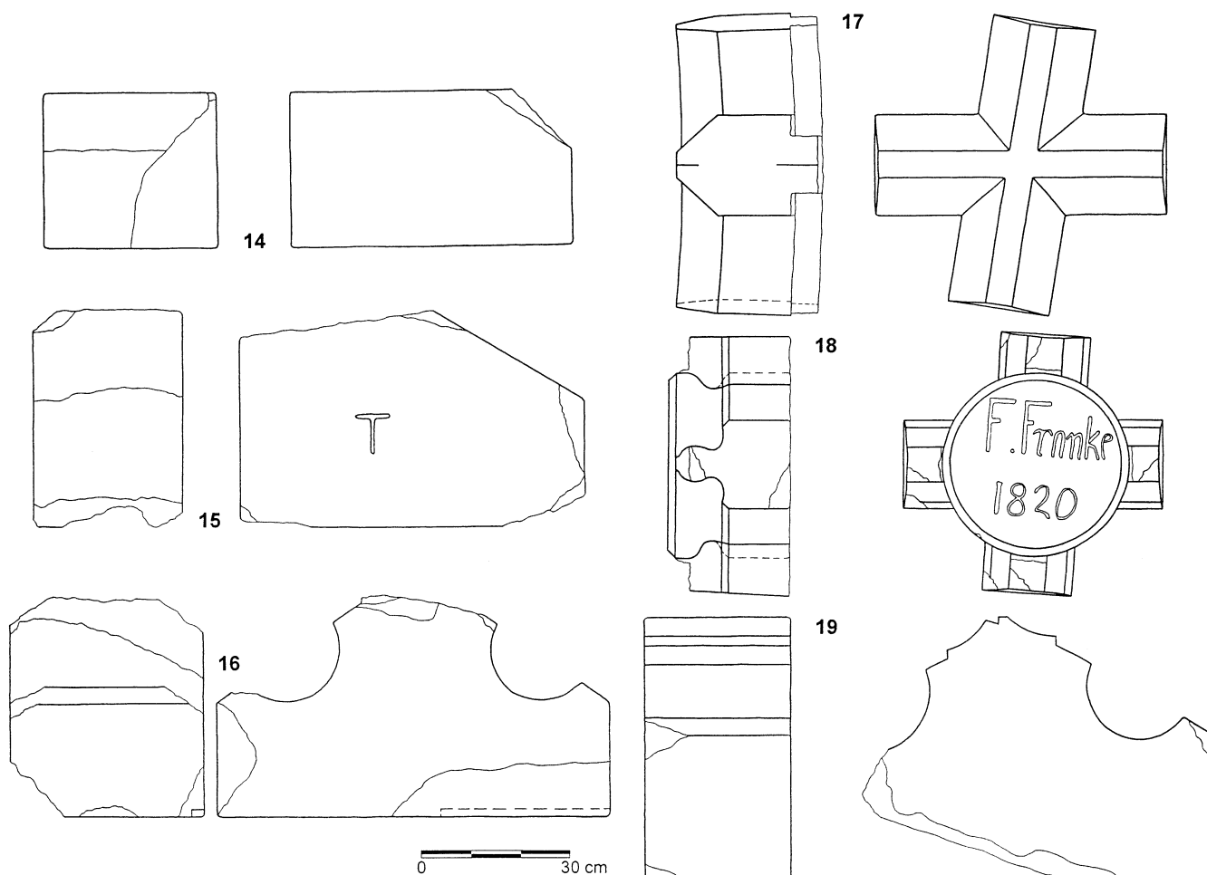
Obr. 13: Architektonické články 14 – 16, skupina 1; architektonické články 17 a 18, skupina 2; článek 19, skupina 3 (kresba J. Panáčková dle podkladů autorů).
