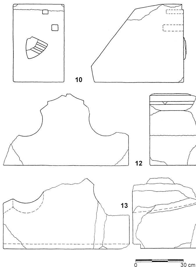
Obr. 10: Architektonické články 10, 12 a 13, skupina 1 (kresba J. Panáčkové dle podkladů autorů).
