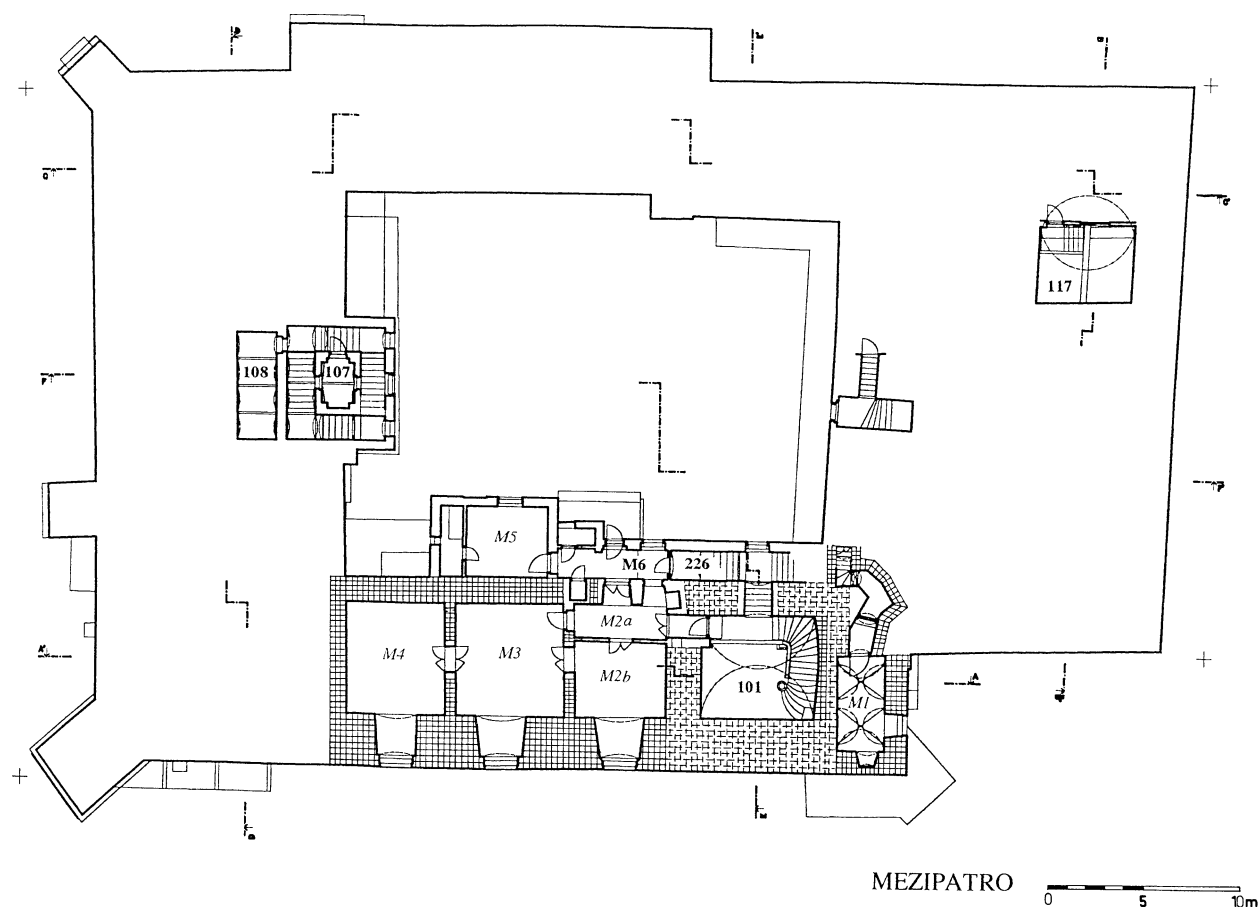
Obr. 5: Prostějov, půdorys mezipatra zámku s vyznačením stavebního vývoje (kresba D. Černoušková).
