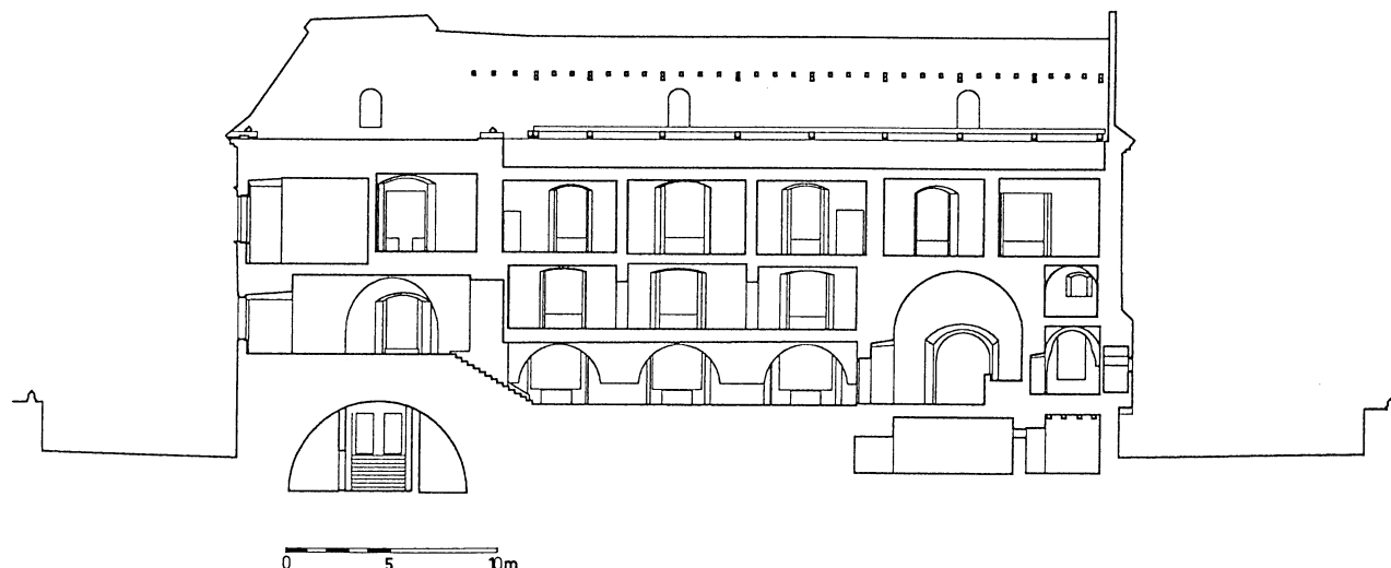
Obr. 7: Prostějov, podélný řez jižním křídlem.
