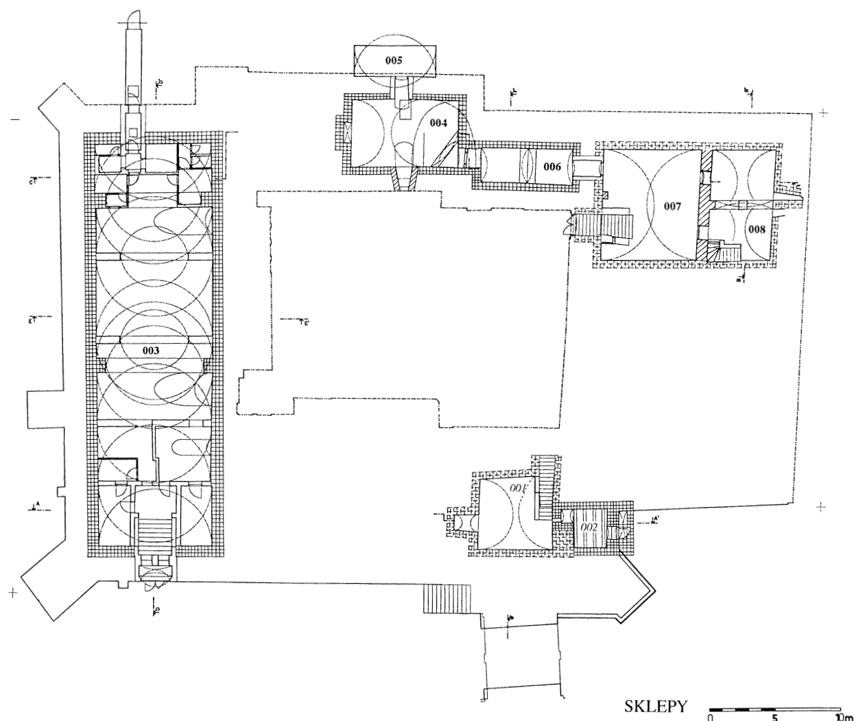
Obr. 4: Prostějov, půdorys sklepů zámku s vyznačením stavebního vývoje (kresba D. Černoušková).
