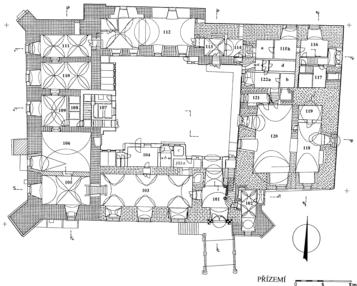
Obr. 3: Prostějov, půdorys přízemí zámku s vyznačením stavebního vývoje. Legenda: přerušované šikmo křížkované – zdívo pozdně gotické (hypoteticky předbrání Kostecké brány), přerušované kolmo křížkované – hypoteticky zdívo z doby Viléma z Pernštejna (do 1521), kolmo křížkované – zdívo z doby Jana z Pernštejna (1522 – 1531), šachovnicový motiv – portál Vratislava z Pernštejna (1568 – 1571), šrafovane – zdívo barokní, mladší úpravy neznačeny (kresba D. Černoušková).
