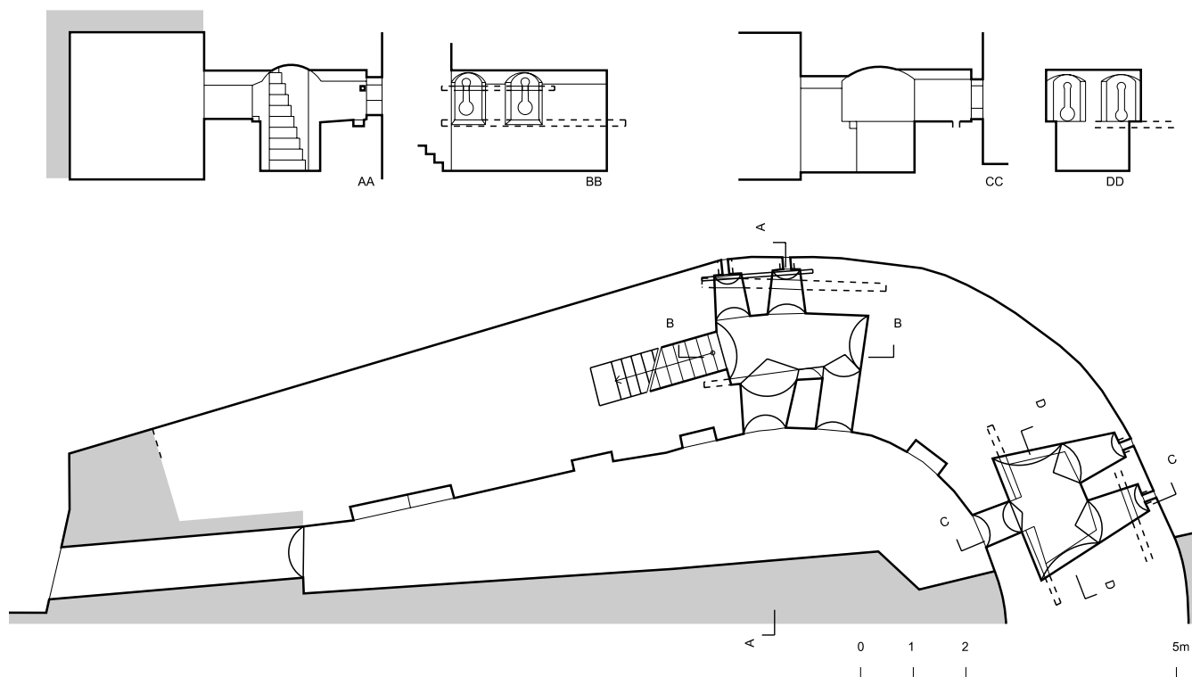
Obr. 22: Louny, velká bašta na severovýchodním nároží vnější hradby, zaměření dochované části stavby. Půdorys přízemí a detaily střilnových komor (zaměření V. Stodola, 1997, doplnění V. Razím a J. Klempíř, 2002).
