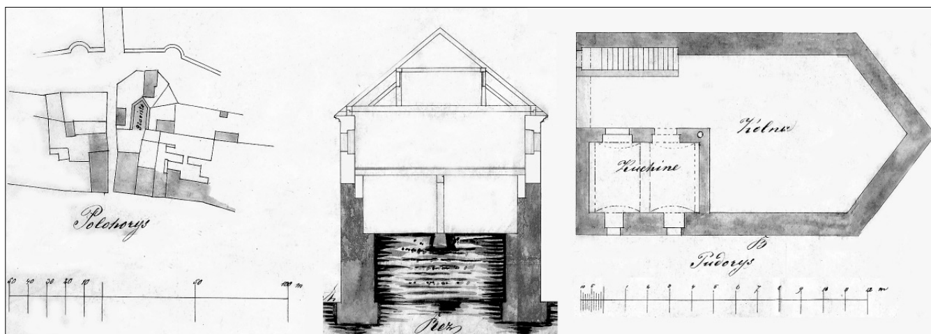
Obr. 12: Louny, plán přestavby velké parkánové bašty za čp. 156–157 na jižní straně města na sýpku z roku 1879 (výřez). Situace, půdorys přízemí a příčný řez (SOKA Louny).
