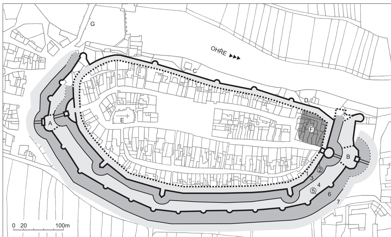
Obr. 4: Louny, plán města podle tzv. císařského otisku mapy stabilního katastru z roku 1843 (srov. obr. 3), pokus o rekonstrukci plánu opevnění v době kolem roku 1600. 1 – předpokládaná trasa hlavní hradby, v 16. století již nefunkční (vznik patrně ve 2. polovině 13. století), 2 – parkánová hradba, vyznačeny tři velké bašty na jihu a barbakány, nevyznačeny předpokládané bašty půlkruhového půdorysu (vznik hradby snad ve 13. století, významná modernizace kolem roku 1450), 3 – vnitřní příkop, 4 – vnitřní val, 5 – vnější hradba s půlkruhovými baštami a barbakány (vznik v rozpětí konce 15 a 1. čtvrtiny 16. století, doplňky v poslední čtvrtině 16. století), 6 – vnější příkop, 7 – vnější val, A – systém Žatecké brány, B – systém Pražské brány, C – Horní fortna, D – Dolní fortna, E – farní kostel sv. Mikuláše (dříve sv. Kříže), F – přibližný rozsah areálu dominikánského kláštera, zlikvidovaného během husitských válek, G – most přes řeku Ohři (návrh V. Razím, kresba K. Vytečková, zpracoval J. Klempíř).
