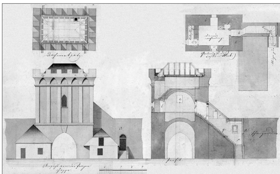
Obr. 27: Louny, Pražská brána vnějšího barbakánu, nere realizovaný plán přestavby z let 1832–1833. Vpravo půdorys 1. patra a řez s pohledem k východu (SOKA Louny, AM Louny, plány I/8).
