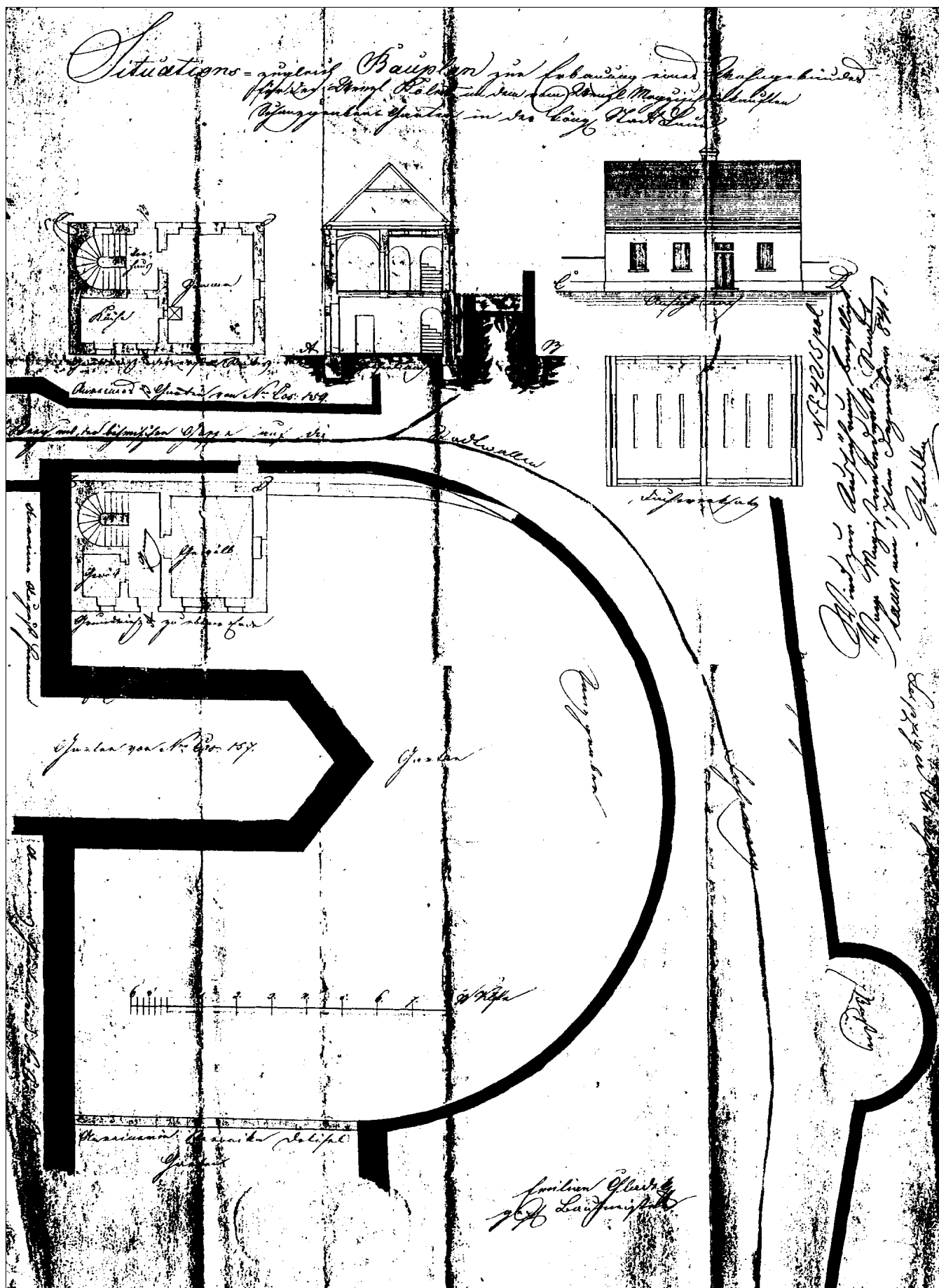
Obr. 11: Louny, plán novostavby domu čp. 333 z roku 1841 se zakreslením části opevnění s velkou parkánovou baštou za čp. 156-157, rozšířenou částí obezděného příkopu před ní a s jednou z bašt vnější hradby (SOKA Louny, AM Louny, plány 1/11).
