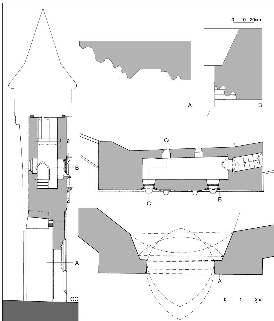
Obr. 39: Louny, Žatecká brána vnějšího barbakánu, příčný řez, půdorys přízemí a 1. patra, profilace vjezdového portálu a okna v 1. patře hlavního průčelí (základní zaměření J. Frühauf a kol., 1995, doplnění, zaměření detailů a kresba J. Klempíř a V. Razím, 2002).
