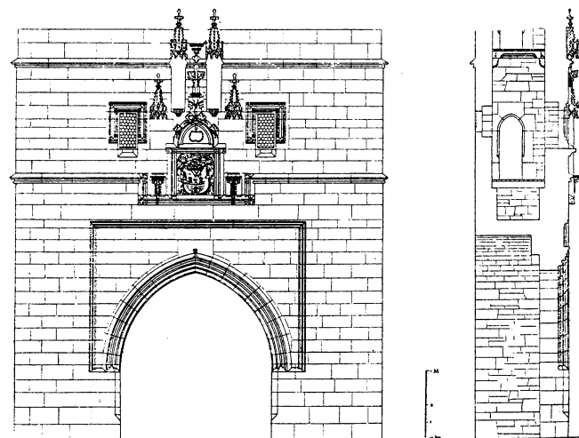
Obr. 38: Louny, Žatecká brána vnějšího barbakánu, příčný řez a hlavní průčelí s pokusem o částečnou rekonstrukci kamenické výzdoby (podle B. Matějky, cit. v pozn. 1, s. 18).
