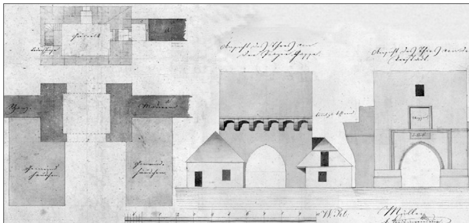
Obr. 26: Louny, Pražská brána vnějšího barbakánu, zaměření z roku 1832. Půdorys přízemí a 1. patra, vnější a vnitřní průčelí (SOKA Louny, AM Louny, plány I/8).
