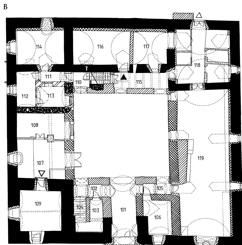
Obr. 3: Třebotov, fara čp. 1 – bývalá tvrz. A – půdorys suterénu s vyhodnocením stavebního vývoje. B – půdorys přízemí s vyhodnocením stavebního vývoje.
