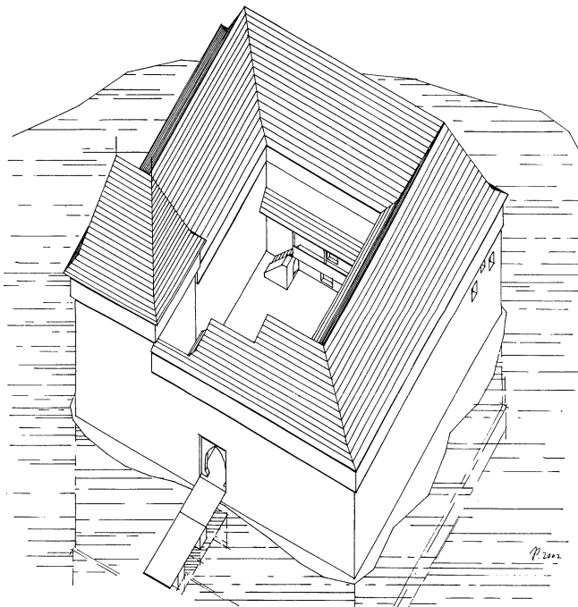
Obr. 21: Třebotov, fara čp. 1 – bývalá tvrz. Hmotová rekonstrukce tvrze po pozdně gotických a renesančních úpravách.
