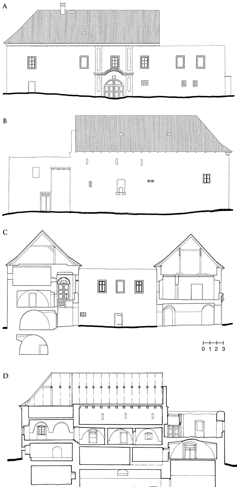
Obr. 6: Třebotov, fara čp. 1 – bývalá tvrz. A – severozápadní (vstupní) průčelí. B – vnější průčelí jihovýchodního křídla (původního paláce). C – příčný řez s pohledem k jihozápadu. Vlevo, jihovýchodní křídlo - bývalý palác s klenutým suterénem, přízemím a prvním patrem a plochostropným sýpkovým druhým patrem. D – podélný řez jižním křídlem (podle výše uvedeného zaměření kresba J. Pešty).
