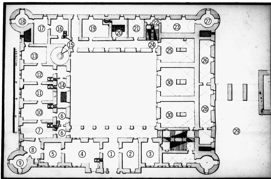
Obr. 8: Kostelec nad Černými lesy, půdorys přízemí vlastního zámku, plán J. Jäger z r. 1779. Tento i následující plány představují návrh barokní přestavby zámku, která se půdorysně kryla s renesančním stavem (dostavěno bylo pouze jihovýchodní nároží s věží, větších změn doznala schodiště), dispozice místností zůstala (kromě východního křídla) více méně zachována. 1 – vstupní brána, 2 – prádelna s přilehlou kuchyňkou, 3 – „sirotčí sklep“, 4 – v tomto prostoru se hned při bráně nacházel malý sklípek na ukládání soli a malá kuchyňka, na něž navazovala „taffelstuben“ – jídelna personálu, 5 – komora se „secretem“, 6 – klenutá síň, 7 – hejtmanský pokoj, 8 – klenutá komora s přístupem do sklepa pod nárožní věží a se „secretem“, 9 – klenutá komora v nárožní věži, 10 – hejtmanská kancelář, 11 – klenutá komora a „dřevnice“, 12 – fraucimor a 13 – fraucimorská komora se „secretem“, 14 – síňka s „vohništěm pro strojení jídla“ a druhým vstupem do „dřevnice“, 15 – síňka s přístupem ke šneku, 16 – klenutá světnice s kamny, 17 – klenutá komora se „secretem“, 18 – komora v nárožní věži, 19 – klenutá síň se studnou a za ní směrem k severu „secret vobecní“, 20 – hlavní zámecká kuchyně, 21 – síňka, spížárna a světnice pro kuchaře, 22 – klenutá komora, 23 – zadní komora, 24 – na místě barokního schodiště se původně nacházel „šnek“ o 97 schodech, přístupný přímo z nádvoří a vedoucí až do podstřeší, 25 – „sklep povrchní z kamene silného a štukoví klenutého“, 26 – „ulice klenutá“ – chodba, do níž byl vchod z předchozího „sklepa“ a která propojovala prostory celého křídla s bažantnicí, 27 – komora ve věži, přístupná z „ulice“, 28 – původní šnekové schodiště do prvního patra zakončené padacími dveřmi, 29 – nároží v renesančním období nedokončené, nacházela se zde bažantnice, 30 – dva nadzemní sklepy.
