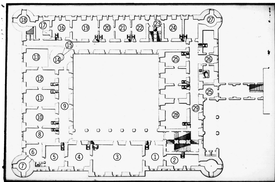
Obr. 9: Kostelec nad Černými lesy, půdorys prvního patra vlastního zámku, plán J. Jágra z roku 1779. 1 – „pokoj stříbrný“ – pokoj pána domu, 2 – komora pána domu se „secretem“ a vstupem na dřevěnou pavlač vedoucí do východního křídla, 3 – „hlavní neb životní taffelstuben“, 4 – pokoj s podlahou „z vápna litou“ a kazetovým stropem malovaným „poetickými figurami“, 5 – komora s „vlaským komínem“, stropem „v okrouhlost klenutým“ a vymalovaným „na způsob ráje“, na stěnách krajiny, ke komoře přiléhá „secret“, 6 – komora „v okrouhlost klenutá“, 7 – „vejstupek neb rundel“, 8 – „komora klenutá bez malování“ s „vlaským komínem“, 9 – maza-hauz, 10 – pokoj s kazetovým stropem malovaným výjevy z trojské války, 11 – pokoj s kazetovým stropem s malbami sedmi divů světa, 12 – pokoj se „stropem lomeným vypuklým truhlářským dílem dělaným a malovaným“ triumfů římských císařů a řeckých hrdinů, 13 – komora se „secretem“ a kazetovým stropem s alegoriemi sedmi planet a dvanácti znamení zvěrokruhu, 14 – šnekové schodiště, 15 – síňka s malovaným stropem, 16 – pokoj s kazetovým malovaným stropem, 17 – komora s kazetovým stropem a „secretem“, 18 – „rundel klenutý“, 19 – pokoj s kazetovým stropem s alegoriemi sedmi svobodných umění a výjevy z dějin panů ze Smiřic, 20 – komora s kazetovým malovaným stropem a se „secretem“, 21 – komora s malovaným kazetovým stropem, 22 – pokoj s kazetovým malovaným stropem, tři posledně jmenované místnosti měly okna do nádvoří i „do valů“ – v plánu naznačená chodba neexistovala, 23 – malá síňka s kazetovým stropem, 24 – velký pokoj, v němž byly vyzděny dvě malé klenuté komůrky se „secretem“, v pokoji s nacházelo ohniště „pro pálení všelijakých vod“, následující místnosti nelze určit zcela přesně, protože jejich dispozice byla barokní přestavbou změněna, 25 – „veliká síň“ s „vlaským komínem“ a „táflováním stropem skrze patrony malovaným“, jíž se procházelo ke kostelu a kam ústilo šnekové schodiště s padacími dveřmi z přízemí, na síni byla vyzděna malá klenutá komůrka bez oken, okna síně ústila do nádvoří, dvě byla obrácena ke kostelu, 26 – pokoj „slove k bílému koníčku“ s kazetovým stropem s malbami krajín, z něj směrem k severu komora, z níž byl vchod do „rundele sklenutého“ (27), 28 – pokoj s nedokončenými kamny a kazetovým stropem, vedle něj klenutá komora, 29 – z velké síně před vstupem na most ke kostelu se směrem k jihu vcházelo do malé síňky se „secretem“, odtud do světnice s kazetovým stropem malovaným „poetickými figurami“ a se zazděným krbem, odtud opět k jihu se vcházelo do „sklepu klenutého, slove Raje“, který byl vymalovaný obrazy krajín s ptactvem. Tato místnost byla dřevěnou pavláčkou spojena s komorou pána domu v jižním křídle.
