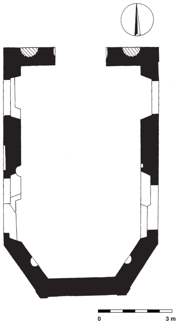
Obr. 2: Půdorys kaple Nejsvětější Trojice a morových patronů sv. Rocha, sv. Šebestiána a sv. Rozálie na Holém vrchu u České Lípy (zaměření K. Podroužek, 2003).
