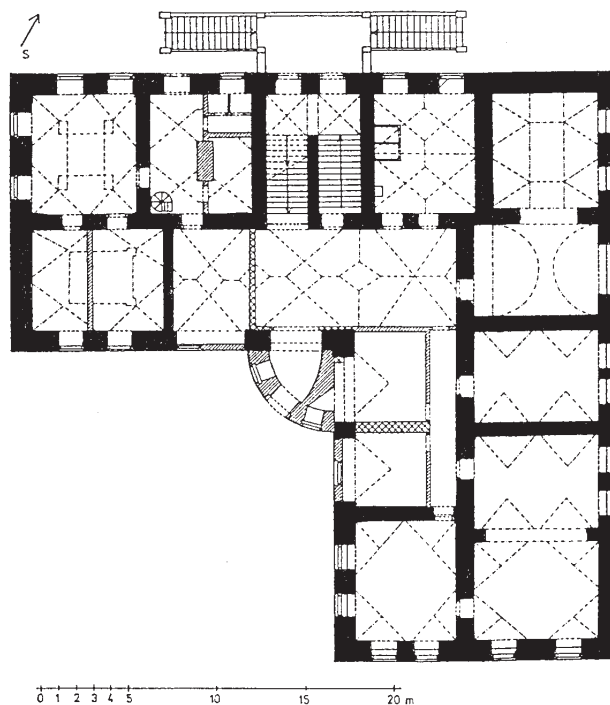
Obr. 13: Prunéřov (okres Chomutov). Půdorys přízemí zbořeného zámku, se schematickým vyhodnocením konstrukcí (převzato z: J. Úlovec, Zaniklé hradby, zámky a tvrze Čech . Praha 2000, s. 238. Upravil autor. Černě vyznačen předpokládaný rozsah pozdně renesančního zámku).
