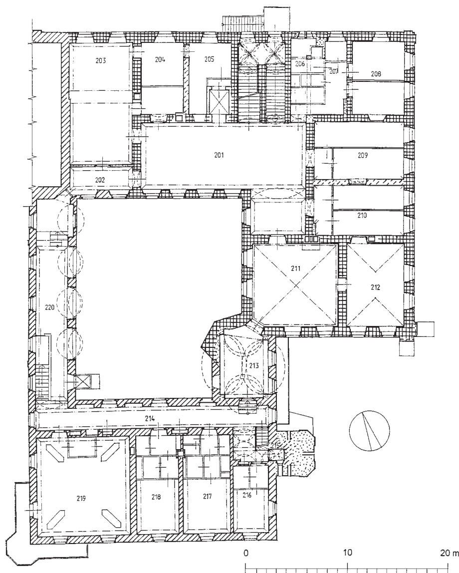
Obr. 7: Žiřetice, zámek – jezuitská rezidence. Půdorys patra 1 : 100 s vyhodnocením stavebního vývoje. 201 – chodba; 211 – místnost s klasicistní (?) klášterní klenbou s neorenesanční malovanou výzdobou; 212 – místnost s renesanční neckovou klenbou; 213 – spojovací krček s klasicistní placovou klenbou; 214 až 218 – barokní přístavba jižního křídla; 219 – spojená místnost s eklektickou alegorickou malovanou výzdobou; 220 – spojovací chodba v patře západního křídla.
