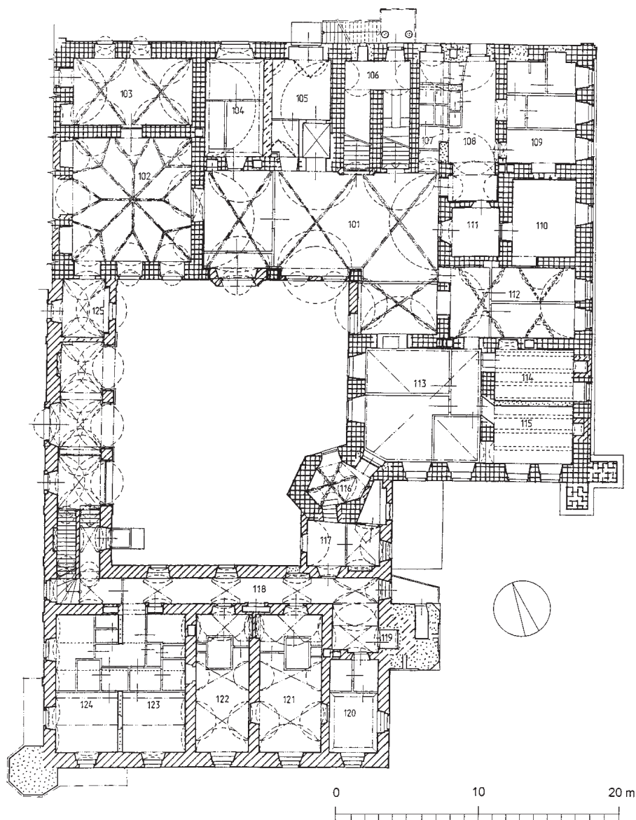
Obr. 6: Žireč, zámek – jezuitská rezidence. Půdorys přízemí 1 : 100 s vyhodnocením stavebního vývoje. 101 – vstupní hala (původně otevřená arkádová vstupní síň); 102 – místnost s renesanční klášterní klenbou; 103 – kaple; 104 + 105, 107 + 108, 112 a 113 – místnosti s nově odhalenými renesančními klenbami; 114 + 115 – místnost s nově odhaleným renesančním trámovým stropem, 109 až 111 – místnosti s předpokládanými renesančními klenbami či stropy, dosud neodhalenými; 116 – podvěží; 117 až 124 – barokní přístavba jižního křídla.
