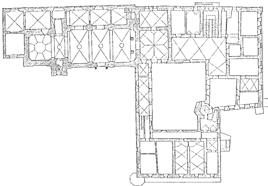
Obr. 12: Žirč, půdorys přízemí kostela sv. Anny a zámku – jezuitské rezidence (převzato z: E. Poche, Soupis památek uměleckých a historických v politickém okrese Královédvorském . Praha 1937).
