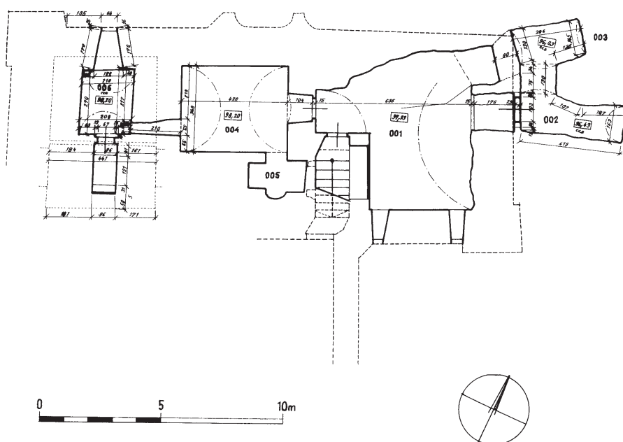
Obr. 6: Zahrádka, půdorys sklepů zámku. (Zaměření a kresba P. Veselý)
