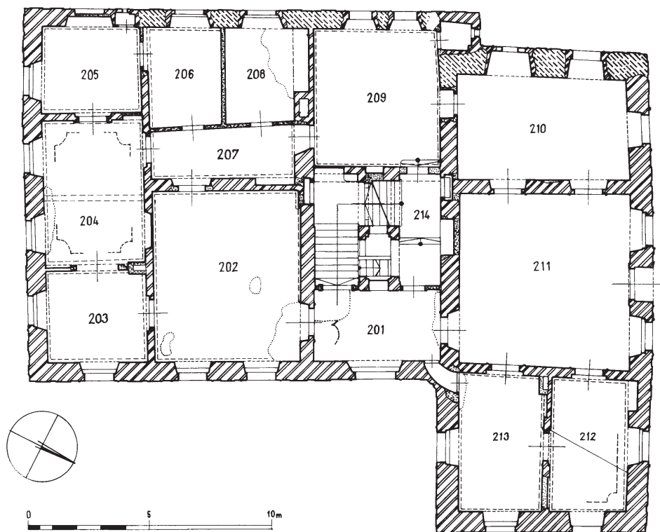
Obr. 7: Zahřádka, půdorys patra zámku s vyznačenými vývojovými fázemi. Křížkované šrafy značí zdivo kladené hypoteticky na přelom 16. a 17. století, přerušované jednoduché šrafy značí zdivo kladené hypoteticky do druhé poloviny 17. století, dvojité šrafy značí zdivo ze dvacátých let 18., století, tečkované značeno zdivo z 19. století. (Zaměření a kresba P. Veselý a J. Veselý)
