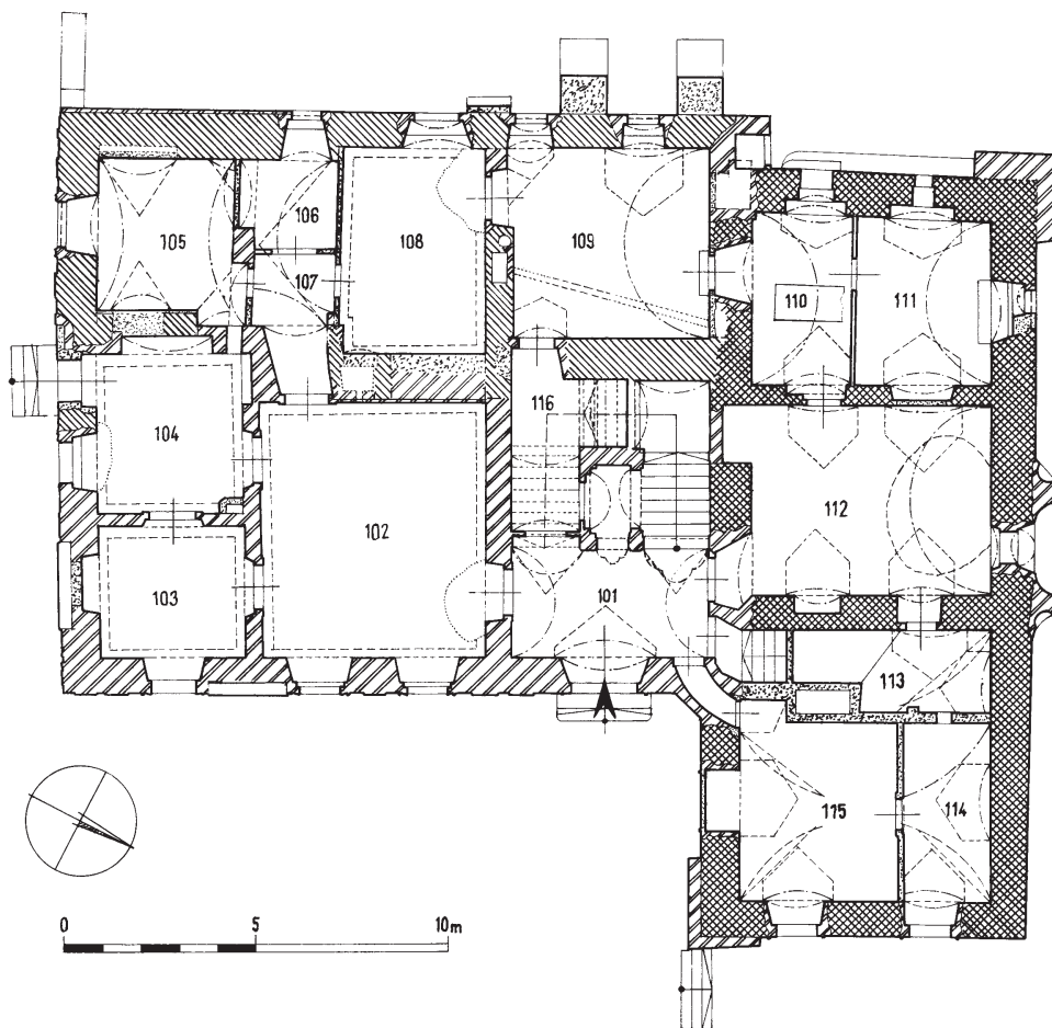
Obr. 5: Zahrádka, půdorys přízemí zámku s vyznačenými vývojovými fázemi: křížkované šrafy značí zdivo kladené hypoteticky na přelom 16. a 17. století, přerušované jednoduché šrafy značí zdivo kladené hypoteticky do druhé poloviny 17. století, dvojité šrafy značí zdivo ze dvacátých let 18. století, tečkované značeno zdivo z 19. století. (Zaměření a kresba P. Veselý a J. Veselý)
