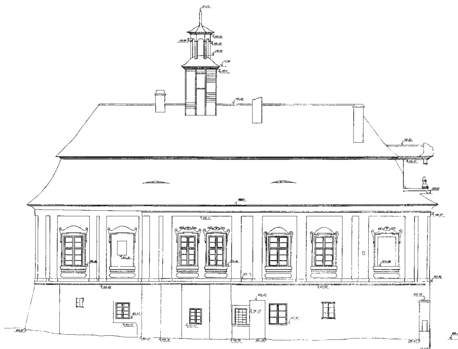
Obr. 14: Zahrádka, zaměření západní fasády zámku (Investis 1975). Na obrázku je zřetelná absence architektonického členění a nepravidelnost v rozmístění oken v přízemí. Jasně je zde rovněž patrné původní členění a výzdoba fasády v patře, dnes téměř bezstopý zaniklé – srov. obr. č. 9.
