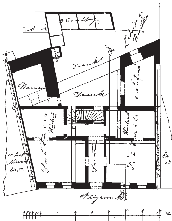
Obr. 23: Jičín. „Nákres k vystavění domu o jednom poschodí, Růžové ulici, čís. popis 51.“ Půdorys přízemí. Kolem 1880 (stavební odbor MÚ Jičín). Plán zachycuje část pravouhlé bašty a dnes již zbořenou partii hradby.
