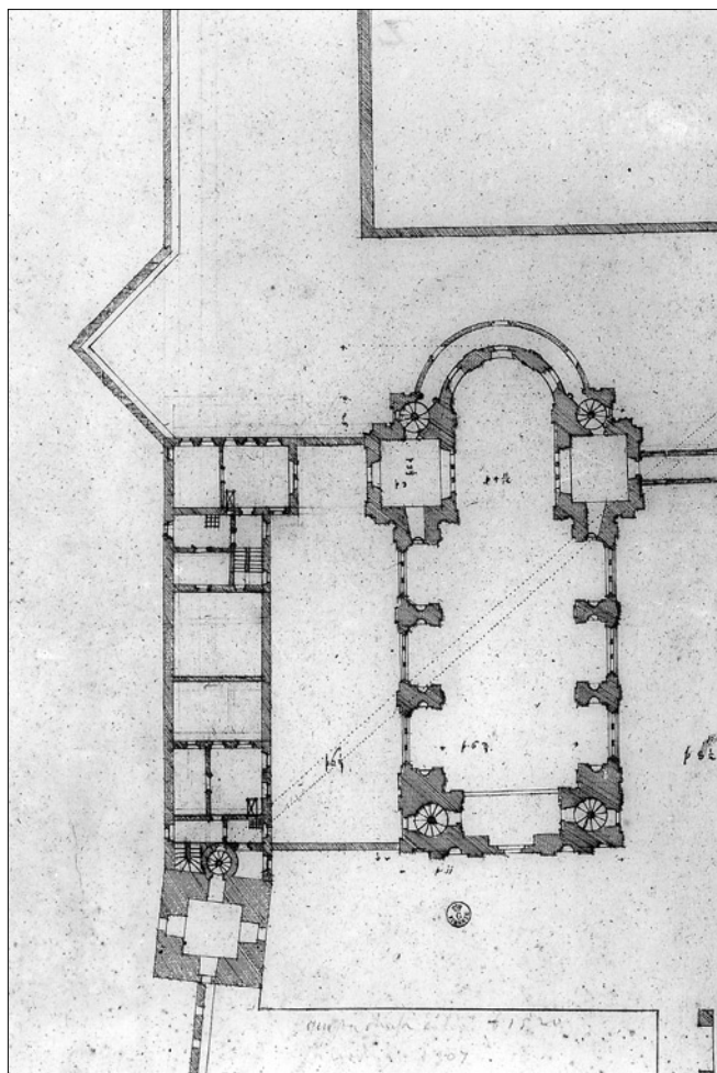
Obr. 9: Jičín. Giovanni Pieroni. Návrh na biskupský kostel sv. Jakuba, budovy biskupství a opevnění u Valdické brány. Půdorys 1. patra. Kolem roku 1624 (podle P. Fídlera, cit. v pozn. 32, s. 32).
