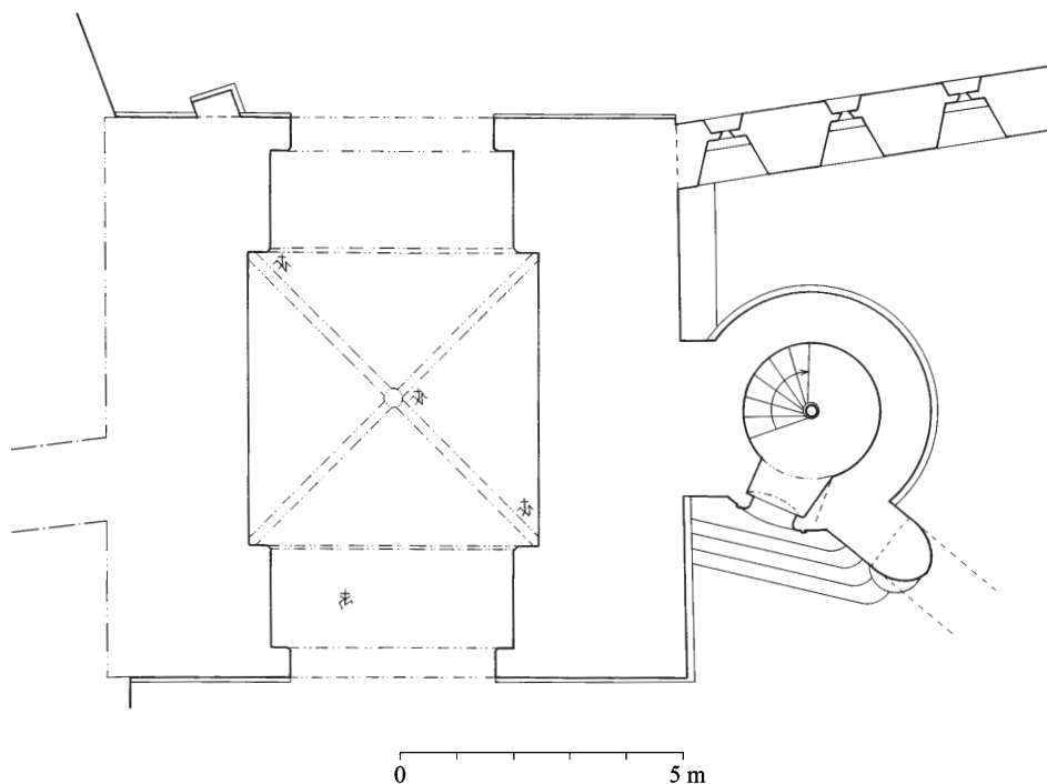
Obr. 8: Jičín. Valdická brána. Půdorys přízemí. Konstrukce brány jsou z roku 1568, klenba datovaná rokem 1578. Valdštejnská hradba postavena kolem 1630. Ve schodišti zbytek starší hradby (zaměření a kresba P. Uličný, 2002).
