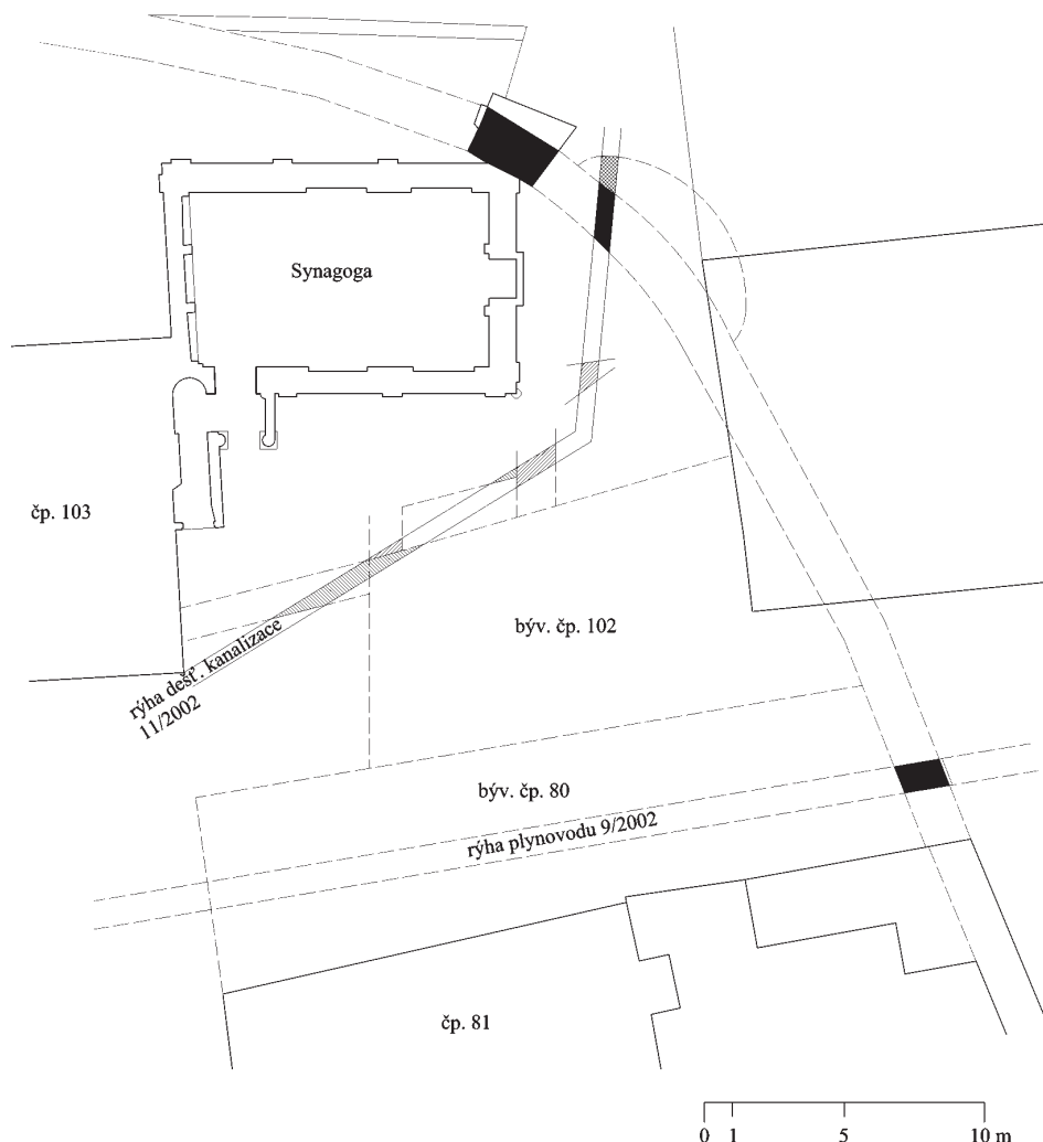
Obr. 29: Jičín. Rekonstrukce opevnění v okolí dnešní synagogy doplněná podle nálezů z výzkumu v roce 2002. Plně znázorněna zachovaná a odhalená hradba, šrafovane odhalená část přístavěné bašty, tečkované předpokládaný průběh hradeb (kresba P. Uličný, 2004).
