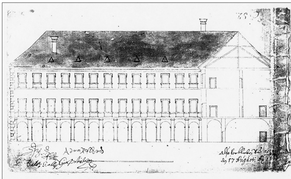
Obr. 3: Projekt II. zámku v Kostomlatech, patrně v dubnu 1666, dvorní fasáda levého křídla.
