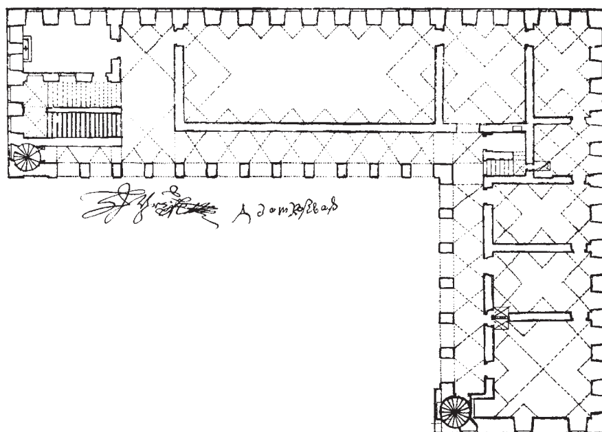
Obr. 2: Projekt II. zámku v Kostomlatech, patrně v dubnu 1666, půdorys přízemí.
