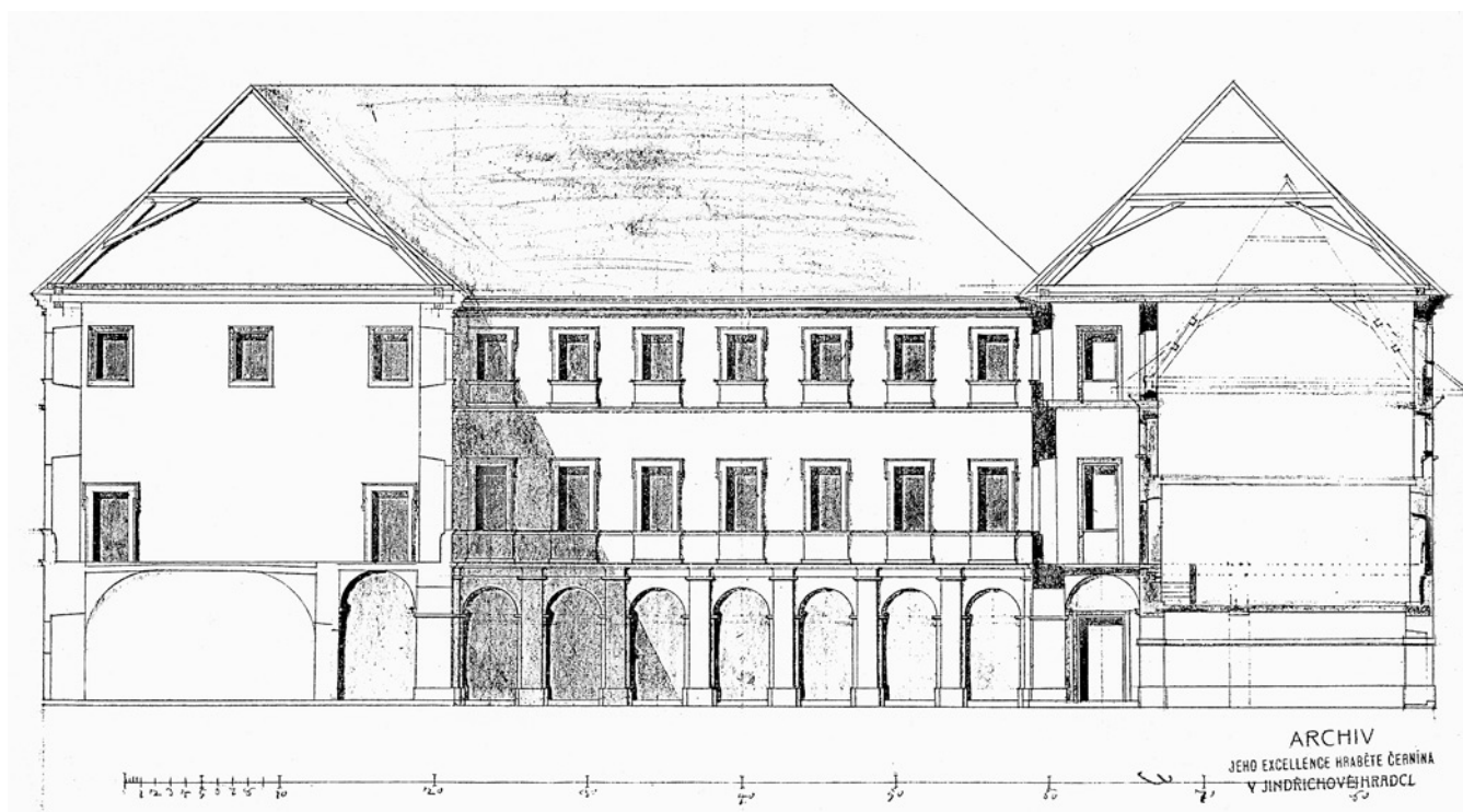
Obr. 6: Projekt I. zámku v Kostomlatech, patrně Marcello Ceresolla v únoru 1666, dvorní fasáda středního křídla v projektu I. Není řešen hlavní portál. Do pravého křídla je pojata starší stavba.
