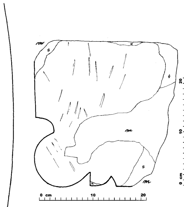
Obr. 4: Divišov, kostel sv. Bartoloměje. Ložná plocha dílu uloženého do zdi- va na severozápadní straně severního schodiště. Značky: „n“ – neopracovaný povrch (lomové plochy); m – malta. Vlevo: zakřivení záklenku (kresleno pomocí somrografu s přesností \pm 2 mm, J. Sommer, 2005).
