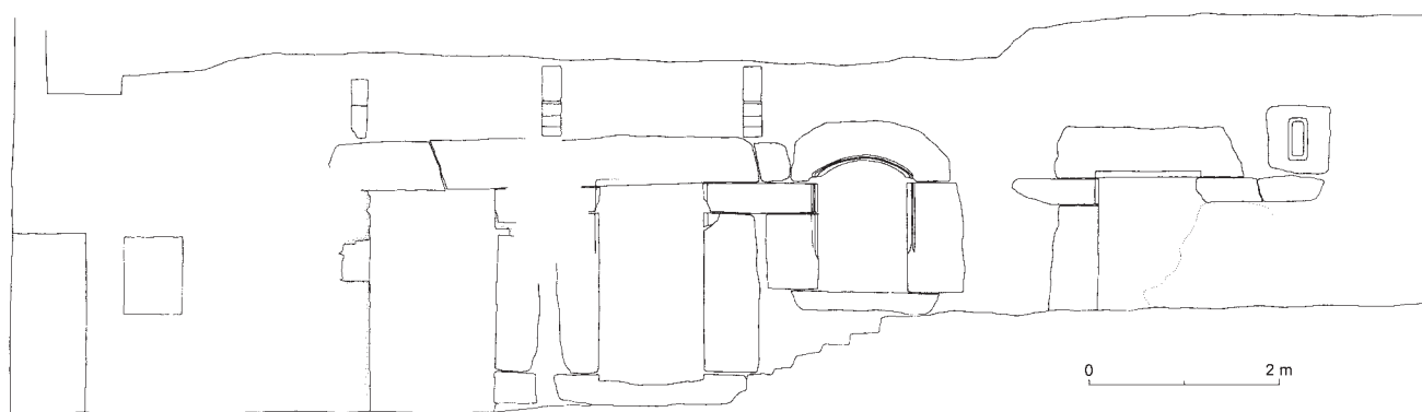
Obr. 22: Černíky, čp. 1. Dvorní průčelí hospodářského objektu ve dvoře usedlosti (kresba a zaměření J. Kypa, 2005).
