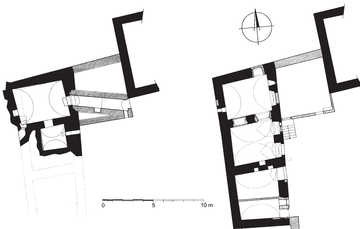
Obr. 21: Černůky, čp. 1. Půdorysy přízemí a sklepa hospodářského objektu ve dvoře usedlosti a západní části obvodového zdiva obytného domu. Tmavě zvýrazněny pozdně středověké konstrukce, šrafovane pobělohorské, zrnitě recentní (kresba J. Veselý, zaměření J. Kypta a J. Veselý, 2005).
