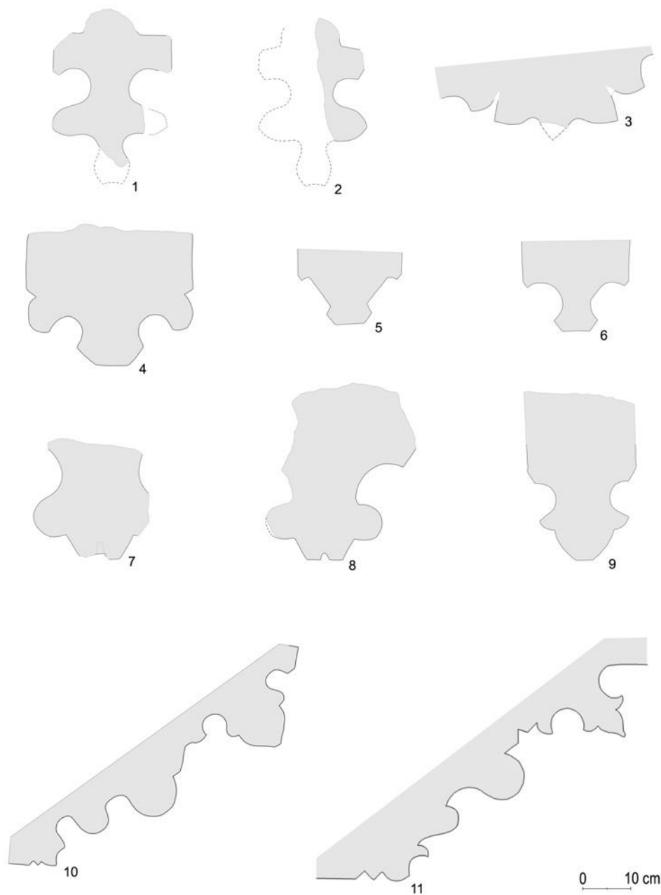
Obr. 1: Srovnávací tabulka vybraných profilů zaměřených autorem (kromě čísla 11) hřebenem s výsuvnými jehlicemi (grafická úprava S. Babušková). U prvků nejsou zakresleny hrany pod úrovní řezu. Prvky 1, 2, 4, 7, 8, 9 jsou uloženy v depozitáři uvedených lokalit. 1 – Břevnov, trojpruté klenební žebro; 2 – Sázava, zlomek trojprutého klenebního žebra; 3 – Strahov, klenební žebro v severním rameni transeptu kostela; 4 – Břevnov, klenební pás; 5 – Sázava, profil klenebního žebra v kryptě v úrovni výběhu; 6 – Sázava, profil klenebního žebra nad výběhem; 7 – Břevnov, okenní ostění; 8 – Sázava, okenní ostění; 9 – Sázava, klenební žebro; 10 – Otruby, profil portálu; 11 – Hodkov, profil portálu podle J. Zacha publikovaný v Památkách archeologických, o. c. v pozn. 30 (upraveno).
