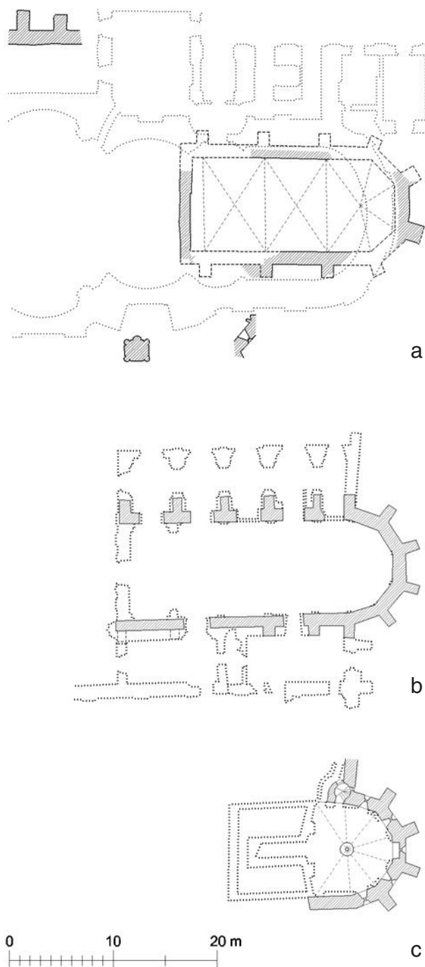
Obr. 3: Srovnání závěrů klášterních kostelů; a – Břevnov – protáhlý presbytář s provizorním uzavřením (severně je zakreslená část jižního ramena ambitu, jižně je zakreslen východní pilíř nedokončeného vícelodí); b – Sázava – gotický presbytář nad kryptou (dle zaměření SÚRPMO, upraveno); c – Sázava – krypta klášterního kostela se schematicky rekonstruovanou kryptou (podle dokumentace M. Klementa a dokumentace SÚRPMO, upraveno; rekonstrukce klenby autor).
