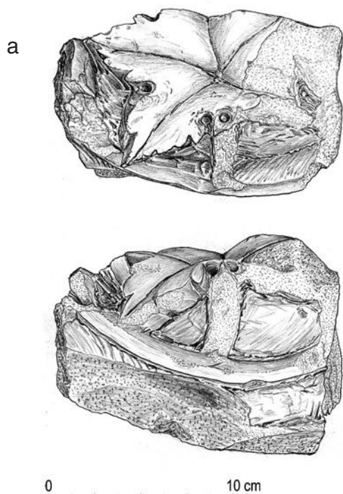
Obr. 2: Břevnovský klášter; dokumentace architektonických článků; a – zlolek architektonické plastiky; b – profil patrně meziokenního pilíře (zaměření autor); c – profil trojprutého klenebního žebra dle starší dokumentace M. Ernesta (zaměření a kresba S. Svatošová).
