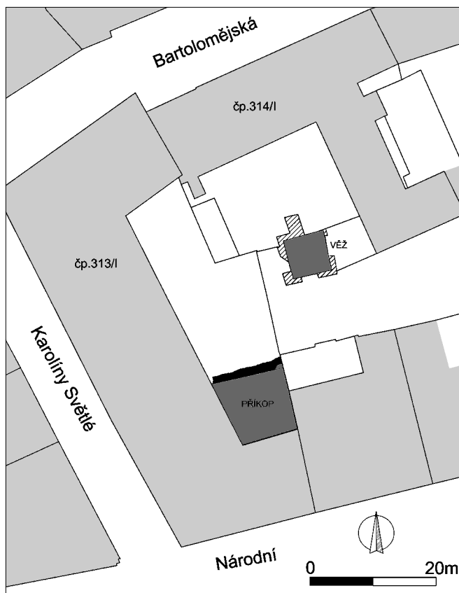
Obr. 3: SMP, situace hradebního příkopu na parcele domu čp. 313/I na Národní třídě a hradební věž na parcele domu čp. 314/I. Černě vyzdívka vnitřní stěny příkopu, šrafovane mladší přístavby k hradební věži a šedě příkop (kresba J. Hlavatý).
