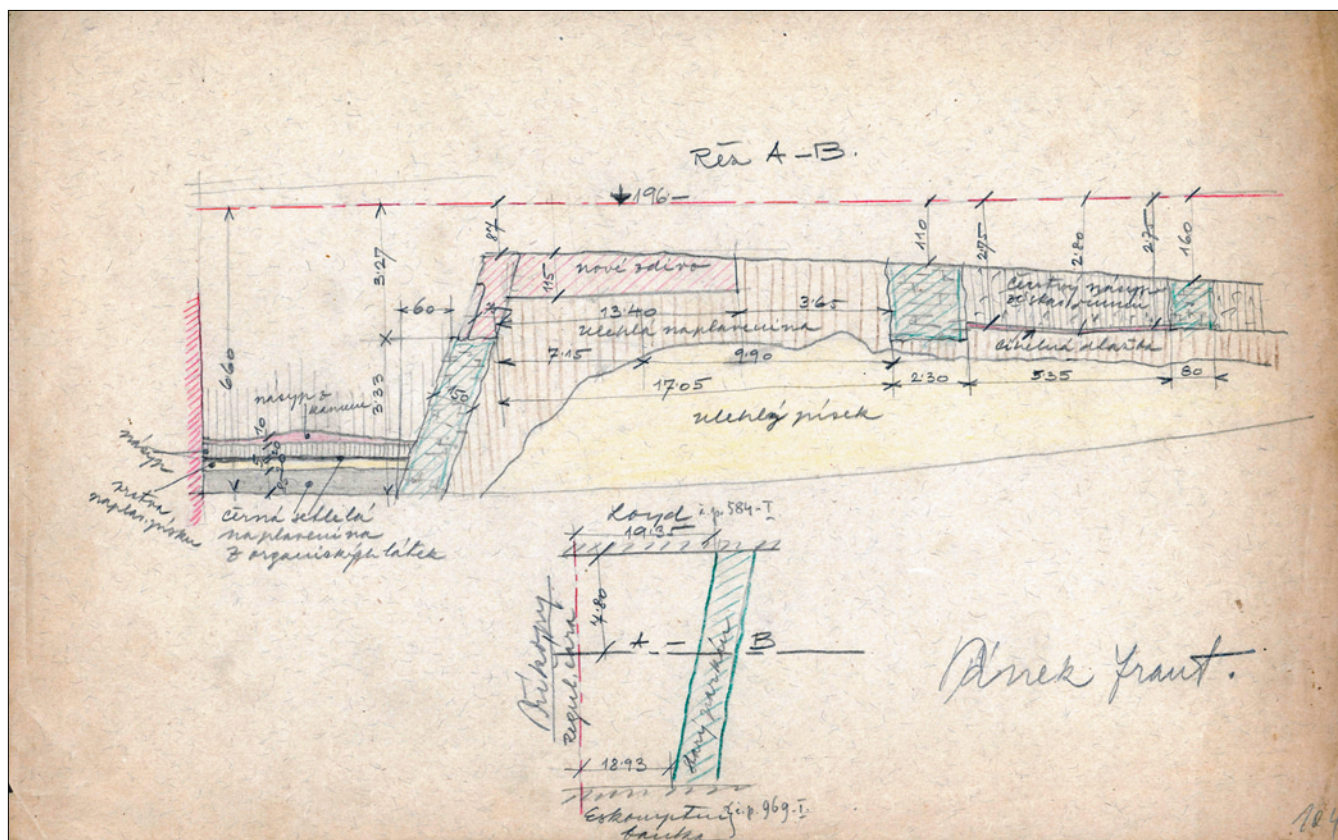
Obr. 18: SMP, výkopy pro stavbu pojišťovny Assicurazioni Generali v ulici Na Příkopě čp. 988/I s odkrytými pozůstatky opevnění. Příčný řez (kresba Fr. Pánek, 1938. ÚDU AV ČR, DSF, W-A-150/1-104).
