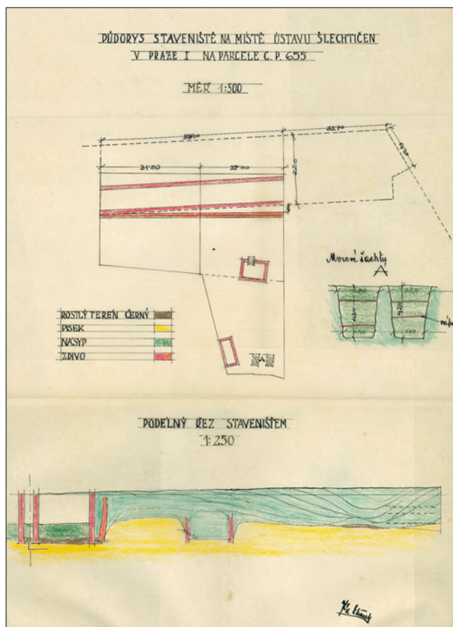
Obr. 13: SMP, výkopy pro stavbu obchodního domu čp. 655/I na místě bývalého premonstrátského semináře s odkrytými pozůstatky opevnění. Celková situace a příčný řez. Čárkované objekty semináře, plně základové stěny pod jeho západním traktem. Šikmo běžící zeď je vnitřní skarpa příkopu s parkánovou zdi (kresba K. Ptáček, 1928. ÚDU AV ČR, DSF, W-A-150/1-154).
