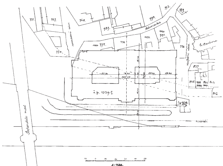
Obr. 6: SMP, situace s Ministerstvem obchodu čp. 1039/I se zakresleným průběhem opevnění (ÚDU AV ČR, DSF, W-A-150/1-109).
