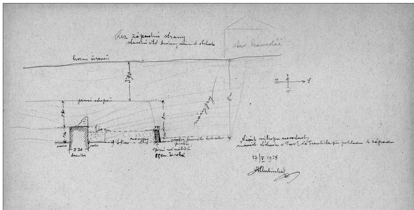
Obr. 5: SMP, výkopy pro stavbu Ministerstva obchodu čp. 1039/I s odkrytými pozůstatky opevnění. Skica příčného řezu v místě hlavní hradby a parkánu (kresba R. Hlubinka, 1928. ÚDU AV ČR, DSF, W-A-150/1-111).
