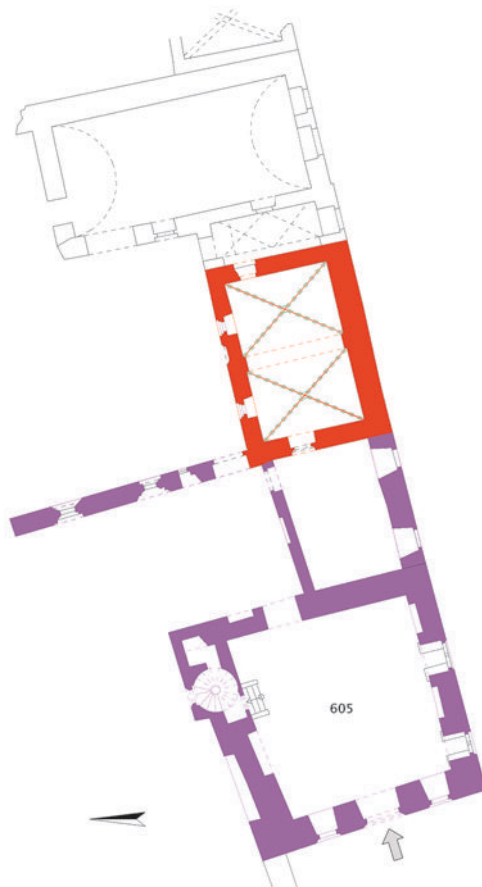
Obr. 28: Palác čp. 605. Schéma stavebního vývoje přízemí. Etapa 1230 až 1305 ■, po 1310 ■, (podklady autor, kresba P. Mourek).
