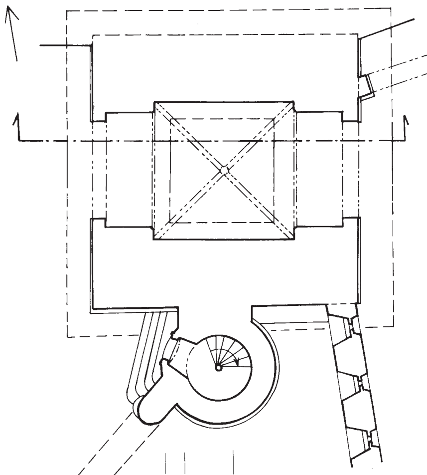
Obr. 2: Jičín, Valdická brána. Půdorys přízemí s vyznačením polohy měřeného profilu – silně čerchované – a půdorysu základů – čárkované (doplněno do upraveného podkladu P. Uličného).
