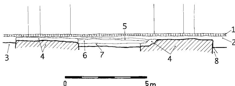
Obr. 1: Jičín, Valdická brána. Severní profil průkopu plynovodního potrubí. 1 – dlažba, 2 – písčité souvrství podkladu dlažby, 3 – žlutý písek, 4 – zdivo z lomových (nepravidelných) pískovcových kvádrů, 5 – šedá písčítá s rezavými a černými peckami, přecházející k východu v hnědošedou hlinitou, 6 – rezavý písek, 7 – hlinitopísčítá se zlomky pískovce, 8 – okrový jíl (pásmem a skládacím dvoumetrem zaměřil 21. května 1992 J. Slavík).
