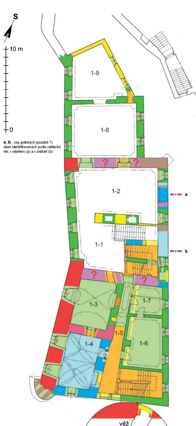
Obr. 7: Bečov nad Teplou, hrad, tzv. Pluhovské domy, stavební vývoj, 1. patro (autorova analýza s použitím plánového podkladu J. Čepeláka).
