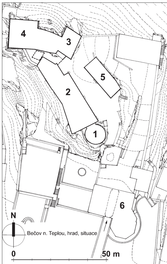
Obr. 2: Bečov nad Teplou, hrad a zámek, situace; 1 – věž, 2 – tzv. Pluhovské domy, 3 – kaplová věž, 4 – donjon, 5 – klasicistní stáje, 6 – zámek (upraveno podle podkladu J. Čepeláka).
