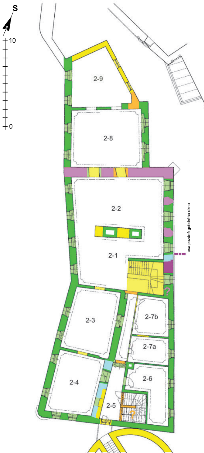
Obr. 8: Bečov nad Teplou, hrad, tzv. Pluhovské domy, stavební vývoj, 2. patro (autorova analýza s použitím plánového podkladu J. Čepeláka).
