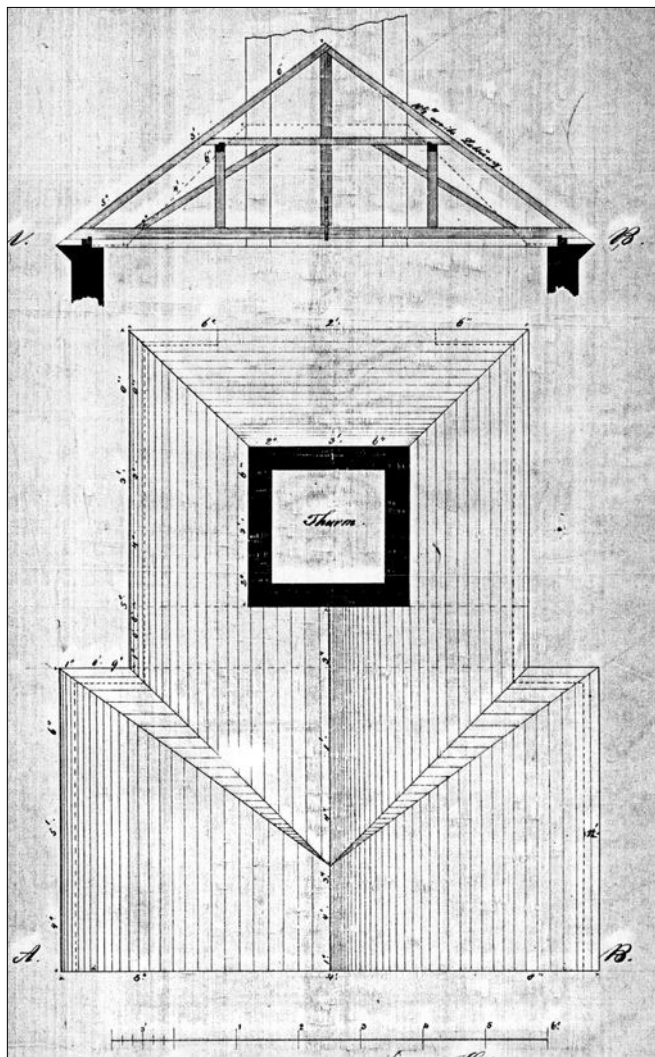
Obr. 5: Záboří nad Labem, kostel sv. Prokopa, plán na pokrytí střechy zábořského kostela taškami, řez, půdorys [E. Haller, asi 1852, SOA Praha].
