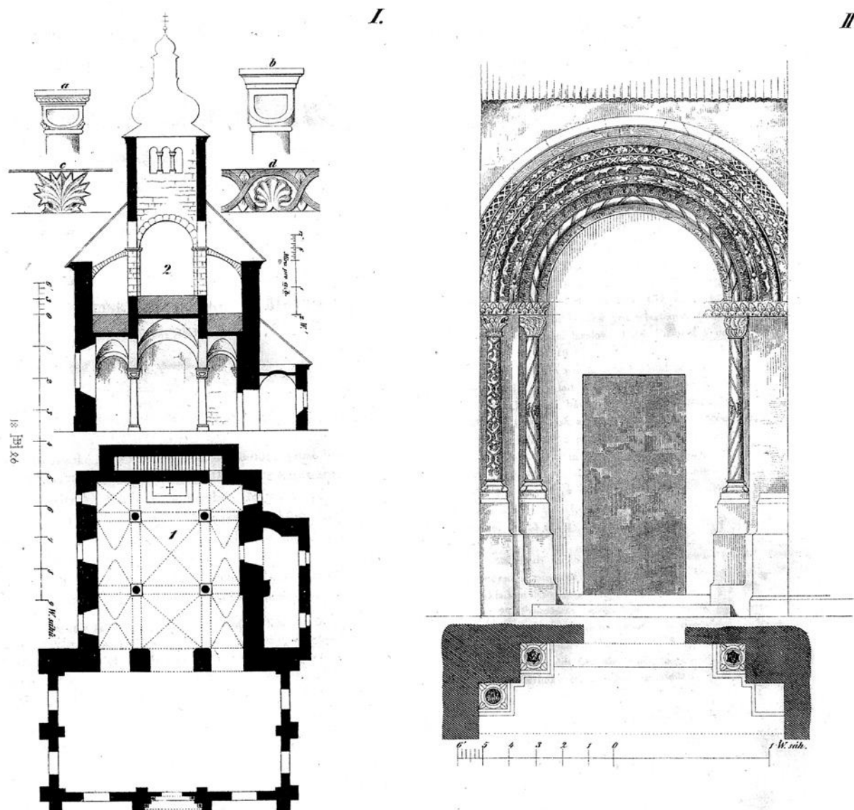
Obr. 2: Zábore nad Labem, kostel sv. Prokopa, půdorys, řez, detaily a portál kostela, 1846 (repro z: J. E. Vocel, o. c. v pozn. 1).
