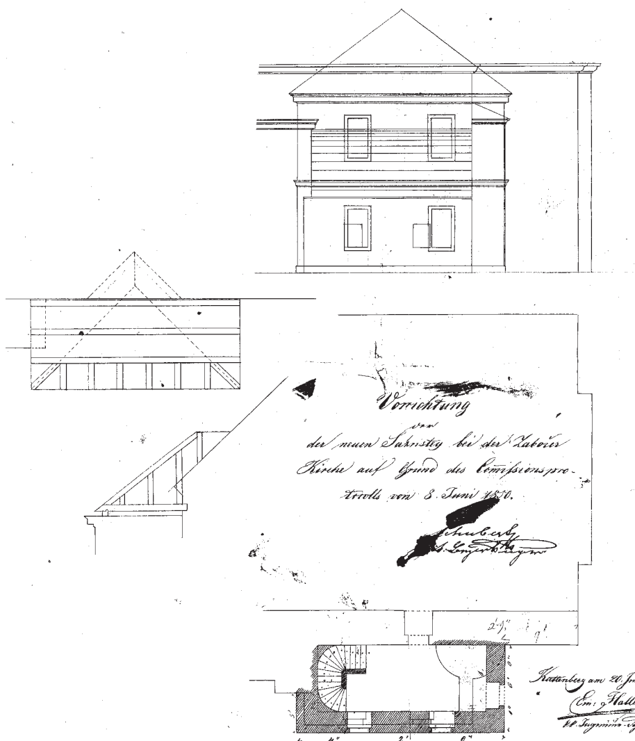
Obr. 4: Záboří nad Labem, kostel sv. Prokopa, plán na zřízení nové sakristie (E. Haller, 1850, SOA Praha).
