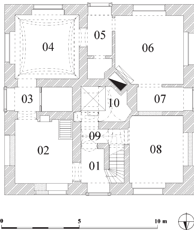
Obr. 5: Nákle, plán přízemí loveckého zámku, sestavený ze zaměření jednotlivých místností, provedeného v roce 1958 (originál uložen v Archivu Akademie věd ČR, kresba R. Vojvody).
