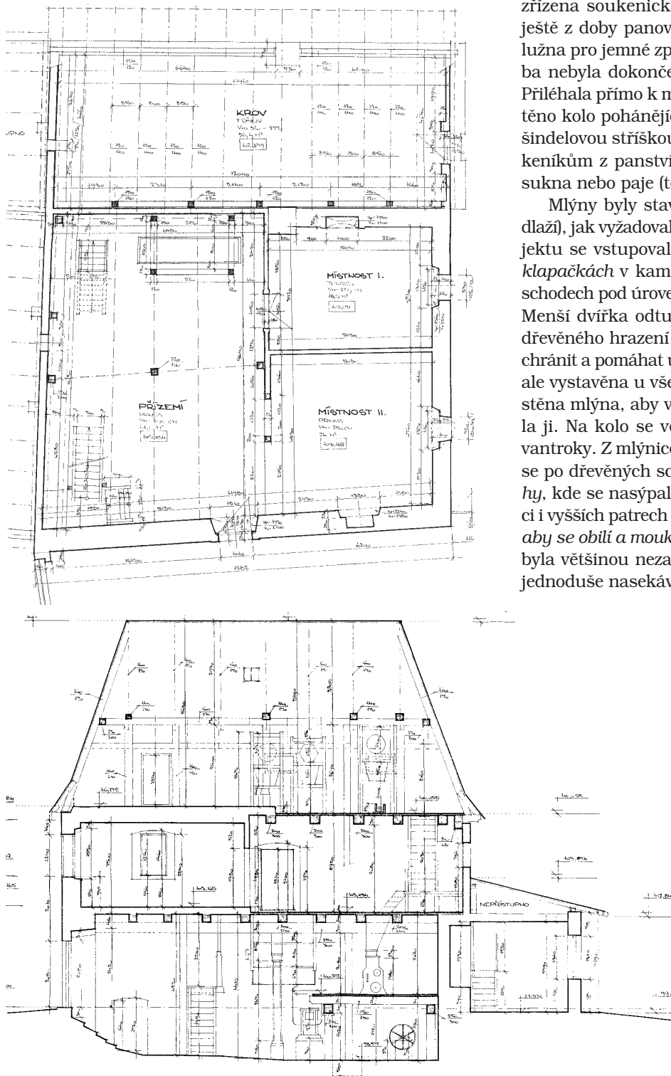
Obr. 40: Tismice (okres Kolín), mlýn, půdorys patra a podélný řez (zaměření M. Fuchs, 1991). Část konstrukcí mlýna byla roubená a hrázdná, zachovány byly pozoruhodné tesařské konstrukce. Budova si zřejmě do svého zániku v 90. letech 20. století zachovala mnohé z výstavby roku 1676 uváděné v urbáři. Popisu odpovídá zděné přízemí i částečně roubené patro, včetně rozdílných konstrukcí vymezujících světnici.
