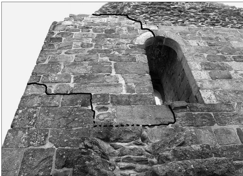
Obr. 35: Hrad Přimda, věž. Detail západního průčelí nad severní zdí rizalitu se vstupem do 1. patra věže. Čárou vymezeno novodobé zdivo (srov. obr. 5, 22; foto autor, 2008, k tisku upravil V. Tutr).
