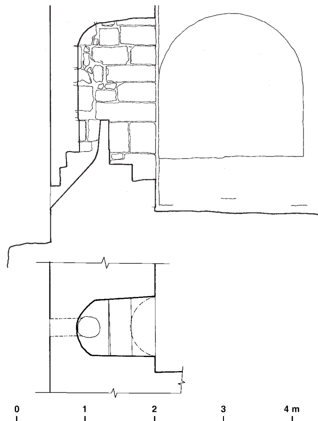
Obr. 30: Hrad Přimda, rizalit věže. Prevet v severní zdi, půdorys a svislý řez s pohledem k východu (zaměření Zv. Dragoun, 2008, k tisku upravili J. Veselý a V. Tutr).
