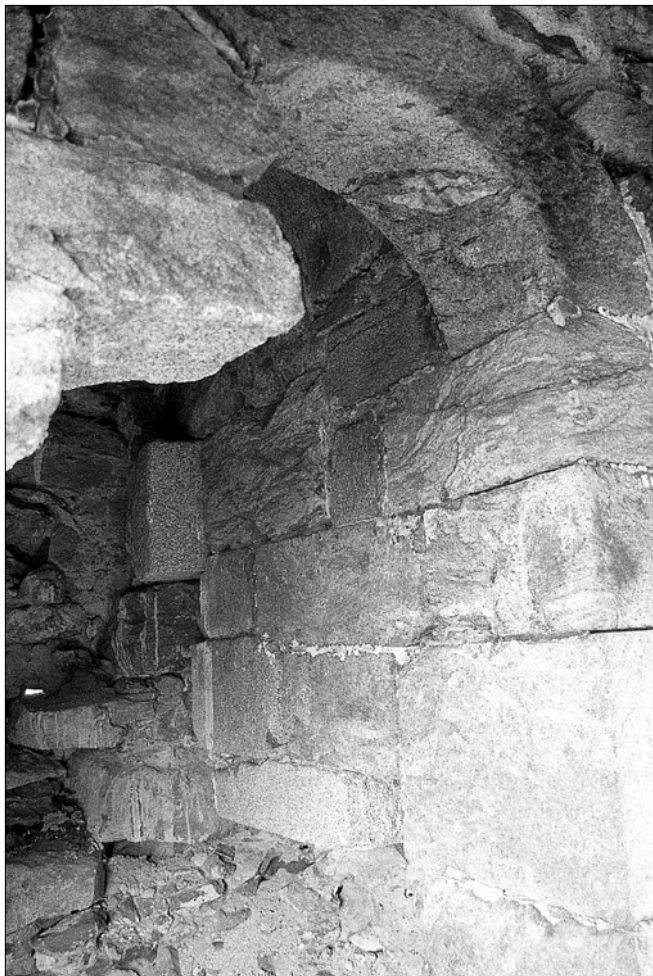
Obr. 23: Hrad Přimda, věž. Celkový pohled do prostoru chodby k prevétu (srov. obr. 18). Stav před vybráním záspy (?) v dolní části (foto autor, 2000).
