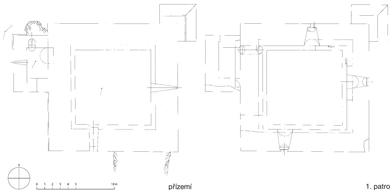
Obr. 10: Hrad Přimda, věž. Půdorys přízemí a 1. patra. Archiv NPÚ, J. Houžvíc, 1962 (nerevidováno; chodbička k předpokládanému prevetu v 1. patře není zakreslena, okénko v přízemí rizalitu nepůvodní).
