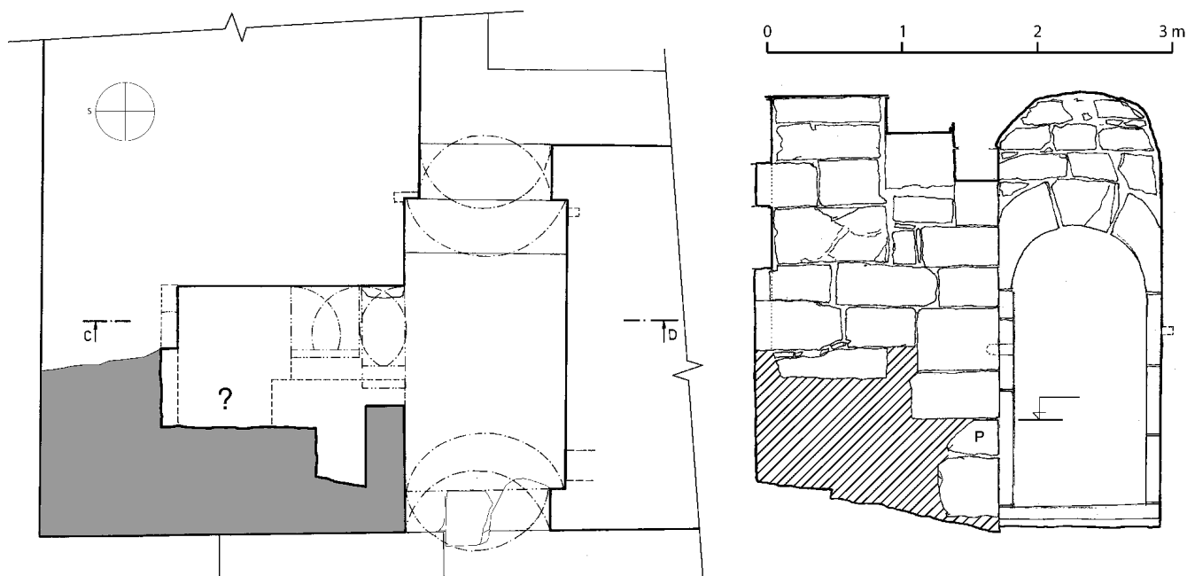
Obr. 22: Hrad Přimda, věž. Vlevo půdorys severozápadního nároží v úrovni 1. patra, s chodbou do rizalitu a dochovanou částí chodbičky k předpokládanému převětu. Sedou vyznačeno novodobé zdivo. Vpravo svislý řez s pohledem k východu (P – práh) (zaměření Zv. Dragoun, 2008, k tisku upravili J. Veselý a V. Tůtr).
