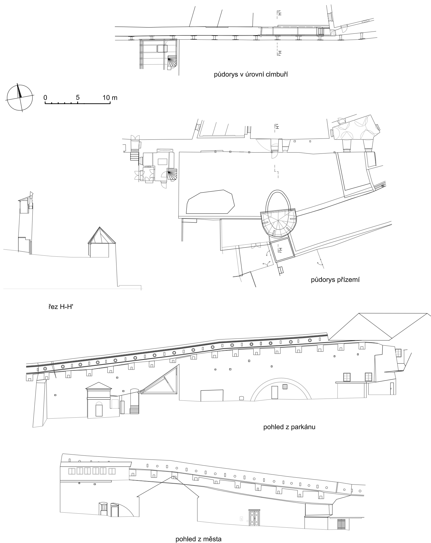
Obr. 29: Telč, zaměření části městských hradeb v jejich jižním oblouku (zaměření GEOMESS, v. o. s., 2007, k tisku upravil V. Tutr).
