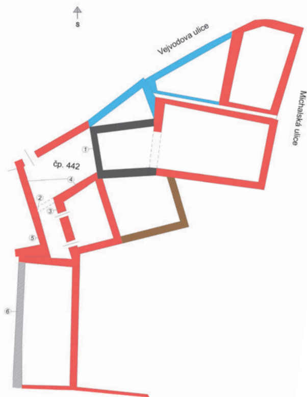
Obr. 3: Praha 1 – Staré Město, Vejvodova čp. 442. Schematický půdorys přízemí a sousedních objektů na základě zaměření SÚRPMO (četné nepravdivosti a nepřesnosti jsou dány nekvalitním zaměřením), doplněno, upraveno. Černě raně gotické konstrukce (bezpečně a předpokládané), červenou barvou předpokládané gotické konstrukce (s doplněnou gotickou uliční stěnou čp. 442), modře předpokládané a hypotetické renesanční konstrukce, hnědě základní barokní etapa. 1 – poloha raně gotické fasády v patře; 2 – technologická spára; 3 – ostění gotického portálu; 4 – místo konstrukcí s otisky vloženého dřevěného interiéru v patře; 5 – přibližná poloha zjištěných otisků dřevěného kuláče a dalších prvků v patře sousedního čp. 443; 6 – hloubková gotická dodatečně nadezděná zeď (upravil M. Kovář, překreslila H. Kovářová).
