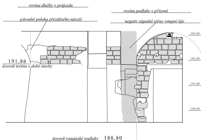
Obr. 6: Praha 1 - Staré Město, Celetná ulice čp. 558/I. Pohled od jihu na klenbové čelo vstupní šíje na vnějším lici jižní stěny místnosti 1 a na torzo tří dochovaných řádků jejího nadzemního zdiva (kresba M. Růžicka a M. Semerád).
