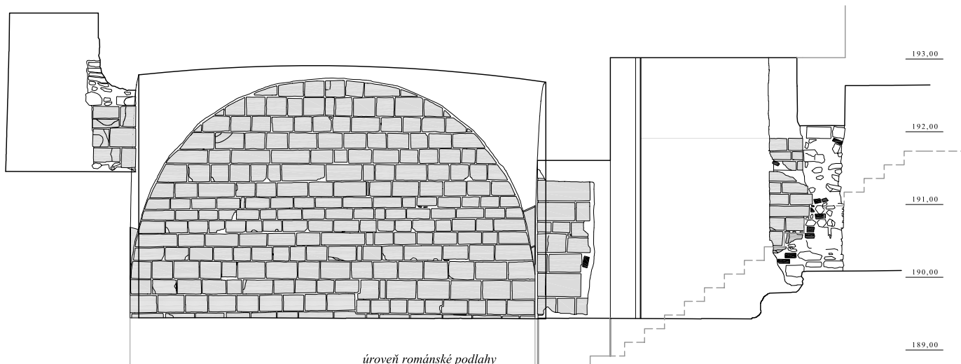
Obr. 4: Praha 1 - Staré Město, Celetná ulice čp. 558/I. Pohled od západu na východní stěnu místnosti 1, bok portálové niky a torzo východní stěny vstupní šije s rekonstrukcí vstupního schodiště (kresba M. Semerád).
