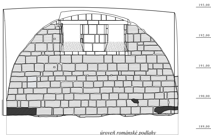
Obr. 5: Praha 1 - Staré Město, Celetná ulice čp. 558/I. Pohled od jihu na severní stěnu místnosti 1 s rekonstruovanou podobou dvojice oken (kresba J. Vachuda a M. Semerád).
