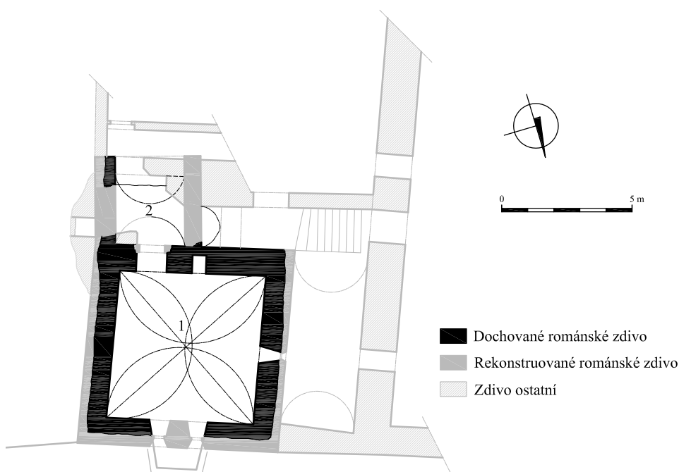
Obr. 2: Praha 1-Staré Město, Celetná ulice čp. 558/I. Půdorysná situace spodního podlaží románského domu, 1 - hlavní prostora, 2 - vstupní šije (kresba M. Semerád).
