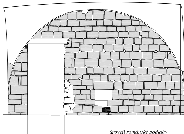
Obr. 3: Praha 1 - Staré Město, Celetná ulice čp. 558/I. Pohled od severu na jižní stěnu místnosti 1 s pozůstatky portálové niky a s odkládací nikou (kresba M. Růžička a M. Semerád).
