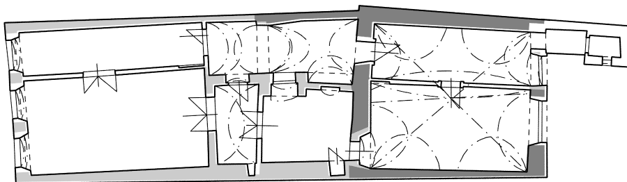
Obr. 9: Jihlava, dům čp. 1320. Půdorys 1. patra s vyznačením stavebních fází. Tmavě šedě vyznačeno zdivo hypoteticky středověké, světle šedě zdivo renesanční (pravděpodobně kolem 1576), šrafované konstrukce barokní (snad konec 17. století).
