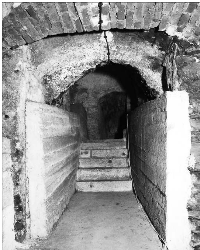
Obr. 11: Jihlava, dům čp. 1320. Přední sklep. Vstupní šje s blokem staršího ostění na západní (levé) straně v ústí šje do sklepa (všechny snímky P. Borský, 2005).
