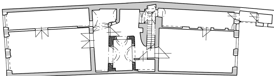
Obr. 10: Jihlava, dům čp. 1320. Půdorys 2. patra s vyznačením stavebních fází. Tmavě šedě vyznačeno zdivo hypoteticky středověké, světle šedě zdivo renesanční (pravděpodobně kolem 1576), šrafované konstrukce barokní (snad konec 17. století).
