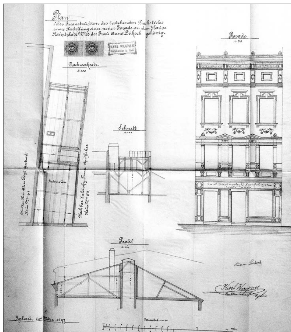
Obr. 5: Jihlava, dům čp. 1320. Realizovaný projekt nové hlavní fasády a krovu nad přední částí domu od městského stavitele Karla Wagnera z března 1897 (SOKA Jihlava, AmJ – Městská správa od roku 1849, Archiv Stavebního úřadu, čp. 1320).
