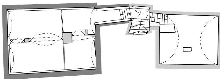
Obr. 7: Jihlava, dům čp. 1320. Půdorys sklepů s vyznačením stavebních fází. Tmavě šedě vyznačeno zdivo hypoteticky středověké, světle šedě zdivo renesanční (pravděpodobně kolem 1576), šrafované konstrukce barokní (snad konec 17. století). Stav před novodobou rekonstrukcí podle zaměření Stavo-projektu Jihlava z roku 1987 (úprava a digitalizace L. Sedláčková, 2010).
