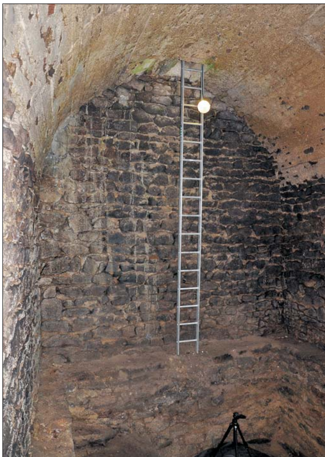
Obr. 28: Landštejn. Spodní podlaží severní věže, celkový pohled interiérem směrem k západu. Dole nepravidelně předstupující základová část, nad neomítnutými stěnami valená klenba s výraznými otisky bednění. Žebřík spojuje korunu základové části s otvorem v klenbě (foto autor, 2011).
