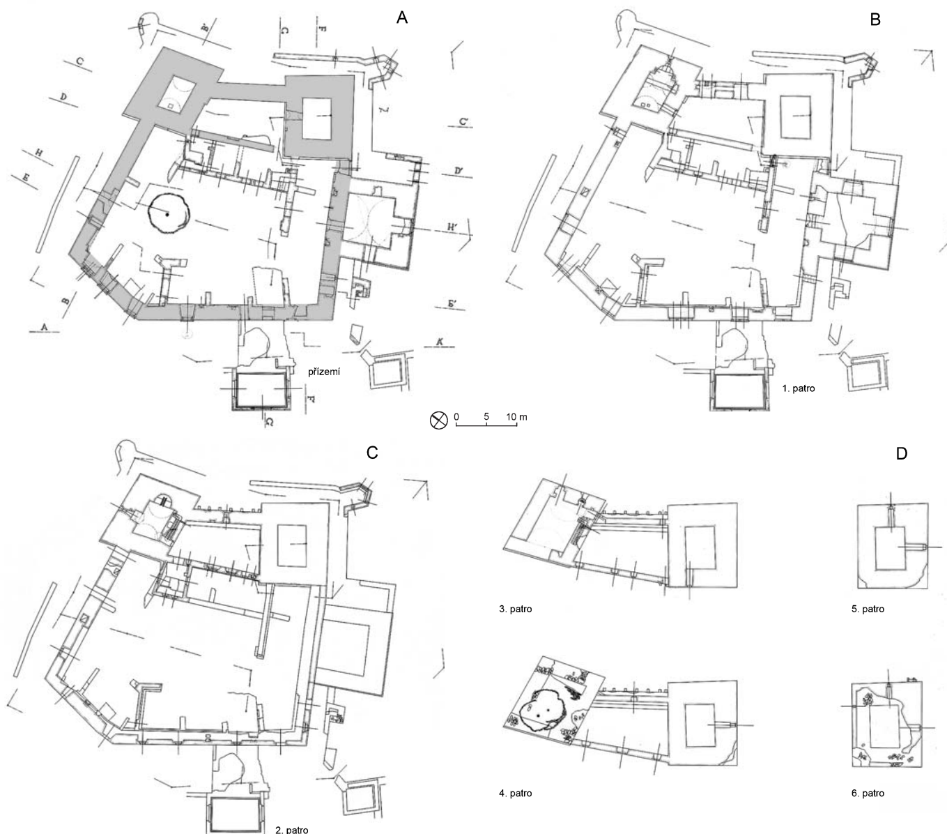
Obr. 15: Landštejn. Výběr ze zaměření jádra hradu z roku 1957. A – půdorys přízemí (šedě zvýrazněny prokazatelné části románské stavební fáze), B – půdorys 1. patra, C – půdorys 2. patra, D – půdorys horních pater věží a paláce, 1 – pohled od severu, 2 – pohled od východu, 3 – pohled od jihu, 4 – řez severní věží s pohledem k severu, 5 – řez jižní věží s pohledem k jihu (zaměření ing. Drápal a kol., fotokopie z NPÚ ÚP, k tisku upravil L. Bezděk a V. Tutr).
