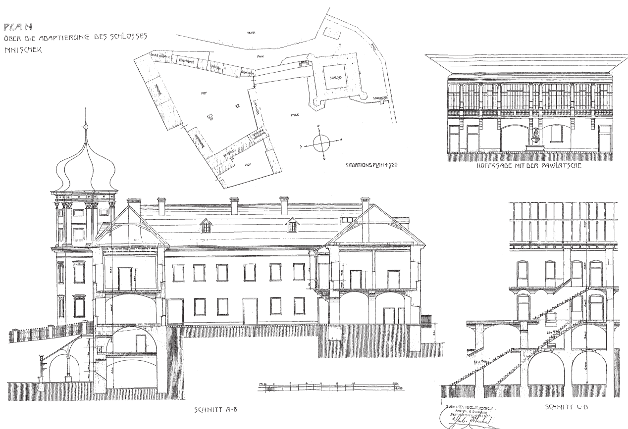
Obr. 5: Mníšek pod Brdy, zámek, plán adaptace zámku (bez data, Mat. Blecha, 1 : 100 – SOA Praha, Vs Mníšek, kart. 111).
