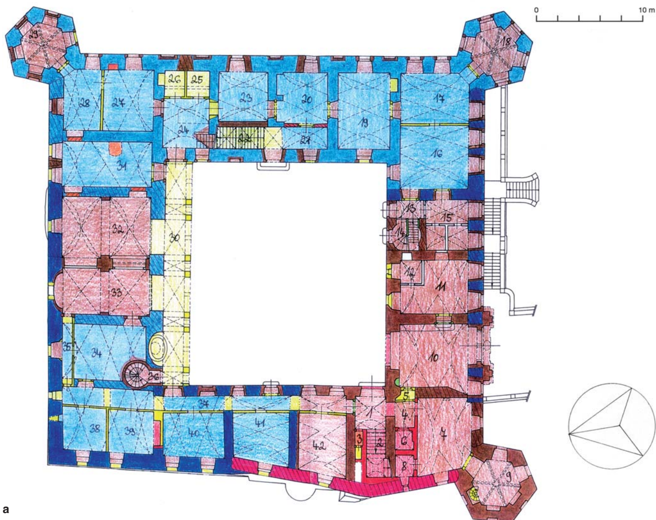
Obr. 7: Mníšek pod Brdy, zámek, půdorysy: a – přízemí; b – prvního patra (vyhodnocení P. Macek, 2001).
