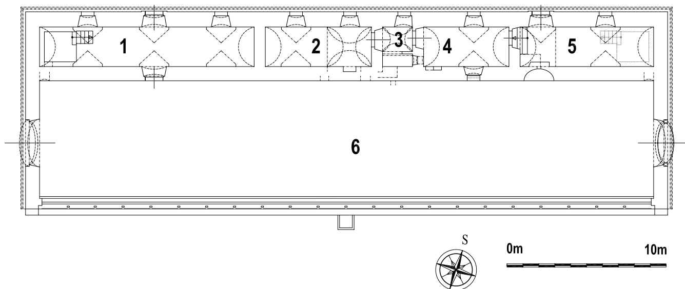
Obr. 26: Krásný Dvůr, půdorys současného stavu oranžerie postavené v roce 1812. Část prostorů v obslužném traktu sloužila zčásti jako byt hlídače (prostor 2 – kuchyň, 3 a 4). Prostor 1 a 5 mohl sloužit jako kolna pro skladování dřeva a nářadí a zároveň se z jejich konců, tam kde jsou schody, vytápěl kanál, který rozváděl teplo do hlavní části určené k pěstování citrusů a exotických rostlin (prostor 6). (zaměření provedl autor příspěvku spolu s L. Chotěborskou v roce 2009, kresba L. Chotěborská).
