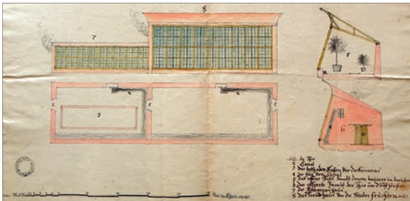
Obr. 25: Krásný Dvůr, plán, řez, jinde zvané jako skleník pro ananasy. Čelní pohled, půdorys, řez a boční pohled. K jednotlivým částem stavby jsou přiřazeny číslice, které jsou popsány ve vysvětlivkách (viz. pozn. 46). Plán je o velikosti 29 × 44 cm, kolorován, v levém dolním rohu je měřítko v loktech (SOA Třeboň, pobočka Jindřichův Hradec, Velkostatek Krásný Dvůr, kart. 150, sign. VI. G alfa).
