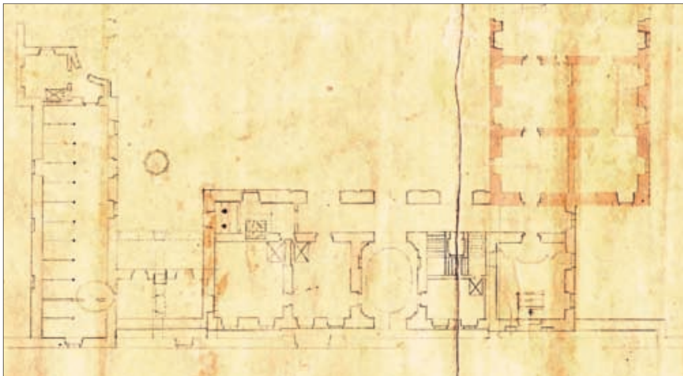
Obr. 3: Krásný Dvůr, detail přízemí východního křídla zámku se zakreslením starších konstrukcí. Na plánu je zakreslena novostavba patrového křídla s napojením na starší budovu zámku. V dolní části vidíme průběh staré ohradní zdi i se zakreslením budovy staré vrátnice v místech před příčným křídlem stájí. Příčné křídlo pochází z první fáze Kaňkova návrhu a mělo být zakončeno světničkou pro vrátného. Křídlo bylo v průběhu výstavby, po změně projektu, ubouráno na dnešní úroveň. Na plánu je také v krajní severní místnosti dobře vidět kaple a na opačném konci „byt oficíra“. Při pozorném pohledu lze rozpoznat i prostor altánu s dvojicí otevřených arkád, který překrývá starší konstrukce vrátnice (celkový plán je uložen SOA Třeboň, pobočka Jindřichův Hradec, Vs Krásný Dvůr, kart. 138, sign. VI. B beta.).
