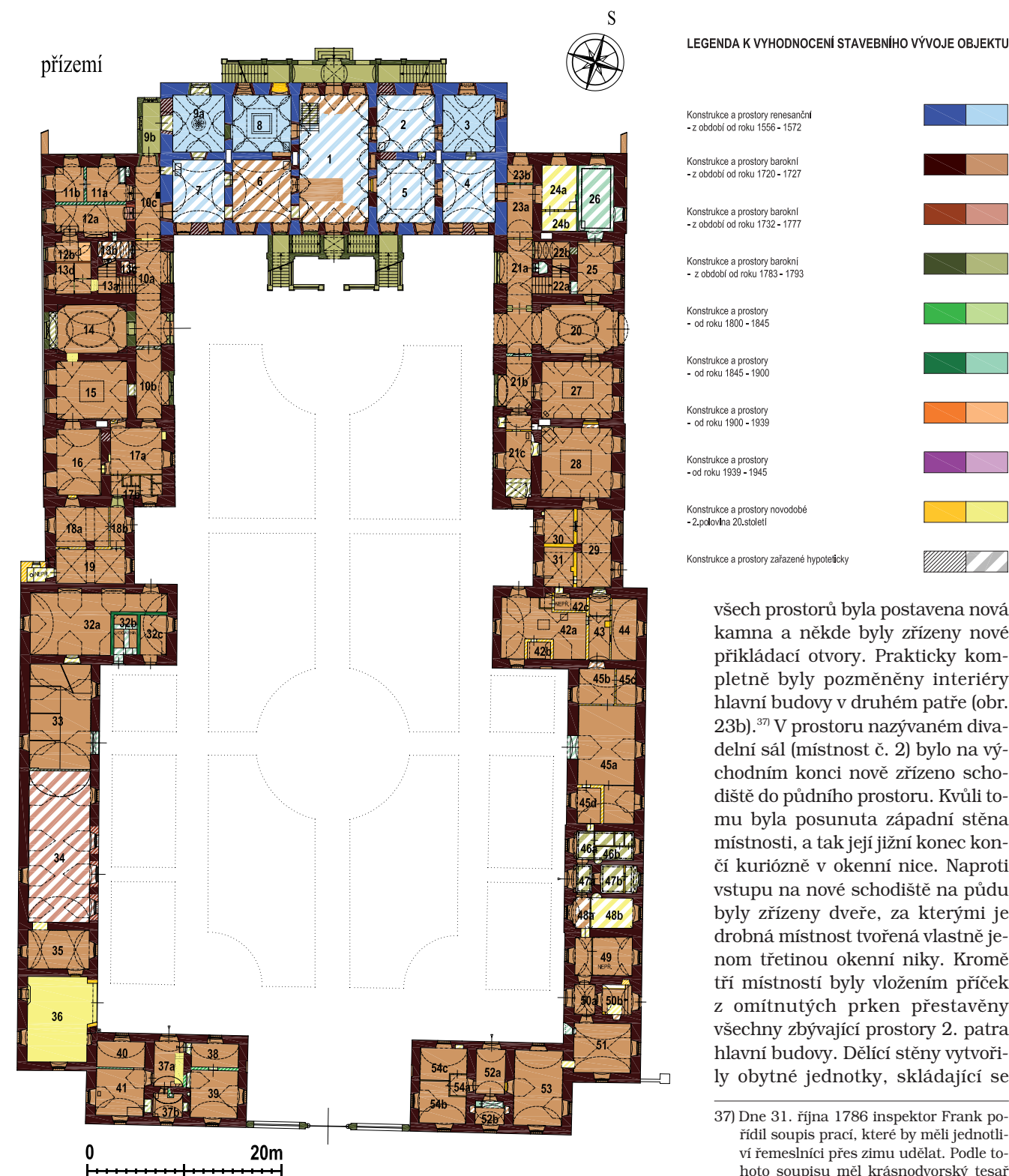
Obr. 22: Krásný Dvůr, zaměření současného stavu, půdorys přízemí se zakreslením stavebního vývoje. Na plánu vidíme hlavní budovu s převážnou většinou před barokních konstrukcí, ke kterým v letech 1783–1793 přibyla dvojice venkovních schodišť. Do prostoru 9a byla přenesena kaple, která byla umístěna v prostorech 23a, b, 24a, b, a 26. Do prostoru 12b byl vestavěn kotel, který vhněl teplý vzduch do 8 prostorů na zámku. Další úpravy pochází již většinou z 2. pol. 20. stol. (kresba L. Chotěborská).
