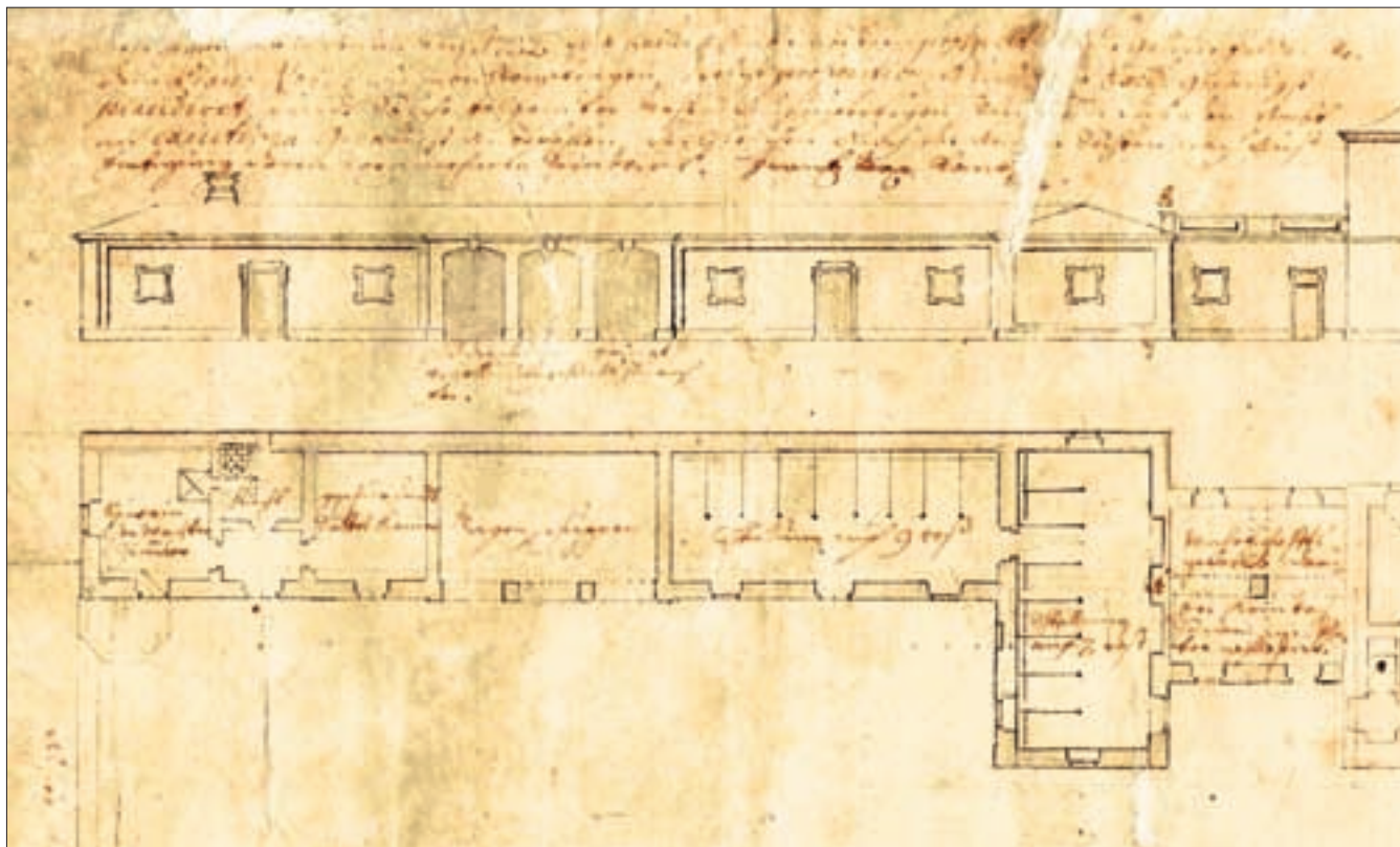
Obr. 5: Krásný Dvůr, detail přízemí západního křídla zámku se zakreslením starších konstrukcí a pohledem na fasádu. Přízemní západní prodloužené křídlo bylo zakresleno do plánu až po změně projektu na jaře 1722. K této změně se vztahuje text v horní části i v půdorysu. Při jižním konci je opět vidět zakončení staré ohradní zdi osmibokým stavením (celkový plán, je uložen SOA Třeboň, pobočka Jindřichův Hradec, Vs Krásný Dvůr, kart. 138, sign. VI. B beta.).
