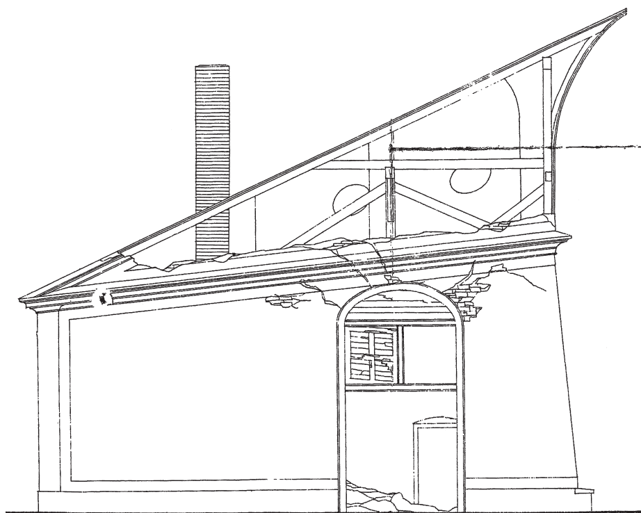
Obr. 28: Krásný Dvůr, oranžerie, pohled na západní fasádu. Zaměření z roku 1956 zachycuje objekt po částečném zřícení interiéru. Nicméně stála ještě střecha s mohutnou fabionovou římsou, která byla později beze zbytku odstraněna (plán je uložen pod označením Krásný Dvůr, zámek – skleník, zaměření stávajícího stavu, 1956. NPÚ Ústí nad Labem, archiv plánů).
