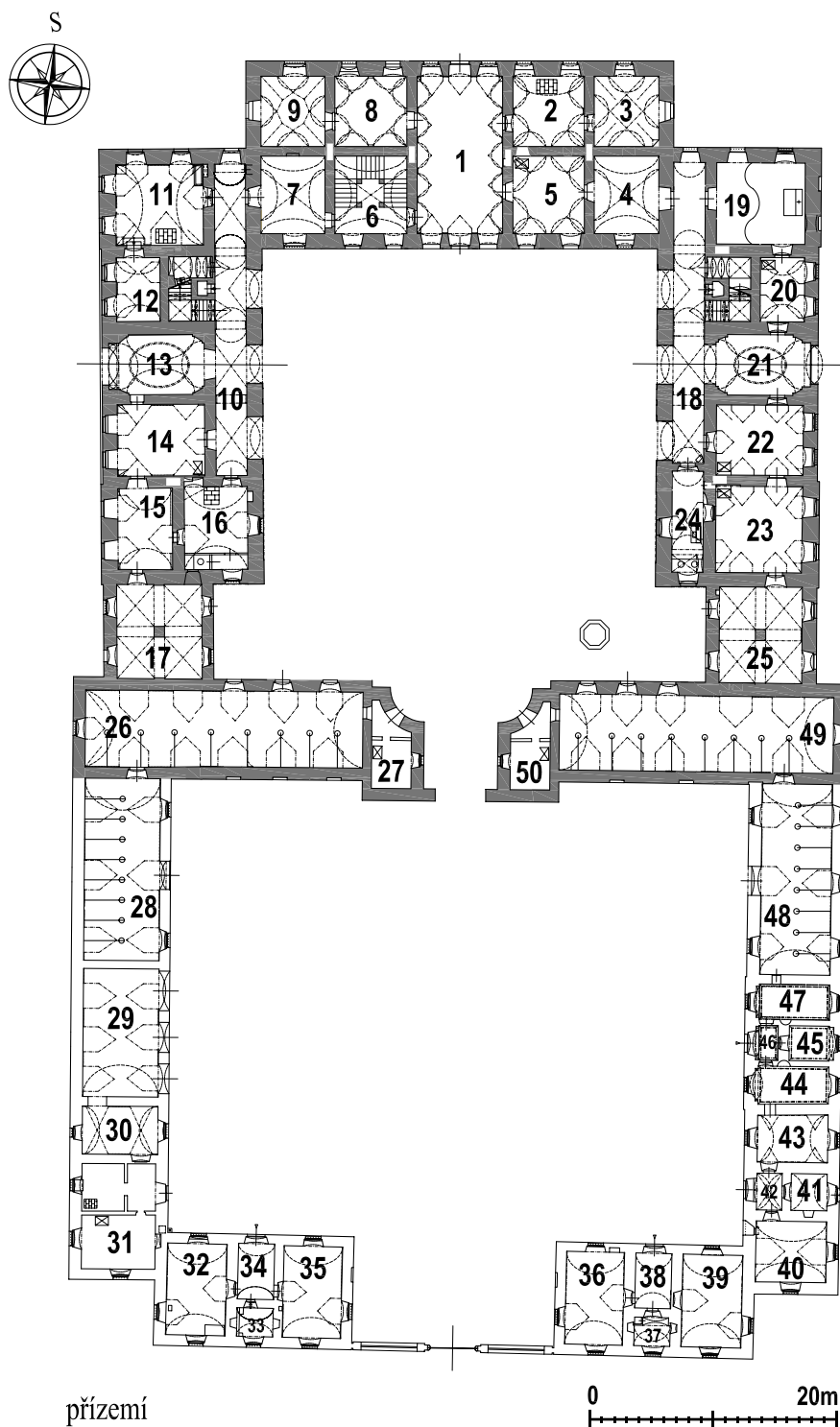
Obr. 16: Krásný Dvůr, půdorys přízemí, předpokládaná podoba v roce 1733 zobrazená spolu s původními příčnými křídly stájí. Rekonstruované rozmístění jednotlivých funkcí podle inventáře z téhož roku: prostor 1 – „stara kancelář“, 2 – „červený“ pokoj, 3 – „zelený“ pokoj, 4 – modře vymalovaný pokoj, 5 – štolbův pokoj, 6 – schodiště spojující všechna podlaží, 7 – pokoj (byť klíčnice? šaty ke komediím?), 8 – pokoj (byť klíčnice? šaty ke komediím?), 9 – (byť klíčnice? šaty ke komediím? pod správou purkrabího?), 11, 12 – kuchyň s prádelnou, 13 – průjezd, 14 až 17 – pod správou purkrabího a kontribučenského písaře, 19 – kaple, 20 – pokoj duchovního, 21 – průjezd, 22 – vedlejší pokoj, 23 a 24 – oficířský pokoj, 25 – kvelb, 26 – stáje pro 9 koní, 27 – světnička vrátného, 28 – stáje pro 7 koní, 29 – kůlna na vozy, 30 – komora na sedla a postroje pro koně, 31 – byt vrátného (prádelna?), 32 až 35 – byt vrátného, 36 až 39 – byt nočního hlídače, 40 až 43 – byt, 44 až 47 – byt, 48 – stáj pro 7 koní, 49 – stáj pro 9 koní, 50 – světnička nočního hlídače. Inventář z roku 1777: 2 a 3 – cukrárna, 4 – oficířský pokoj, 5, 9, 8 – pokoje, 7 – kvelb na ryby a vitkuálie, 11 – panská kuchyň, 12 – kuchyňský kvelb, 14, 15, 16, 17 – byt důchodního, 19 a 20 – kaple a sakristie (s oltářním obrazem sv. Huberta) 22 až 25 – pokoje, 40 – prádelna? 41 až 43 – u nabíječů pušek. Inventář z roku 1845: 2 a 3 – cukrárna s komorou, 7, 11, 12 – kuchyň, spíš a kvelb, 14 až 16 – kancelář s bytem důchodního, 17 – čeledník?, 19 – kaple, 20 – oratoř, 22 až 25 – obydlí správce, 32 až 35 – sluha, 36 až 39 – vrátný.
