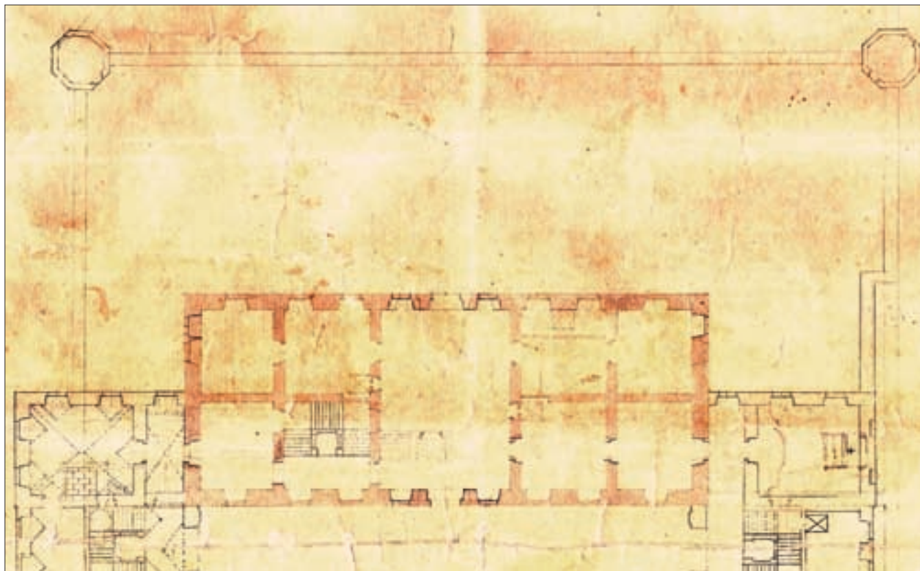
Obr. 2: Krásný Dvůr, detail přízemí hlavní budovy zámku se zakreslením starších konstrukcí. V horní části vidíme starou „renesanční“ ohradní zeď původního areálu s dvojicí osmibokých staveb. Hlavní budova je zvýrazněna tmavší barvou. Ve vstupní síni je vidět situaci staršího schodiště, po levé straně je schodiště nové, navržené Kaňkou. V místnosti severovýchodně od sálu je zachycena kuchyň. Na plánu jsou vidět posunutá vstupy i okna. Nesignovaný a nedatovaný plán pochází nejspíše z roku 1718, starší konstrukce zachytil zednický polír Václav Pinter, ostatní pocházejí od F. M. Kaňky, včetně psaného textu. Vzhledem k rozměrům (92 x 55,5 cm) a lepší čitelnosti zde plán prezentujeme po částech. (Celkový plán je uložen SOA Třeboň, pobočka Jindřichův Hradec, Vs Krásný Dvůr, kart. 138, sign. VI. B beta.).
