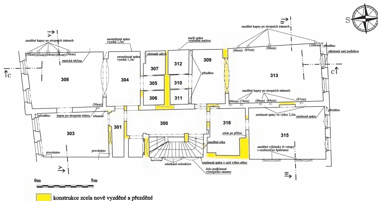
Obr. 6: Hradec Králové, Velké náměstí, dům čp. 41. Půdorys 2. patra s vyznačením nálezoových situací. Žlutě je vyznačeno zdivo z nynějších úprav.
