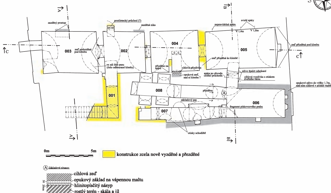
Obr. 4: Hradec Králové, Velké náměstí, dům čp. 41. Půdorys suterénu s vyznačením nálezových situací. Žlutě je vyznačeno zdivo z nynějších úprav.
