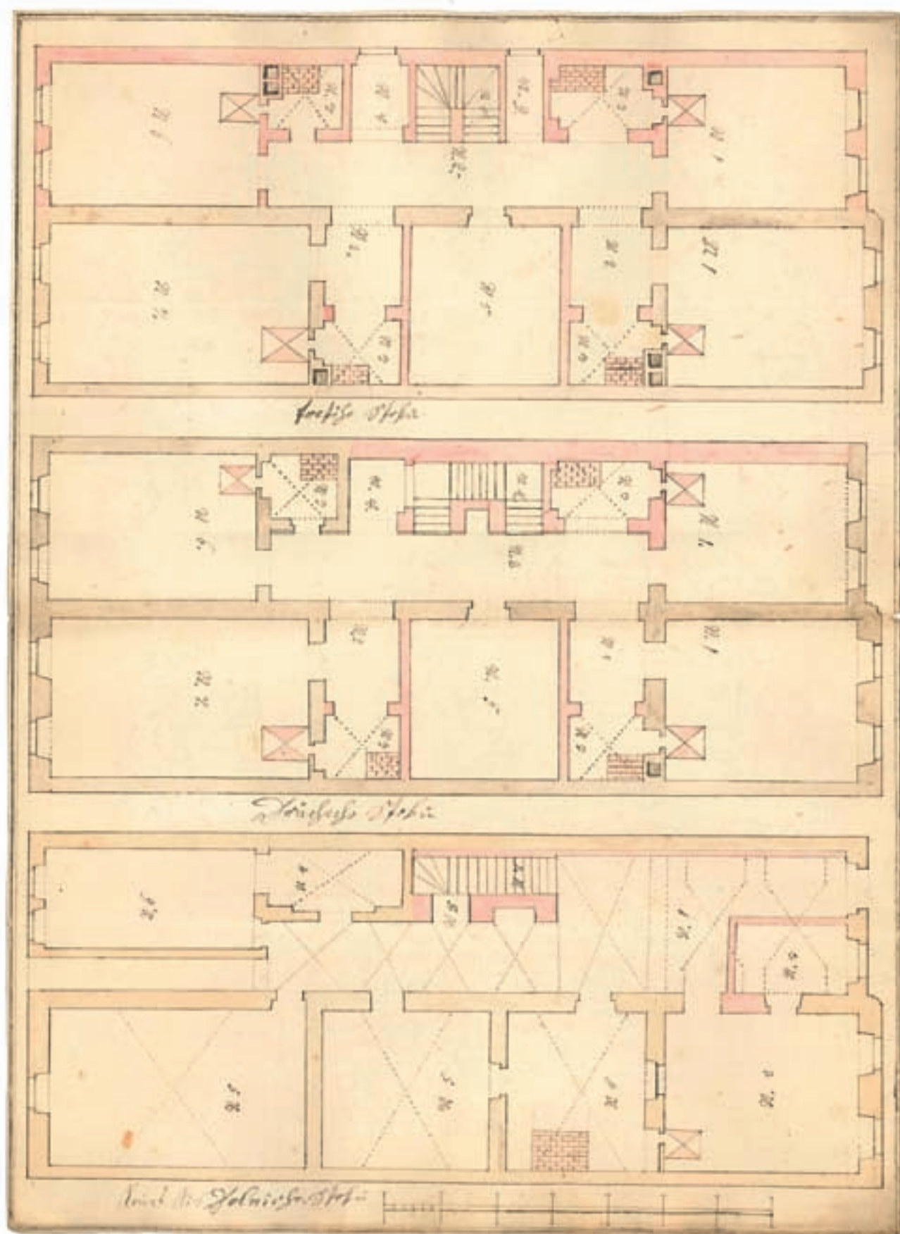
Obr. 16: Hradec Králové, Velké náměstí, dům čp. 41. Plán z počátku 19. století, půdorys. Popis místností (bez úpravy pravopisu): Poznamenání numer (v) dolním štok: N 1 – Foršház, N 2 – Přední pokoj, N 4 – Kuchyně, N 5 – Kvelbi, N 6 – Dílna perníkářská, N 7 – Do prvního štoky schody, N 8 – Do sklepa schody. Poznamenání první(ho) štoky: N 1 – do předu pokoje, N 2 – forcház, N 3 – Kuchyně, N 4 – schody do druhého štoky, N 5 – komora, N 6 a 7 – dozadu pokoje, N 8 – světlík. Poznamenání (v) druhém štok: N 1 – do předu pokoje, N 2 – forcház, N 3 – kuchyně, N 4 – na půdu schody, N 5 – komora, N 6 a 7 – zadní pokoje, N 8 a 9 – světlíky. (Státní okresní archiv Hradec Králové, Archiv města Hradce králové, inv. č. 5135, fasc. 12., Anonym, nedatováno).
