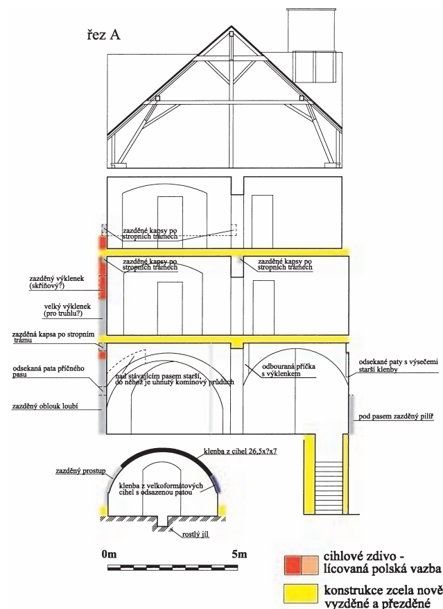
Obr. 8: Hradec Králové, Velké náměstí, dům čp. 41. Příčný řez s vyznačením náleзовých situací. Žlutě jsou vyznačeny novodobé konstrukce, oranžově lícované cihlové zdivo v polské vazbě.
