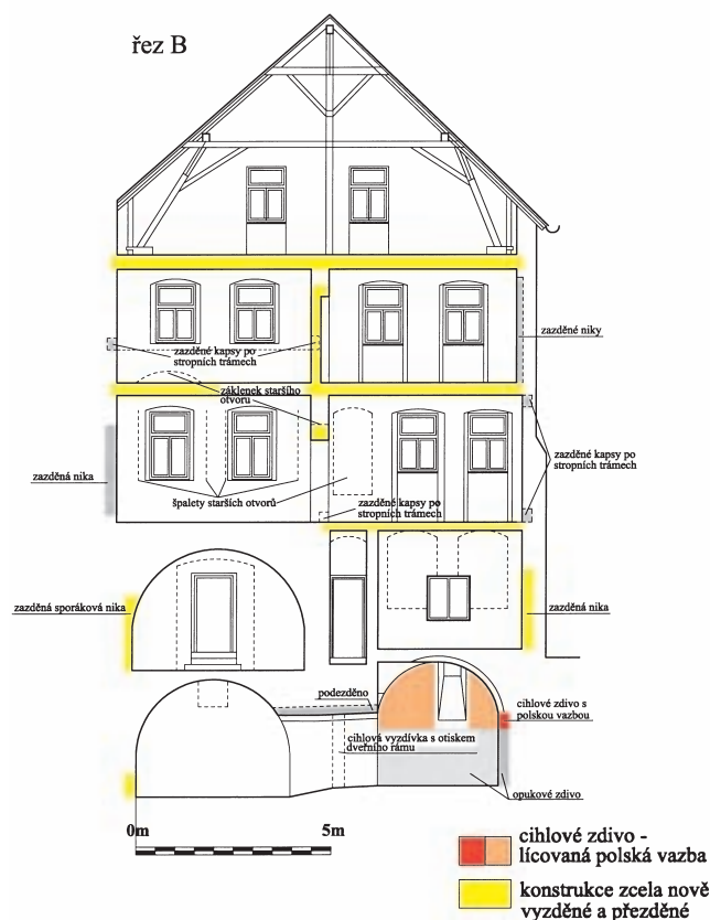
Obr. 9: Hradec Králové, Velké náměstí, dům čp. 41. Příčný řez s vyznačením náleзовých situací. Žlutě jsou vyznačeny novodobé konstrukce, oranžově lícované cihlové zdivo v polské vazbě.
