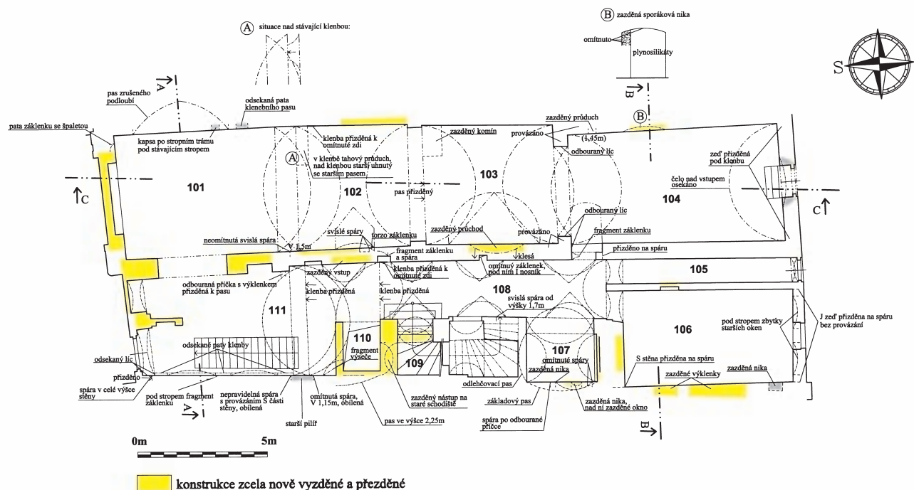
Obr. 3: Hradec Králové, Velké náměstí, dům čp. 41. Půdorys přízemí s vyznačením náleзовých situací. Žlutě je vyznačeno zdivo z nynějších úprav (jakou podklad výkresové dokumentace byl použit Projekt změny stavby před dokončením – Ing. Oldřich Drahorád – DUO projekt, 2010, grafické zpracování Miloš Buroň, platí také pro obr. 4–9).
