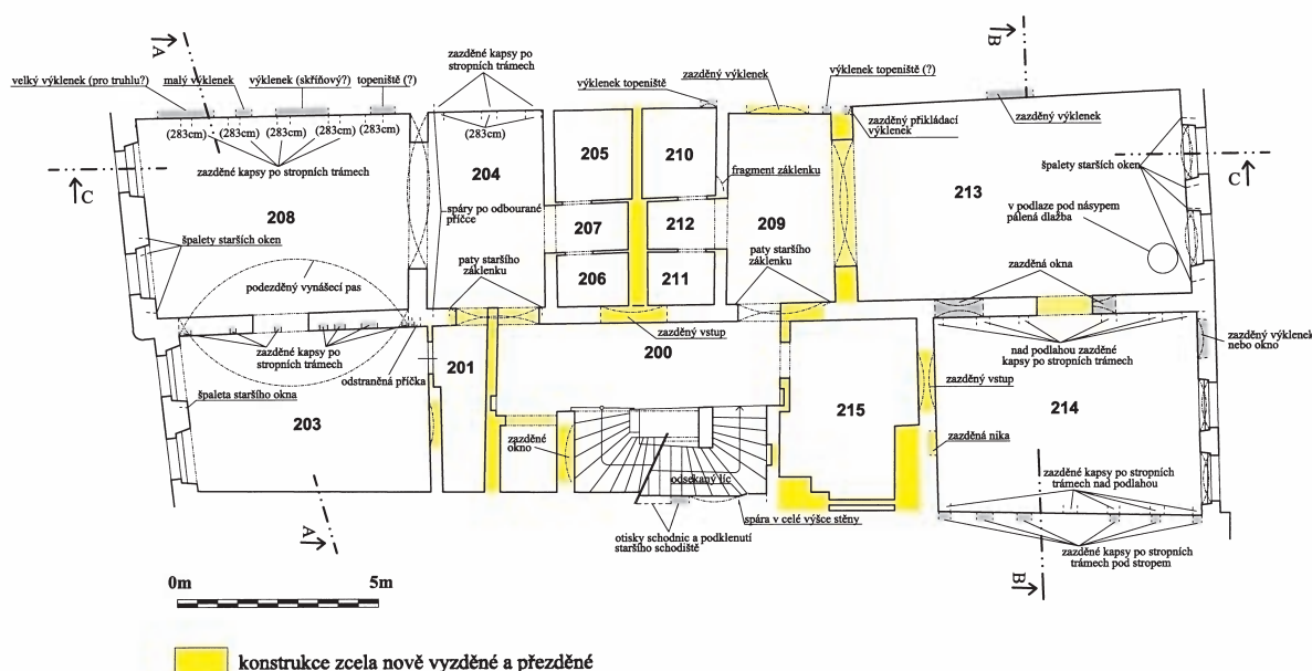
Obr. 5: Hradec Králové, Velké náměstí, dům čp. 41. Půdorys 1. patra s vyznačením náleзовých situací. Žlutě je vyznačeno zdivo z nynějších úprav.
