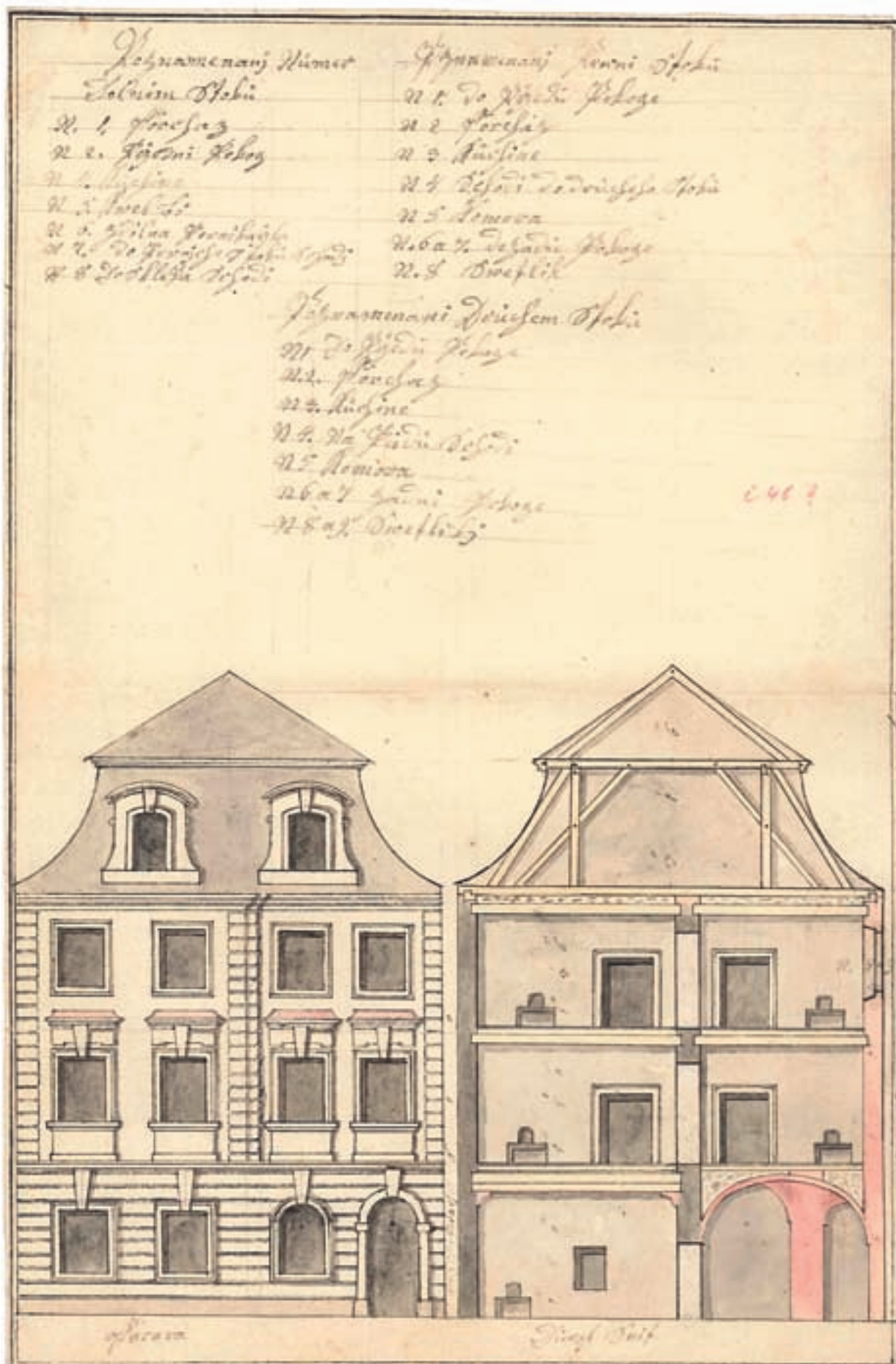
Obr. 17: Hradec Králové, Velké náměstí, dům čp. 41. Plán z počátku 19. století – příčný řez. (Státní okresní archiv Hradec Králové, Archiv města Hradce Králové, inv. č. 5135, fasc. 12., Anonym, nedatováno).
