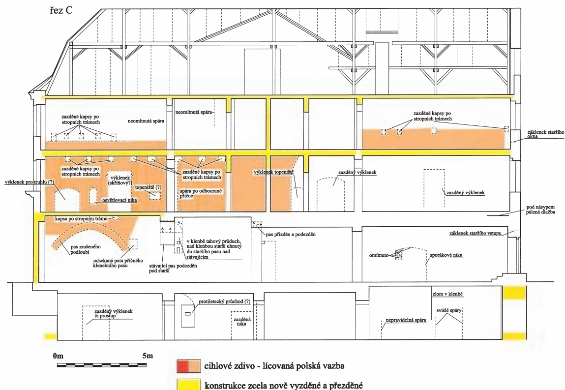
Obr. 7: Hradec Králové, Velké náměstí, dům čp. 41. Podélný řez východním traktem s pohledem k východu s vyznačením náleзовých situací. Žlutě jsou vyznačeny novodobé konstrukce, oranžově lícované cihlové zdivo v polské vazbě.
