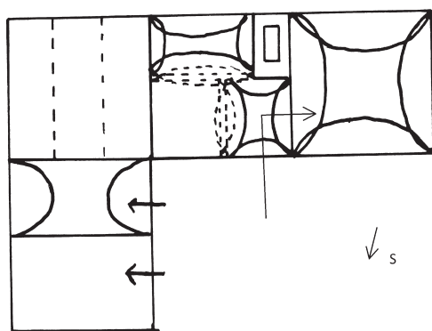
Obr. 20: Sedlec, čárové schéma půdorysu domu čp. 20, kresleno bez měřítka.
