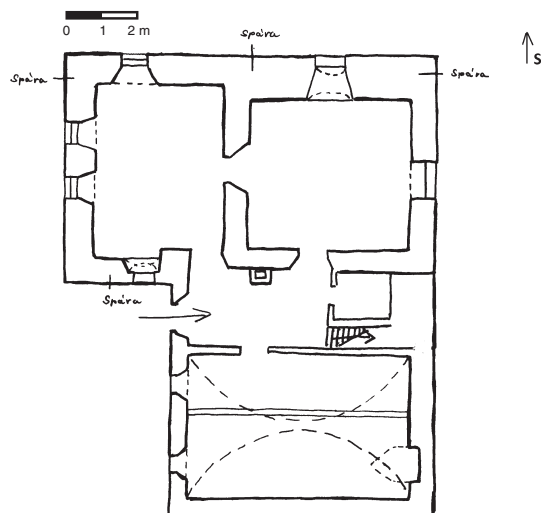
Obr. 15: Sedlec, čárové schéma půdorysu přízemí a patra domu v usedlosti čp. 6.
