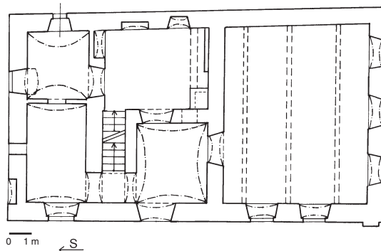
Obr. 18: Sedlec, půdorys domu v usedlosti čp. 14 (zaměření J. Švec, Z. Vařeková)
