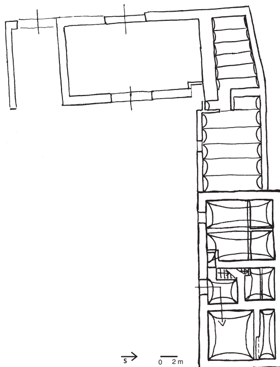
Obr. 11: Sedlec, čárové schéma půdorysu usedlosti čp. 5 s vyznačením stropních konstrukcí. (Z. Vařeková)
