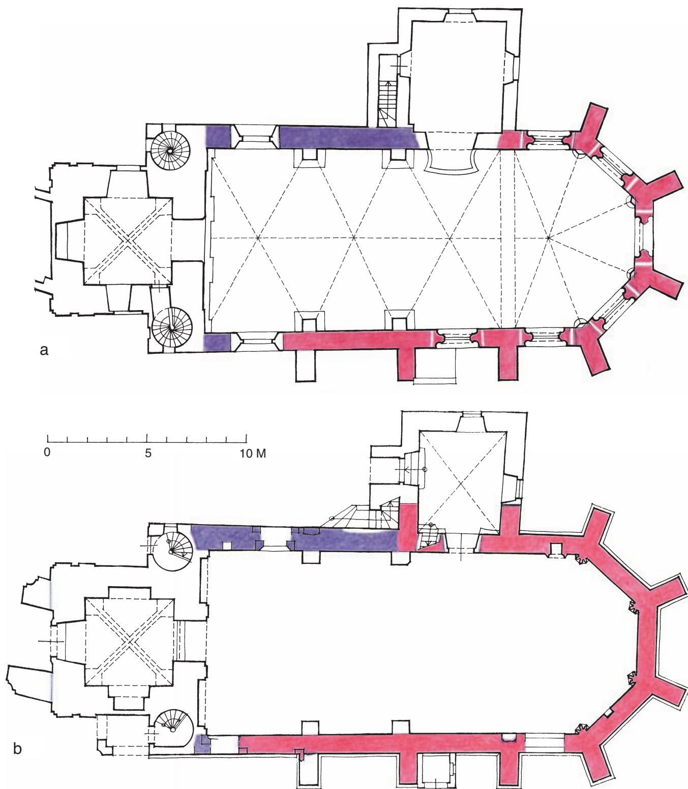
Obr. 6: Benátky nad Jizerou, kostel Narození Panny Marie v areálu zámku, a – půdorys v úrovni oken, b – půdorys v úrovni vstupů s vyznačením gotických stavebních fází a náleзовých situací. Červeně označeno gotické zdivo kolem roku 1350, fialově pozdně gotické zdivo, bez barevného označení mladší etapy (vyhodnocení stavebního vývoje se zaměřením náleзовých situací E. Vyletová, 2012, s využitím zaměření půdorysu Ing. Blabolá z roku 1976).
