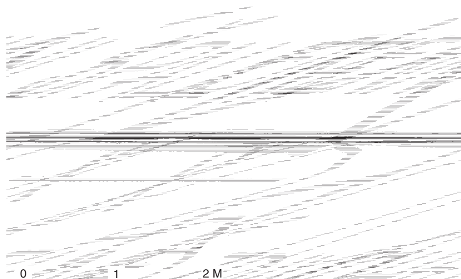
Obr. 29: Benátky nad Jizerou, kostel Narození Panny Marie, západní pole jižního průčelí s nálezy po odstranění omítek (zaměření a kresba E. Vyletová, 2005).
