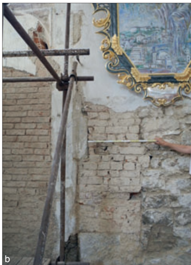
Obr. 13: Benátky nad Jizerou, kostel Narození Panny Marie: a – jižní stěna závěru s odkrytým výklenkem, pravděpodobně sedilí. Z původního gotického výklenku se zachovaly kvádry ostění. Kružba byla zřejmě při pozdější úpravě snesena níž, čemuž nasvědčují druhotně odsekané části horních kvádrů ostění pro její vložení. Výška původního výklenku by tak odpovídala výšce dochovaných výběhů původní podokenní římsy. K posunutí kružby mohlo dojít nejspíše v souvislosti se snížením parapetů oken závěru. V další fázi stavebních úprav byl vložen cihelný pas a došlo i k odsekání profilace ostění pod pasem. Při poslední úpravě byl výklenek ze strany interiéru zaslepen cihelnou zazdívkou o tloušťce 15 cm. Při současné obnově interiéru byla cihelná zazdívka odstraněna. Foto zachycuje stav v průběhu prací; b – Cihelná plenta o šířce 60 cm vpravo od ostění výklenku v místě předpokládané přípoje, která byla zřejmě odstraněna v souvislosti s vložení renesanční klenby.
