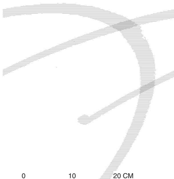
Obr. 24: Benátky nad Jizerou, kostel Narození Panny Marie, profilace záděných portálů západního pole interiéru: a – profilace sondážně odkryté části ostění v západním nároží jižní stěny; b – profilace pravoúhlého portálu západního pole severní stěny (zaměření a kresba E. Vyletová, 2012).
