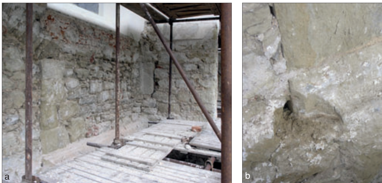
Obr. 28: Benátky nad Jizerou, kostel Narození Panny Marie: a – západní pole jižního průčelí s fragmentem profilovaného článku pod mladší přístěvkou pílře. Vlevo ostění původního vstupu; b – detail pískovcové římsy soklu zalamující se podél ostění (stav po odstranění omítek 2005)
