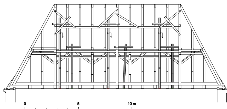
Obr. 8: Jedlka, kostel sv. Anny, podélný řez krovem nad lodí s pohledem k severu. Světle šedou jsou zvýrazněna jednoduchá a tmavší šedou dvojitá věšadla (zaměření a kresba J. Skopec 2011).
