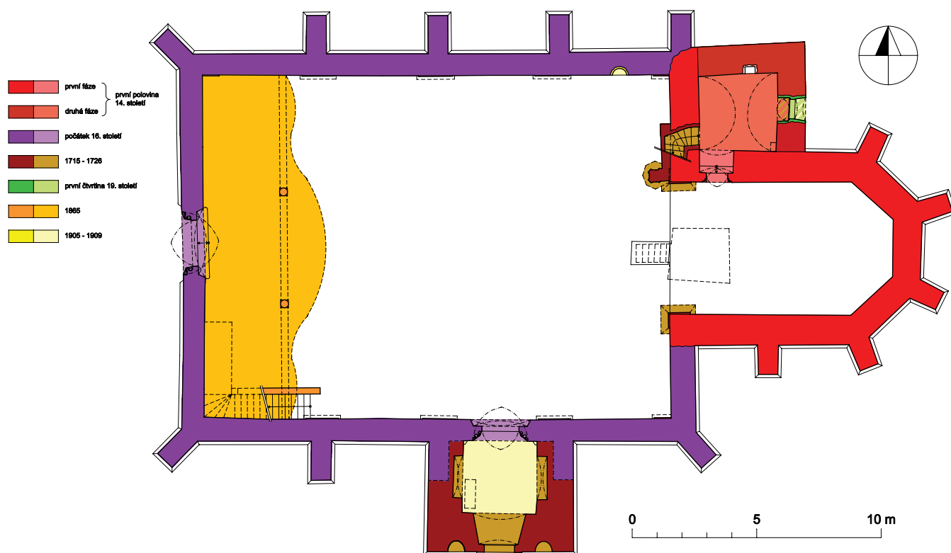
Obr. 4: Jedlka, kostel sv. Anny, půdorys v úrovni vstupů s vyhodnocením stavebního vývoje (zaměření J. Skopec a V. Zeman, kresba a vyhodnocení J. Skopec 2012. Zaměření krypty bylo převzato z Antonín Majer – Martin Strejc, Malá Veleň – Jedlka. Kostel sv. Anny. Nedestrukční vyhledání a zaměření krypty, Západočeský institut pro ochranu a dokumentaci památek, Plzeň 2010).
