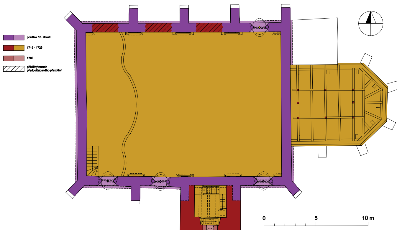
Obr. 6: Jedlka, kostel sv. Anny, půdorys v úrovni horní etáže prvního patra věže s vyhodnocením stavebního vývoje (zaměření J. Skopec a V. Zeman, kresba a vyhodnocení J. Skopec 2012).
