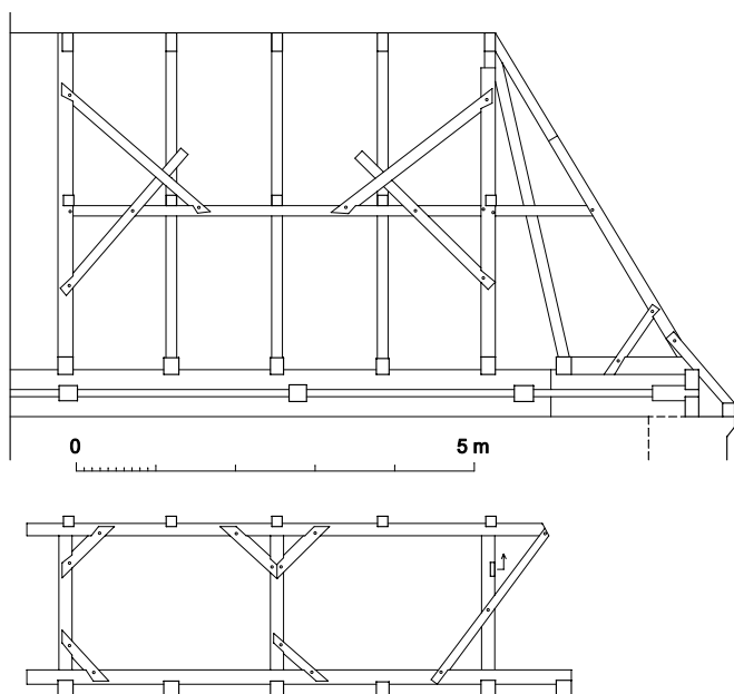
Obr. 10: Jedlka, kostel sv. Anny, krov nad presbytářem. A – podélný řez s pohledem k severu, B – severní podélná stolice v pohledu od jihu (zaměření a kresba J. Skopec 2011).
