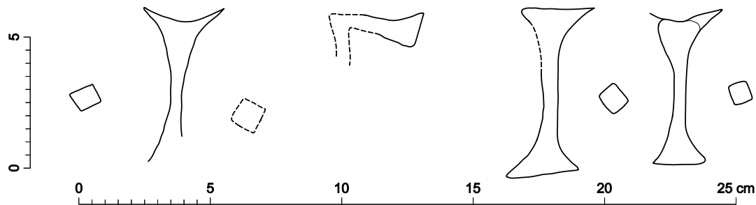
Obr. 30: Jedlka, kostel sv. Anny, nárys čelního pohledu fragmentu letopočtu 1511 na nejvrchnějším kvádru jihojihozápadního opěrného pilíře lodi. Čárkovaná čára značí již velmi slabě znatelné linie. Letopočet byl pauzován na průhlednou fólii (zaměření a kresba J. Skopec, 2009).
