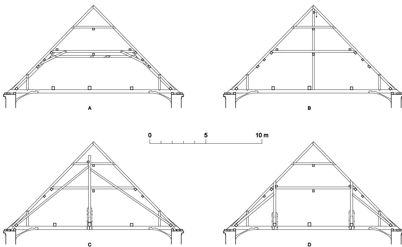
Obr. 9: Jedlka, kostel sv. Anny, krov nad lodí. A – druhá plná příčná vazba od západu s pohledem k východu, B – osmá mezilehlá příčná vazba od západu s pohledem k východu, C – příčný řez na úrovni třetího jednoduchého věšadla od západu, D – příčný řez na úrovni třetího dvojitého věšadla od západu (zaměření a kresba J. Skopec, 2011).
