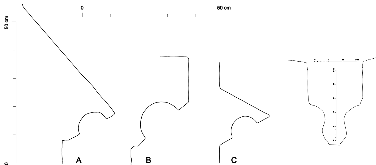
Obr. 13: Jedlka, kostel sv. Anny, profily říms. A – profil římsy odsazení opěrných pilířů lodi, B – profil korunní římsy lodi, C – profil podokenní římsy lodi. Zaměření říms B a C bylo provedeno pomocí obrysové šablony s posuvnými jehlami, římsa A byla pauzována na průhlednou fólii (zaměření a kresba J. Skopec, 2012).
