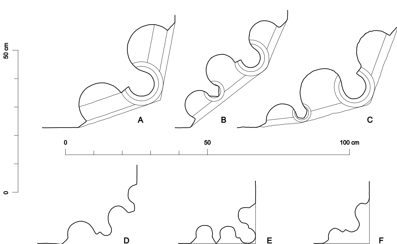
Obr. 12: Profily portálových ostění. A – profil severní stojky západního portálu lodi kostela sv. Anny v Jedlce, B – profil západní stojky jižního portálu lodi kostela sv. Anny v Jedlce, C – profil západní stojky jižního portálu lodi kostela Narození Panny Marie v Benešově nad Ploučnicí, D – profil západní části archivolty třetího jižního portálu od západu Horního zámku v Benešově nad Ploučnicí, E – profil severní stojky portálu dvoulodní místnosti v druhém patře severního křídla františkánského kláštera v Kadani, F – profil západní stojky portálu z presbytáře do sakristie kostela sv. Anny v Jedlce. Zaměření bylo provedeno pomocí obrysové šablony s posuvnými jehlami (zaměření a kresba J. Skopec, 2012).
