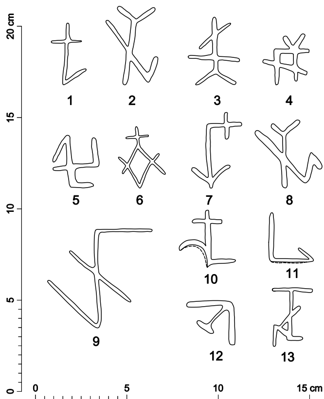
Obr. 29: Jedlka, kostel sv. Anny, nárysy čelních pohledů kamenických značek s číselným indexem označující typ uváděný v textu. Značky byly pauzovány na průhlednou fólii (zaměření a kresba J. Skopec, 2009).
