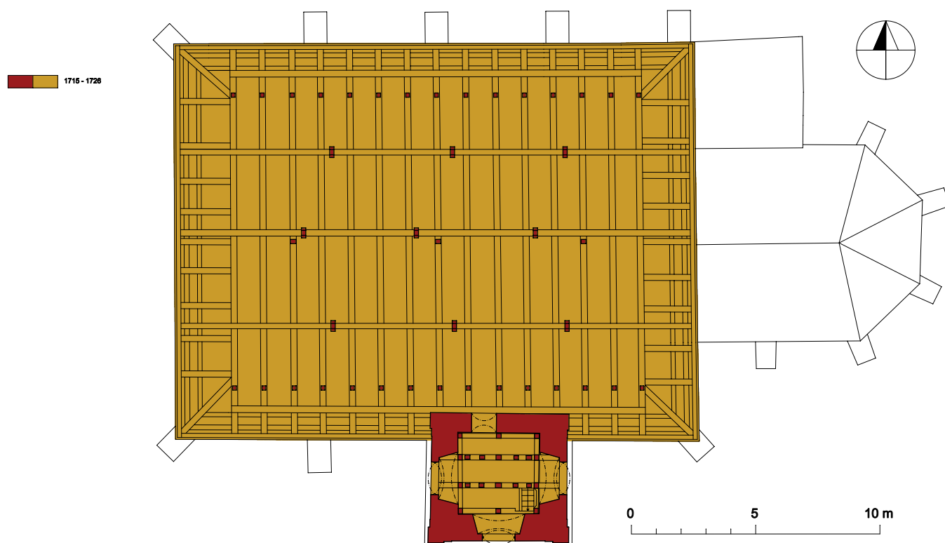
Obr. 7: Jedlka, kostel sv. Anny, půdorys v úrovni druhého patra věže s vyhodnocením stavebního vývoje (zaměření J. Skopec a V. Zeman, kresba a vyhodnocení J. Skopec 2012).
