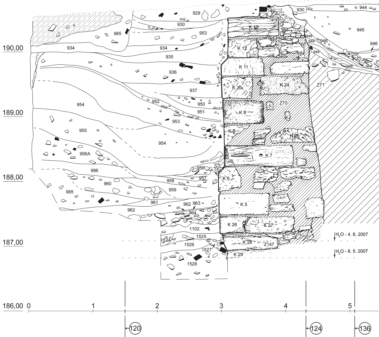
Obr. 5: Praha-Malá Strana, dvůr mezi čp. 28 a 33/III. Severovýchodní stěna nárožního opěráku na JZ rohu východního traktu na výřezu archeologického profilu č. 123. Vrstva 1102 je pochozí terén patrně raně renesanční (zaměření a kresba M. Müller, 2007).
