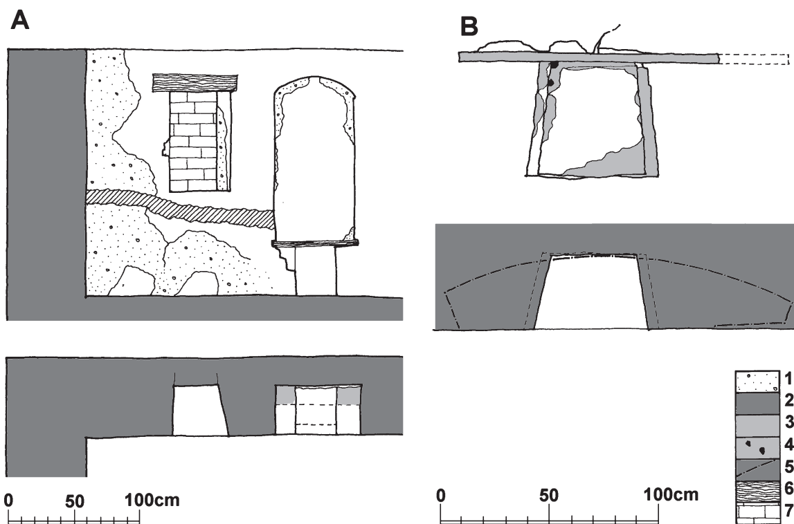
Obr. 18: Hrad Buchlov, A – zaměření záchodové niky a střelnového okénka na půdě, situovaných v jižní zdi východní věže; nahoře – čelní pohled od severu, dole – vodorovný řez, B – zaměření výklenku ve východní stěně sklepa; nahoře – čelní pohled od západu, dole – vodorovný řez horní částí niky s deskou překlada (čárkovaně vyznačen půdorys dna niky); 1 – „předpožárová“ omítka, 2 – zdivo v řezu, 3 – plochy malty s otisky dřevěných prvků, 4 – zbytky kovových prvků, 5 – obrys desky, využitý jako překlada nad nikou, 6 – dochované dřevěné prvky.
