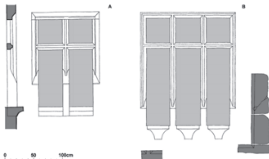
Obr. 8: Hrad Buchlov, A – zaměření okenního ostění arkýře v severovýchodní fasádě traktu; napravo čelní pohled, nalevo svislý řez; B – zaměření západního okna rytířského sálu, vnější pohled; tmavě šedou jsou vyznačeny plochy torza ostění staršího okenního otvoru. Mimo zaměření se nachází kamenná, barokní výlevka.
