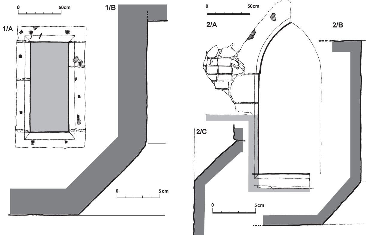
Obr. 15: Hrad Buchlov, 1 – zaměření okenního ostění v patře východní věže (západní zed); 1/A – čelní pohled od západu, 1/B – vodorovný profil levé stojky ostění, 2 – zaměření torza okenního ostění u severozápadního nároží traktu; 2/A – čelní pohled (šedě je vyznačen průběh přiložené, parapetní zidky balkonu), 2/B – vodorovný profil stojky, 2/C – svislý profil bankálu.
