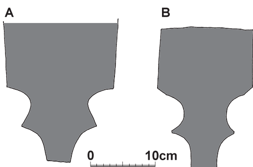
Obr. 24: Hrad Buchlov, zaměření profilu klenebních žeber; A – profil žebra v místnosti č. 21, B – profil cihelné tvarovky, uložené v hradním lapidáriu.
