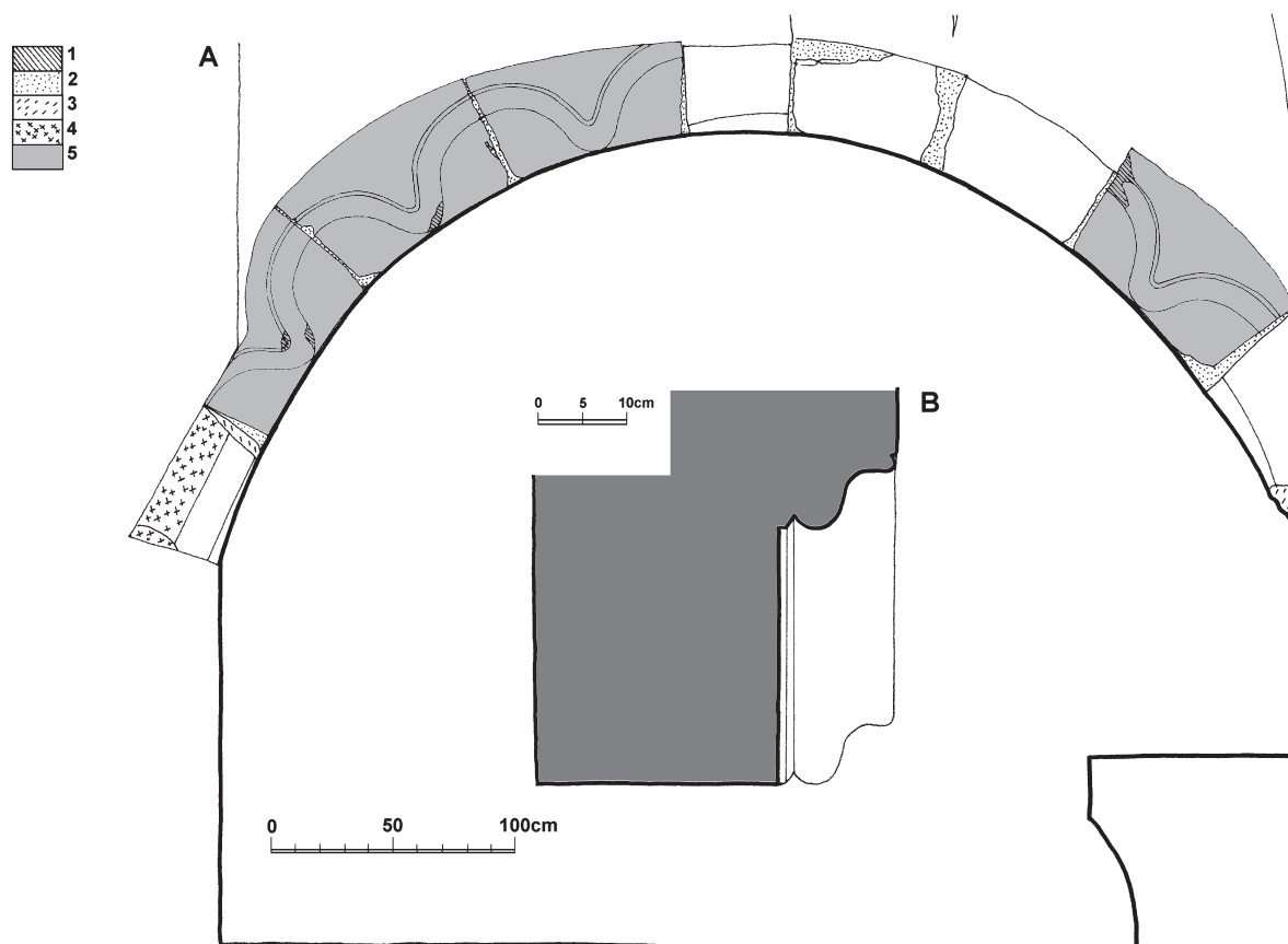
Obr. 23: Hrad Buchlov, zaměření pasu v místnosti č. 17; A – pohled od severu, 1 – poškozený povrch kamene, 2 – malta, 3 – druhotné opracování, jemnější, 4 – druhotné opracování, hrubé, 5 – pozdněrománské bloky, B – svislý profil styčné (boční) plochy pozdněrománského bloku.
