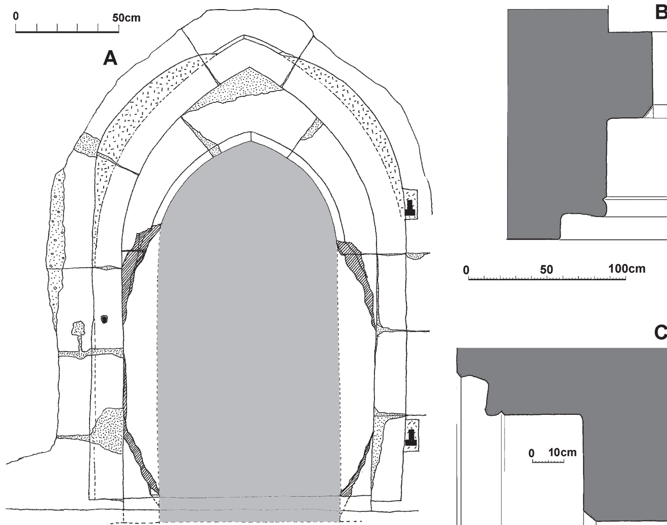
Obr. 19: Hrad Buchlov, A – zaměření portálu vstupu do místnosti č. 11, pohled od západu; tečkované – malty, šrafované – povrch se stopami odlámání, čárkované – plochy přesekané pro použití vrat, B – vodorovný profil levé stojky, C – svislý profil ostění ve vrcholu záklenku.
