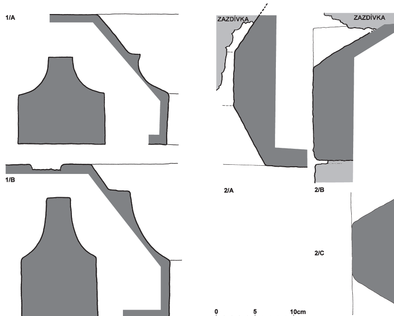
Obr. 9: Hrad Buchlov, 1 – profilace stojek a svislých, dělicích prutů pozdně gotických oken vnější fasády severního traktu; 1/A – arkýř v severovýchodní fasádě, 1/B – východní okno rytířského sálu; 2 – zaměření profilace fragmentů okenního ostění u západního okna rytířského sálu; 2/A – vodorovný profil okenní stojky, 2/B – svislý profil bankálového prvku s náběhem dělicího prvku, 2/C – pohled shora na přístupnou část bankálového prvku – šedá plocha označuje profil náběhu svislého, dělicího prvku.
