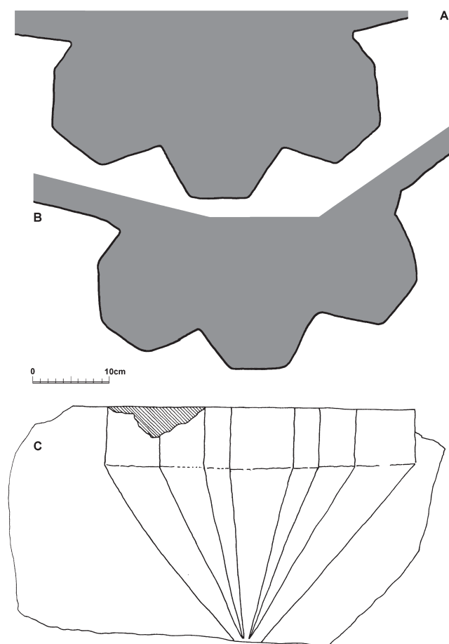
Obr. 36: Hrad Buchlov, zaměření dvojice klenebních konzol, uložených v hradním lapidáriu; A, B – zaměření horních hran prvků, dole – čelní pohled na konzolu A.
