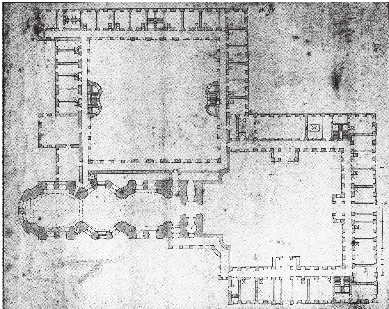
Obr. 2: Jan Blažej Santini-Aichel, návrh novostavby rajhradského kláštera, definitivní verze projektu, půdorys přzemí celého kláštera, asi 1721 (Staatsbibliothek Bamberg, Bestandsgruppe Msc. Add., sign. Msc. Add 38)
