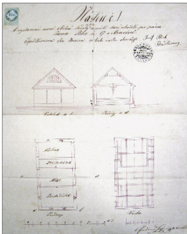
Obr. 7: Mravín, nedatovaný plán k vystavění nové obilní stodoly na místě staré shoelé pro pana Jana Pelce, čp. 17 v Mravíně, navržený Ferdinandem Boh... mistrem stavitelským. Projekt navrhoval obdélnou stodolu v typické čtyřdílné dispozici s průjezdným mlatem, dvěma perami a připojenou kolnou. Stodola byla postavena po požáru usedlosti v roce 1864 a ve dvacátých letech dvacátého století zvětšena a přestavěna (SOKa Chrudim, AO Mravín, inv.č. 25, kart.č. 2).
