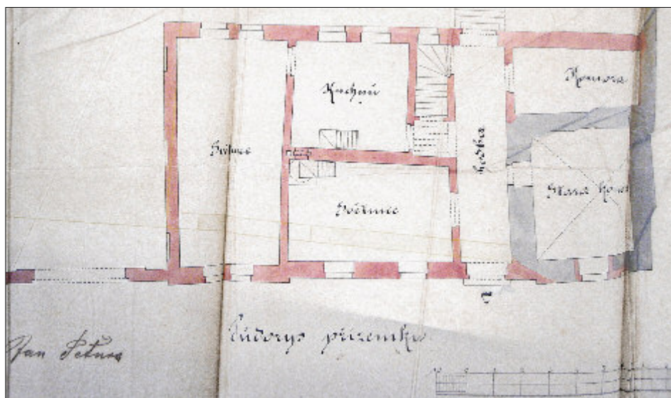
Obr. 14: Mravín, čp. 2, stavební plán výstavby nového okapově orientovaného domu směrem k návsi s využitím komory ze staršího štítově orientovaného domu, vypracováno vysokomýtským stavitelem Josefem Drahošem v roce 1884 (SOKA Chrudim, inv.č. 25, kart.č. 2).
