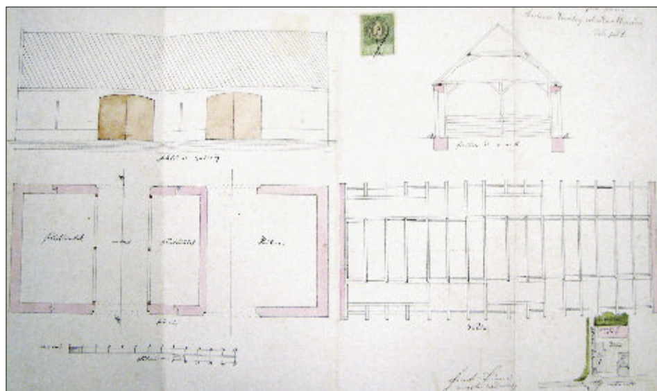
Obr. 8: Mravín, plán na výstavbu nové stodoly pro Antonína Novotného z Mravína čp. 1. Projekt stavby, který byl schválen v roce 1881, navrhl Franc Tůma, mistr zednický. Jednalo se o příčně průjezdnou stodolu se středním mlatem, dvěma přístodůlky a napojeným příjezdem s kolnou. Stavba byla zděná z opuky s vyzděnými šterbinovými větracími průduchy, krov řešen Rankovou konstrukcí a střecha byla kryta břidlicí. Stodola byla odstraněna v 1982 (SOKa Chrudim, AO Mravín, inv.č. 25, kart. 2).
