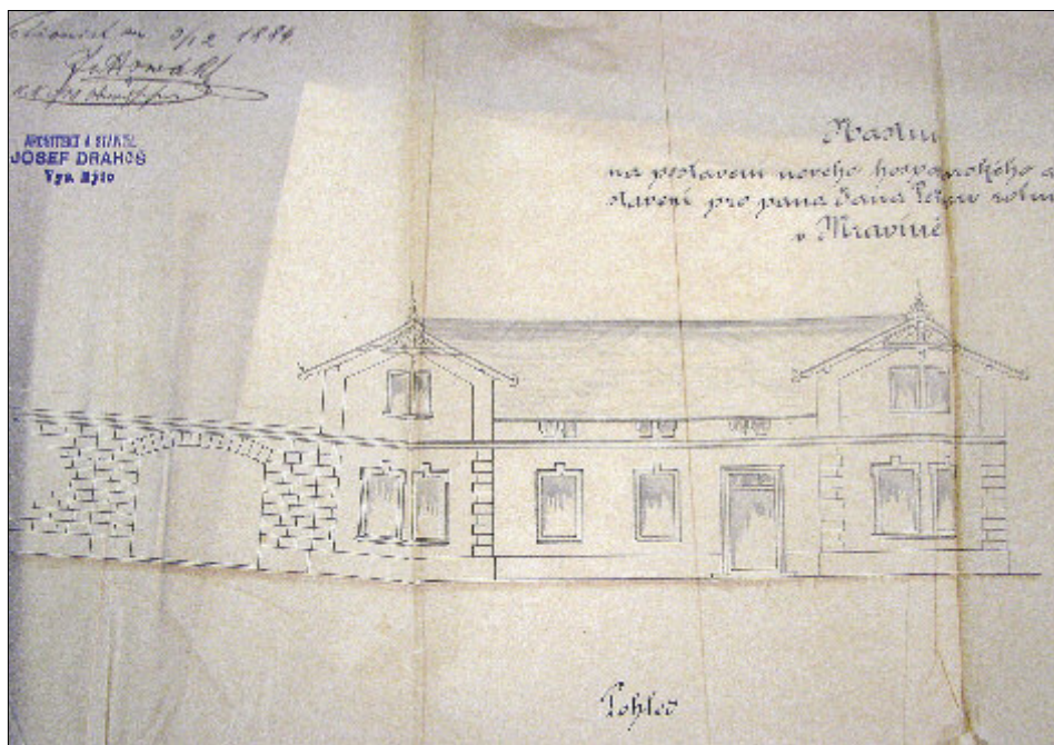
Obr. 10: Mravín, stavební plán průčelí domu v usedlosti čp. 2 pro Jana Petiuru, vypracovaný vysokomýtským stavitelem Josefem Drahošem v roce 1884. Projekt zachycuje návrh vzhledu průčelí domu v tehdejší moderním duchu historismu, které pravděpodobně nebylo v této podobě realizováno (SOKA Chrudim, inv. č. 25, kart. č. 2).
