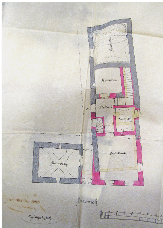
Obr. 9: Mravín, stavební plán přestavby světnice a kuchyňské části pro Jana Svatoše majitele domu čp. 19 v Mravíně, vypracovaný vysokomýtským stavitelem Josefe Drahošem v roce 1885. Projekt zachycuje odstranění staré světnice a kuchyňské niky s dymníkem v zadní části síně a navrhuje prodloužení světnice a výstavbu nové kuchyně s tahovým komínem uzavřené segmentovou klenbou (SOKA Chrudim, inv.č. 25, kart. č. 2).
