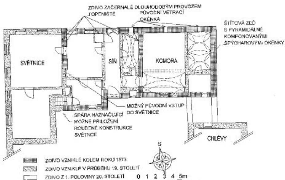
Obr. 22: Děkanské Skaliny, čp. 13 – půdorys obytné části usedlosti (podle zaměření J. Drozdy).
