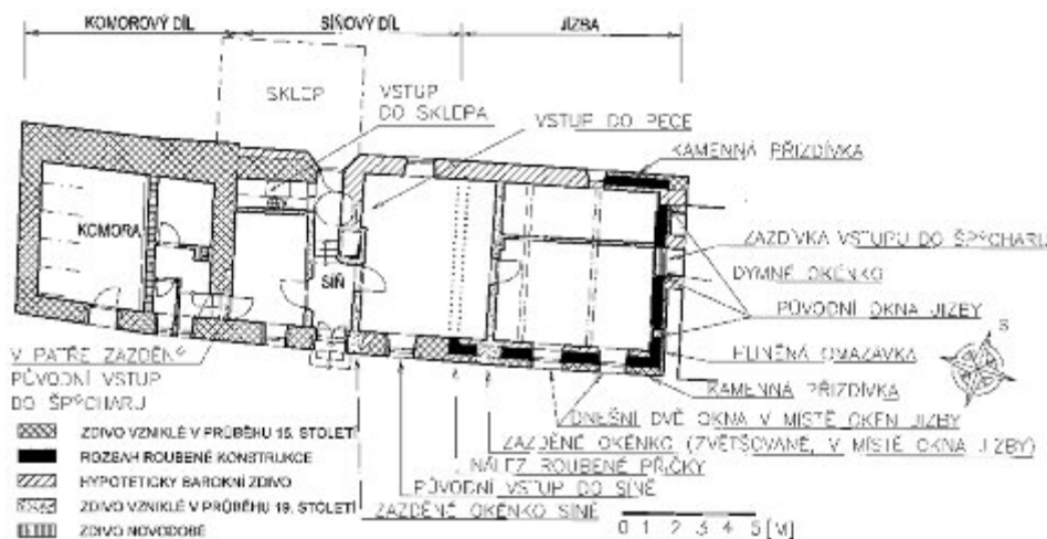
Obr. 2: Mirkovice, čp. 1 – půdorys obytné části usedlosti (podle zaměření M. Špinarové).
