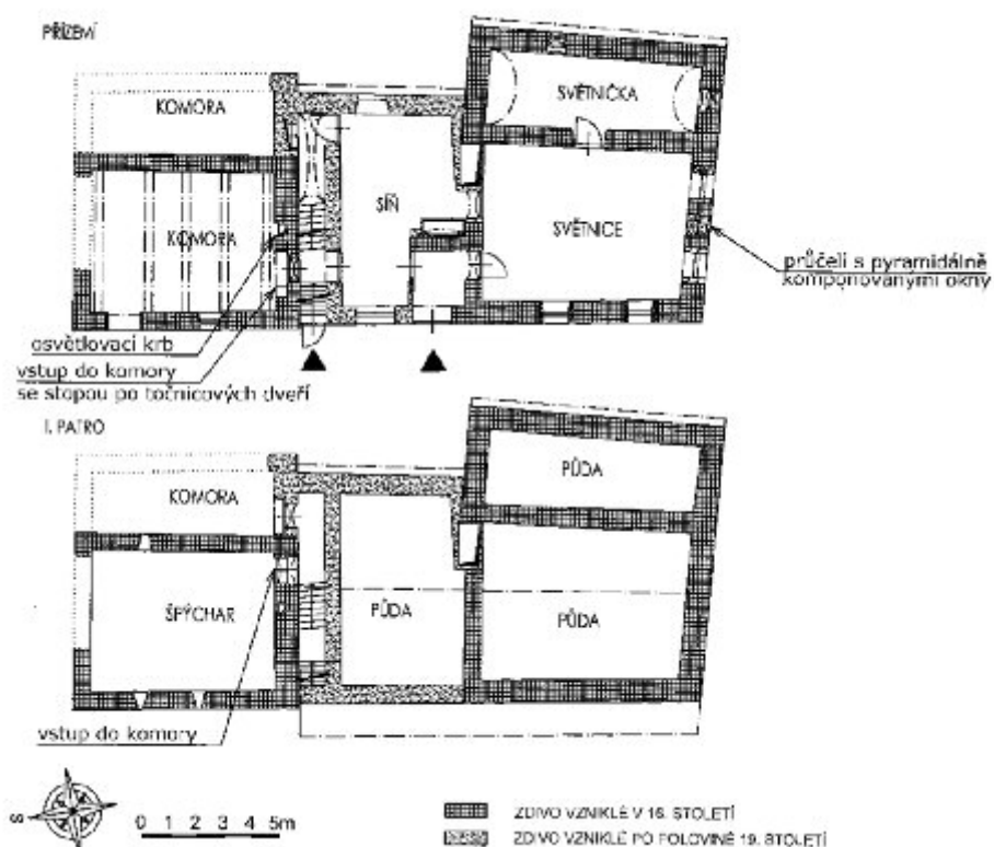
Obr. 11: Záluží, čp. 6 – půdorys obytné části usedlosti (zaměření autor).
