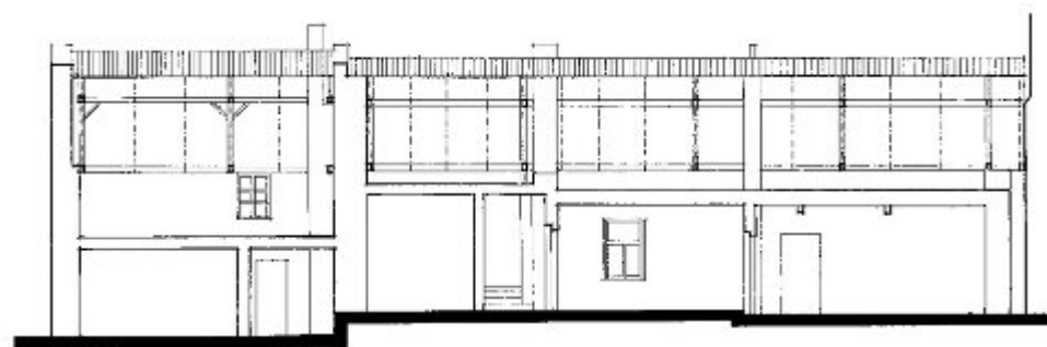
PODELNÝ ŘEZ B-B' MIRKOVICE ČP. 1 (OBYTNÁ ČÁST)
