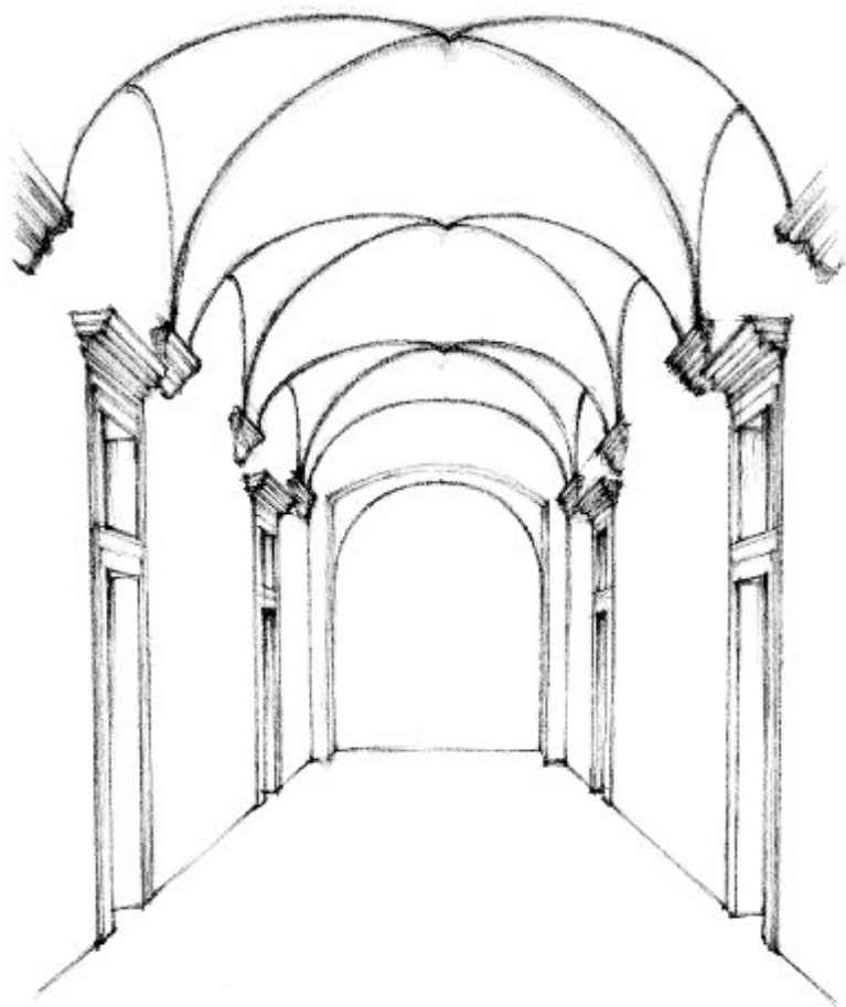
Obr. 22: Brandýs nad Labem, dům čp. 98. Rekonstrukce renesančního průjezdu, perspektivní skica s pohledem k náměstí (kresba E. Výletová, 2013).
