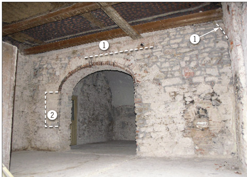
Obr. 13: Brandýs nad Labem, dům čp. 98 – přízemí, východní trakt, přední místnost s pohledem do středu dispozice, 1 – odsekaná pata klenby; 2 – zazděný okenní otvor s poškozeným renesančním ostěním, stav 2005.
