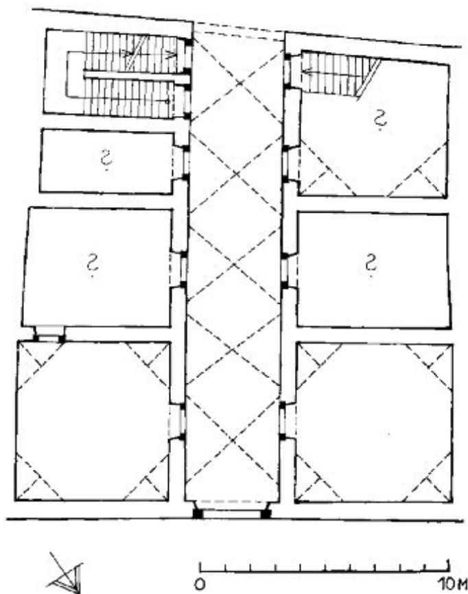
Obr. 20: Brandýs nad Labem, dům čp. 98. Schéma půdorysu přízemí s rekonstrukcí renesančního stavu (kresba E. Vyletová, 2013).
