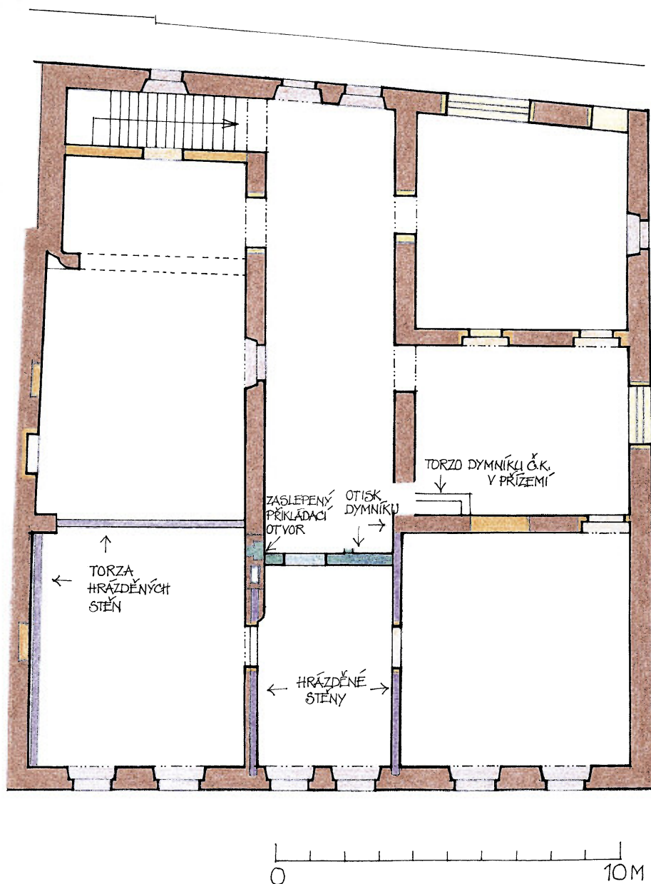
Obr. 9c: Brandýs nad Labem, dům čp. 98, půdorys patra s vyznačením stavebního vývoje (vyhodnocení stavebního vývoje a kresba E. Vyletová, 2013, s využitím zaměření MURUS, 2013).
