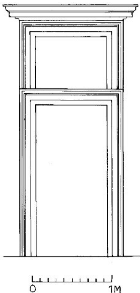
Obr. 21: Brandýs nad Labem, dům čp. 98. Rekonstrukce renesančních portálů v průjezdu (zaměření a kresba E. Výletová, 2013).
