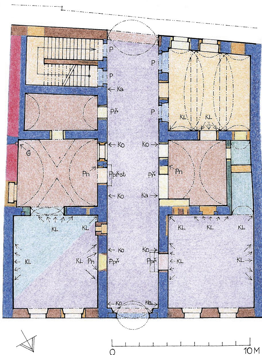
Obr. 9b: Brandýs nad Labem, dům čp. 98, půdorys přízemí s vyznačením stavebního vývoje (vyhodnocení stavebního vývoje a kresba E. Vyletová, 2013, s využitím zaměření MURUS, 2013).
