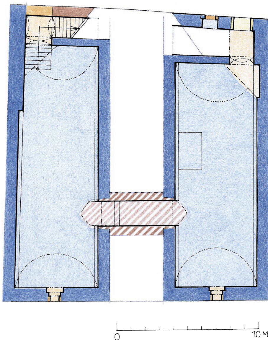
Obr. 9a: Brandýs nad Labem, dům čp. 98, půdorys sklepů s vyznačením stavebního vývoje (vyhodnocení stavebního vývoje a kresba E. Vyletová, 2013, s využitím zaměření MURUS, 2013).
