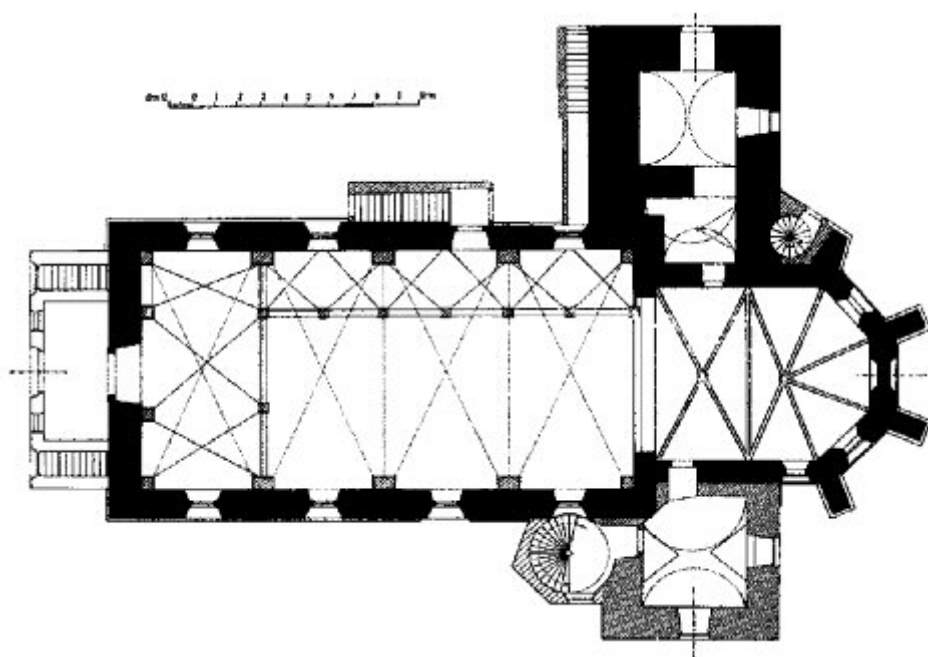
Obr. 2: Náchod, kostel sv. Vavřince – půdorys s vyhodnocením stavebního vývoje (podle Z. Wirtha 1910).
