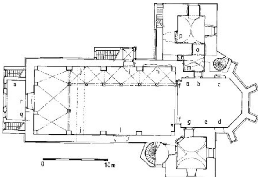
Obr. 3: Náchod, kostel sv. Vavřince – půdorys s vyznačením nálezů a stavebního vývoje: a – půlkruhový výklenek; b – portál severní sakristie; c – sanktuárium; d – zazděný průchod; e – epitaf Smiřických; f – soklový profil vítězného oblouku, na severní straně výklenek; g – portál jižní sakristie; h – přezdívková líce východního pole v severní stěně; i – severní portál; j – přízdívky v místě předpokládaného konce původní stavby; k – ryté kvádrování na jižní straně vítězného oblouku; l – zazděný jižní vstup; m – odsekaný sokl v severní sakristii; n – zazdívková mezera mezi věží a severní stěnou lodi; o – dodatečně prolomený průchod přízemím věže; p – zazděný původní vstup do přízemí věže; q – zazděný starší vstup na kůr; r – alabastrová erbovní deska; s – kruhotně osazené náhrobníky.
